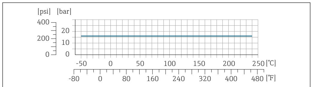
☑ 34 连接部件材质: 1.4404 (316/316L)
