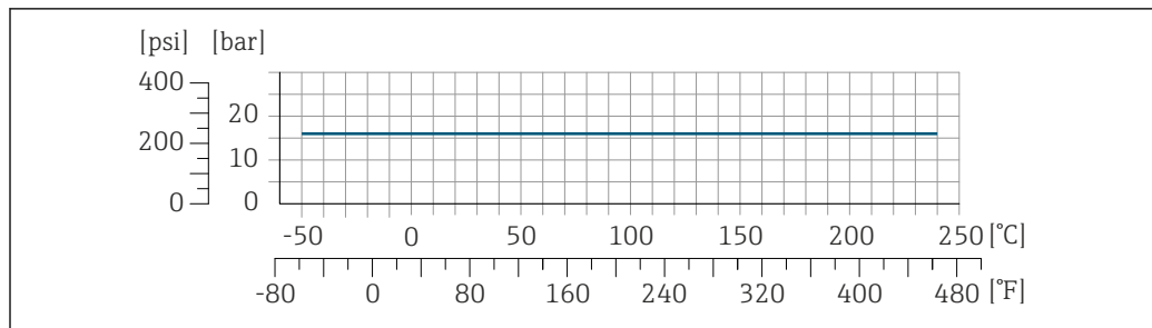
图 35 连接部件材质: 1.4404 (316/316L)
