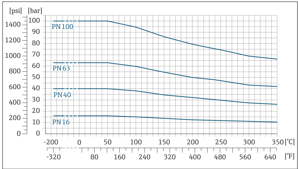
图 24 法兰材质: 1.4404 (F316/F316L)、Alloy C22 合金
