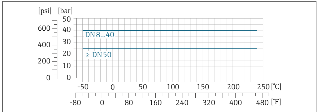
☑ 33 连接部件材质: 1.4404 (316/316L)
