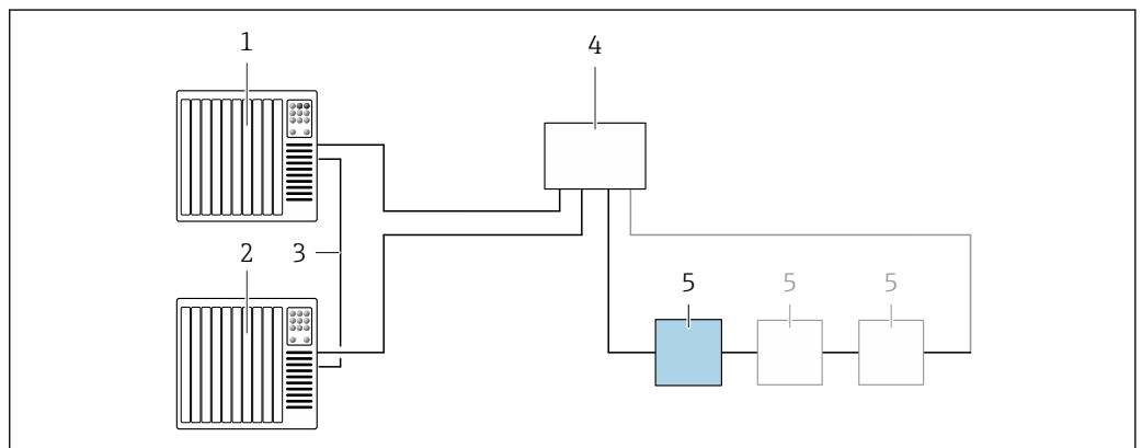
9 S2 系统冗余的连接示例
