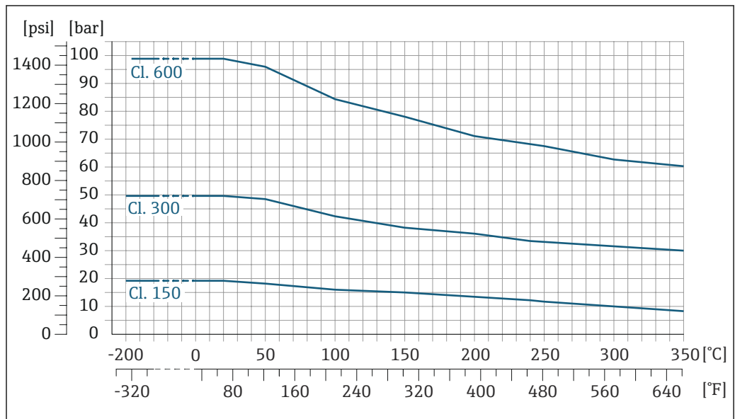
图 25 法兰材质: 1.4404 (F316/F316L)
