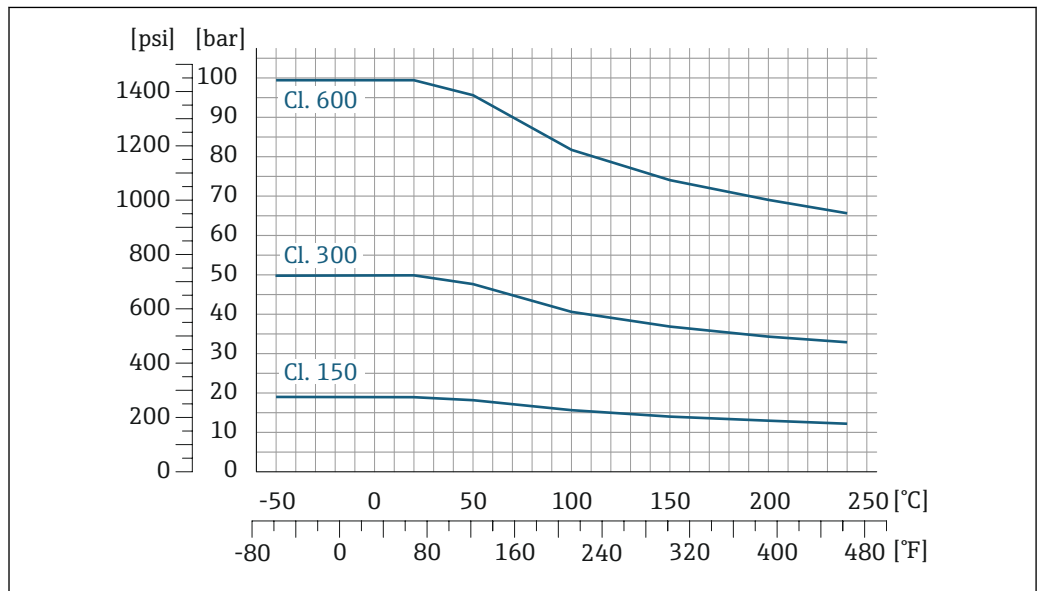
图 34 法兰材质: 1.4301 (F304) ; 接液部件材质: Alloy C22 合金
