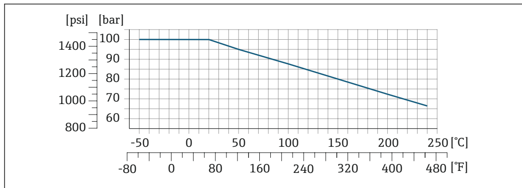
图 40 连接部件材质: 1.4404 (316/316L)
