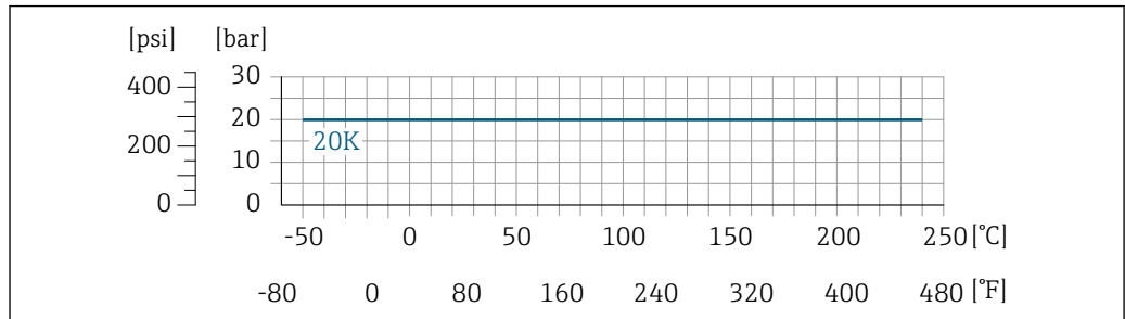
图 35 法兰材质: 1.4301 (F304) ; 接液部件材质: Alloy C22 合金
