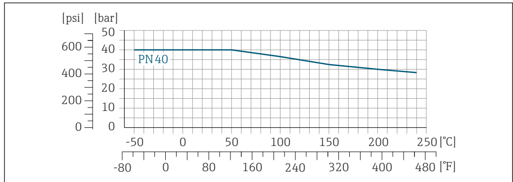
图 33 法兰材质: 1.4301 (F304) ; 接液部件材质: Alloy C22 合金
