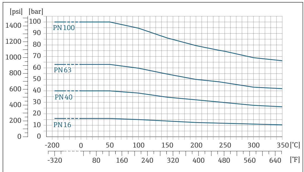
图 28 法兰材质: 1.4404 (F316/F316L)、Alloy C22 合金
