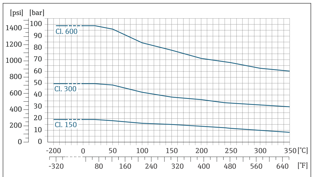
图 29 法兰材质: 1.4404 (F316/F316L)
