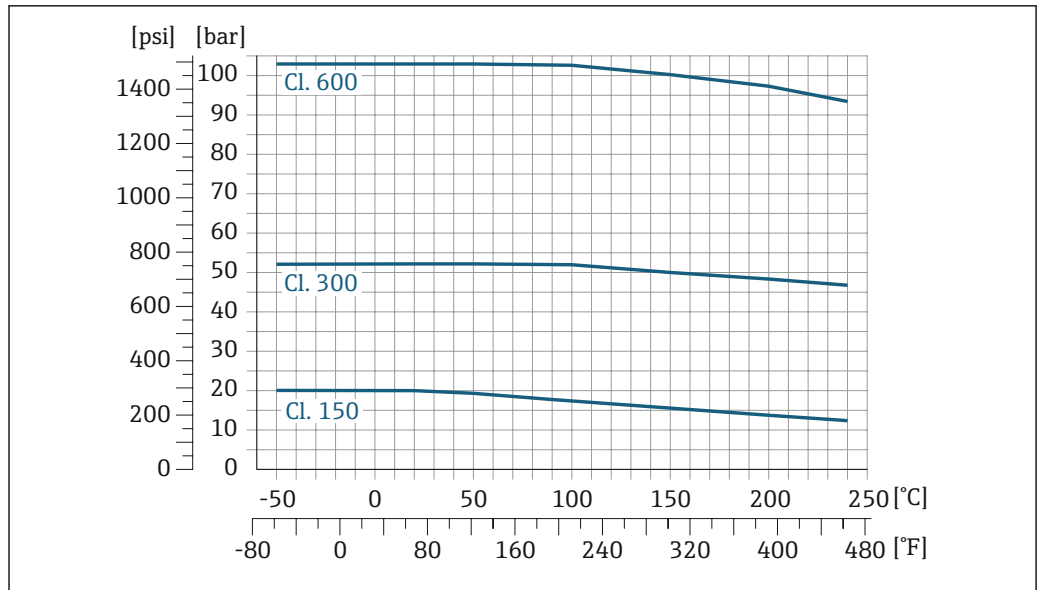
图 26 法兰材质: Alloy C22 合金
