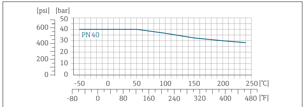
图 29 法兰材质: 1.4301 (F304) ; 接液部件材质: Alloy C22 合金
