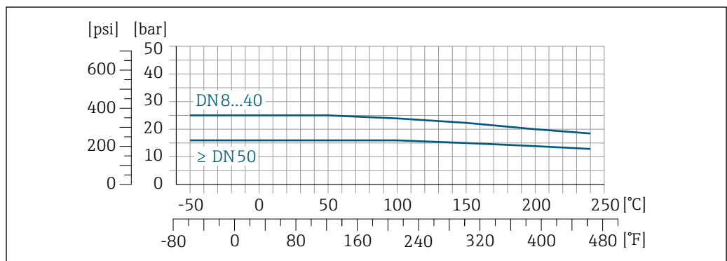
图 28 连接部件材质: 1.4404 (316/316L)
