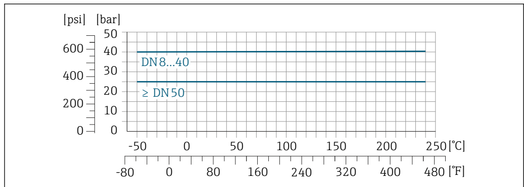
图 32 连接部件材质: 1.4404 (316/316L)
