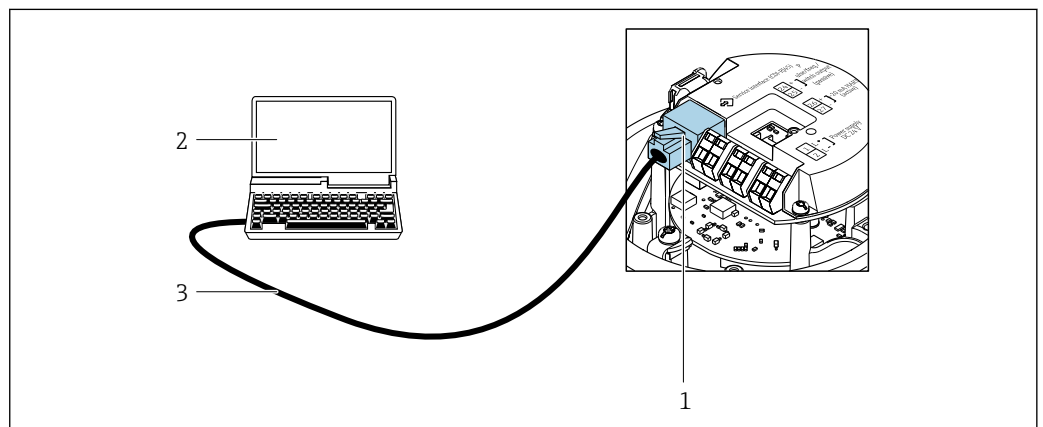
图 45 订购选项“输出”，选型代号 B：4...20 mA HART，脉冲/频率/开关量输出
