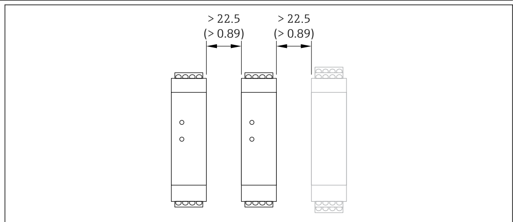
22 Promass 100 安全栅或其他模块的最小安装间距。单位: mm (in)
