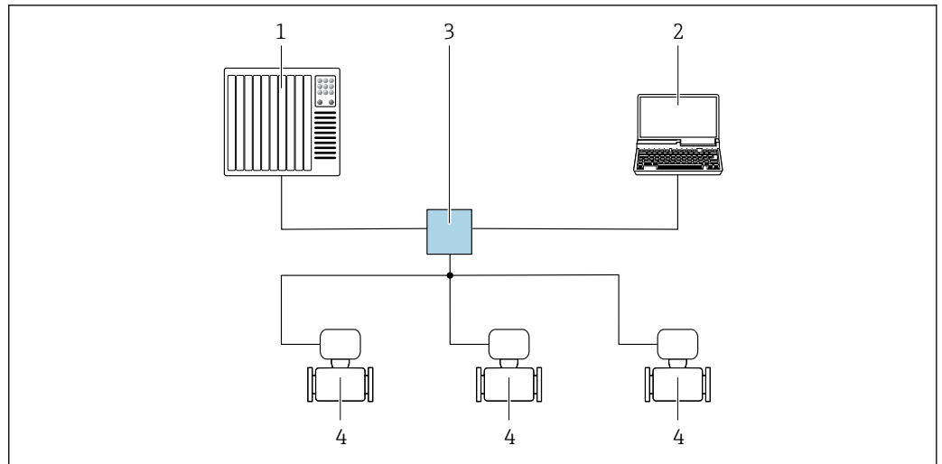
图 44 通过 PROFINET 网络实现远程操作：星形拓扑结构
