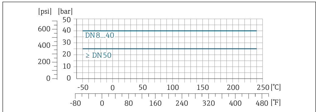
图 33 连接部件材质: 1.4404 (316/316L)
