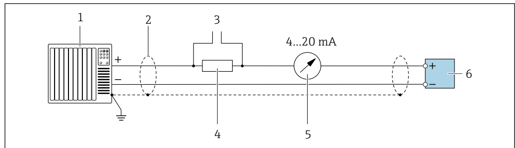
图 9 4...20 mA HART 电流输出（有源）的连接示例
