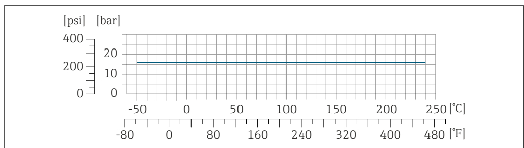
图 34 连接部件材质: 1.4404 (316/316L)
