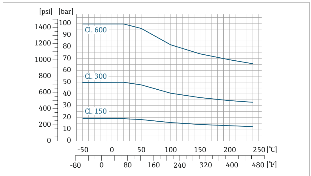
图 30 法兰材质: 1.4301 (F304) ; 接液部件材质: Alloy C22 合金
