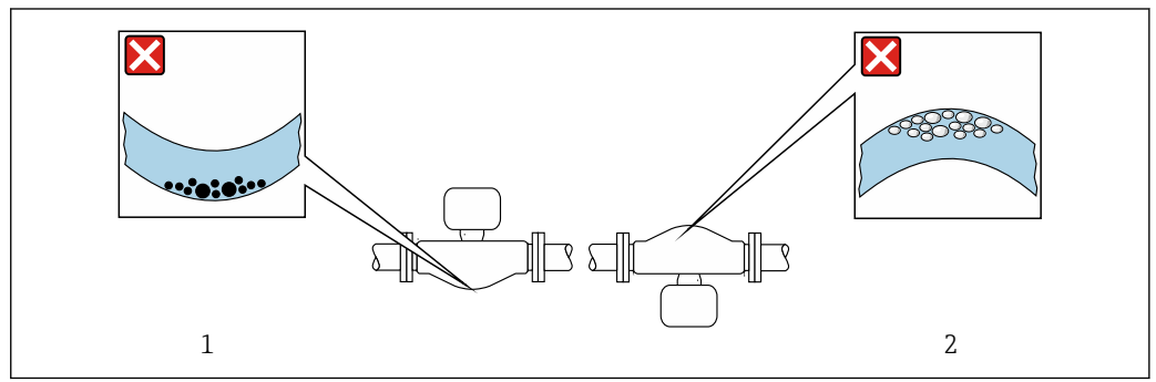
☒ 21 带弯测量管的传感器的安装方向
