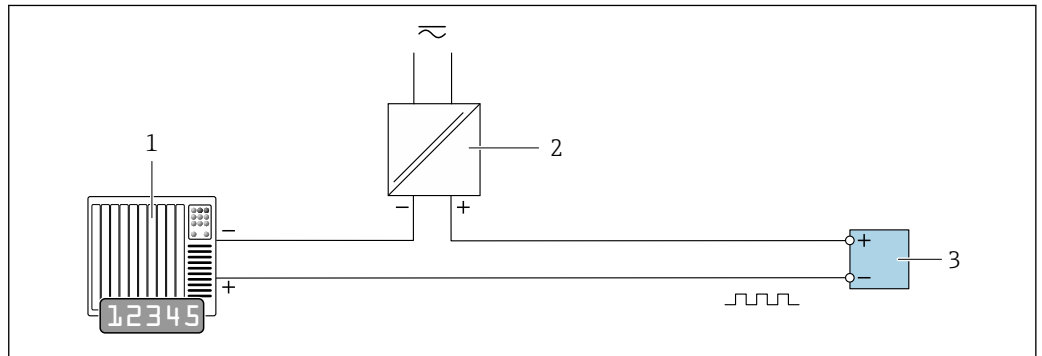
图 11 脉冲/频率输出（无源）的连接实例
