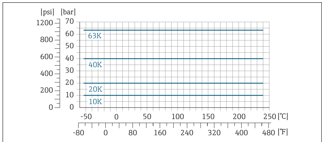
图 27 法兰材质: 1.4404 (F316/F316L)、Alloy C22 合金
