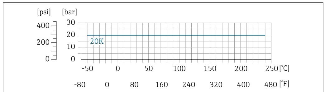
图 31 法兰材质: 1.4301 (F304) ; 接液部件材质: Alloy C22 合金
