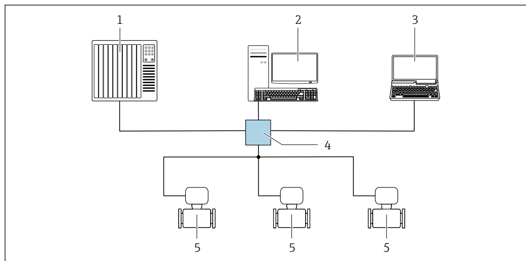
图 43 通过 EtherNet/IP 网络实现远程操作：星形拓扑结构
