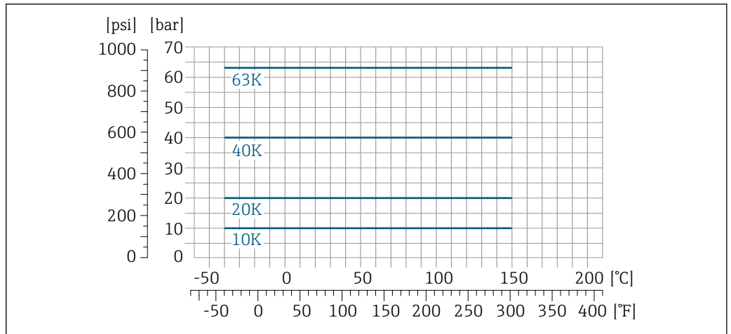
27 法兰材质: 1.4404 (F316/F316L)
