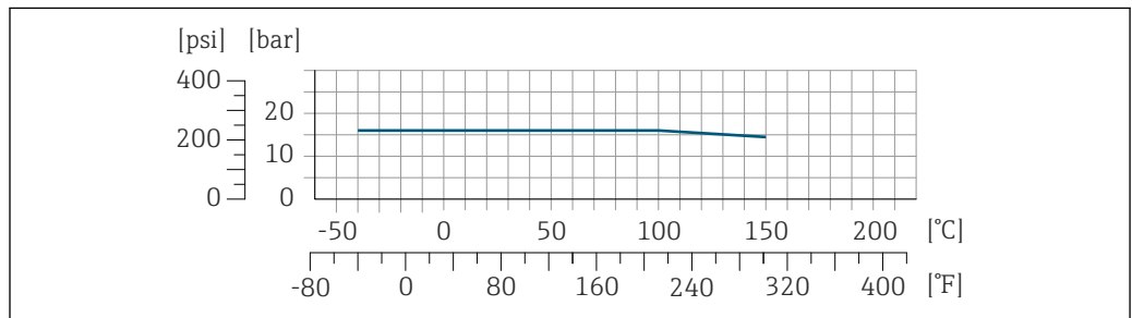
图 31 连接部件材质: 1.4404 (316/316L)
