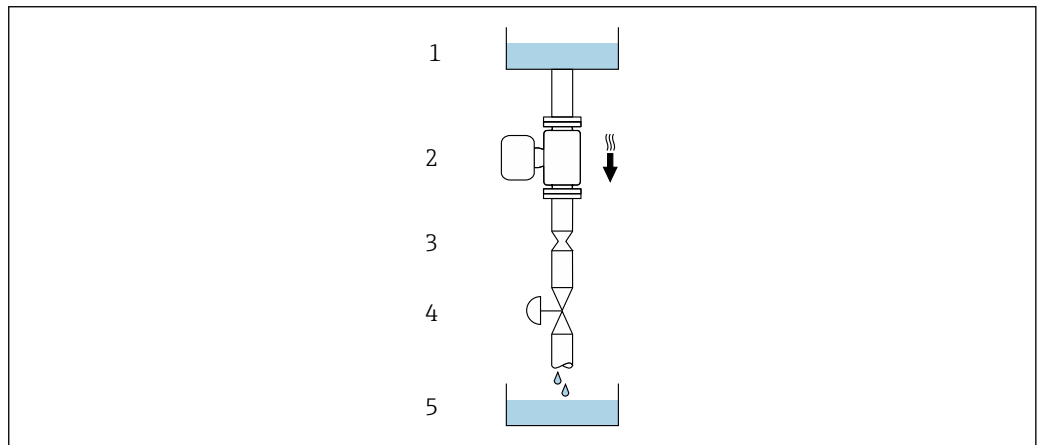
图 22 在竖直向下管道中安装（例如批处理应用）
