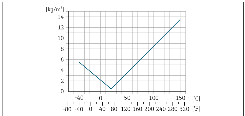
图 21 现场密度校准，例如在+20 °C (+68 °F)时
