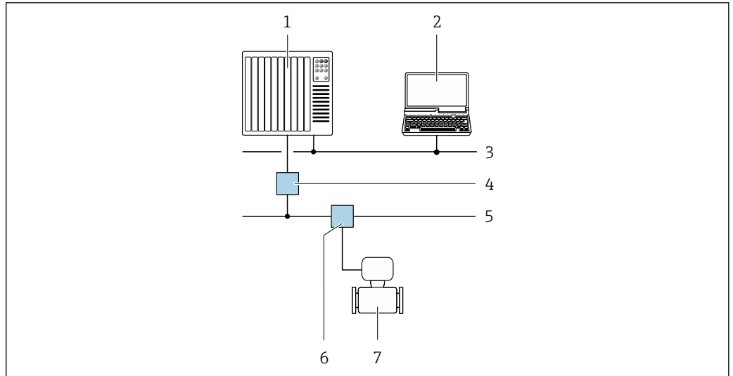
图 49 通过 PROFIBUS PA 网络进行远程操作
