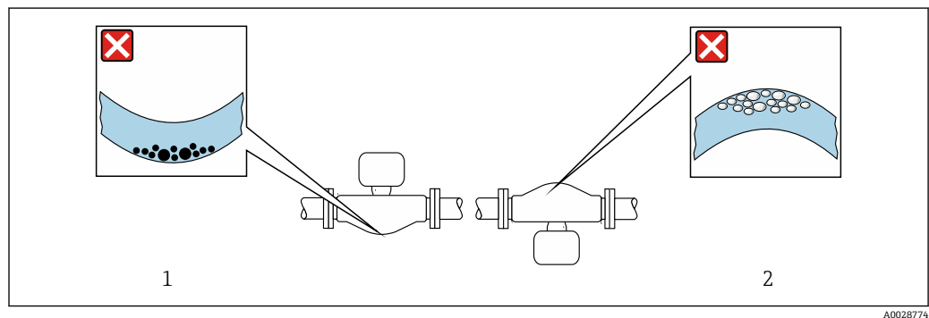
☑ 23 带弯测量管的传感器的安装方向
