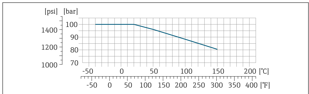
图 33 连接部件材质: 1.4404 (316/316L)
