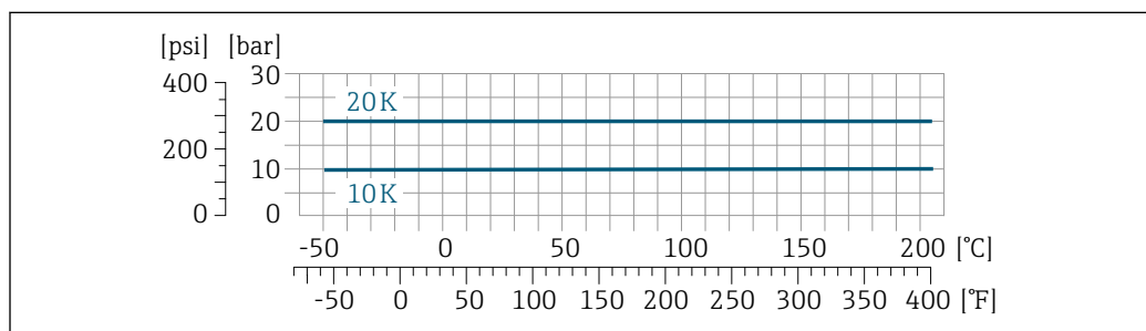
图 32 法兰材质: 1.4301 (304) ; 接液部件材质: 锆 702、钽
