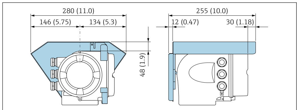
图 35 Proline 500 (模拟) 的防护罩
