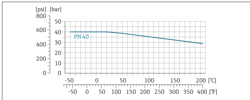
图 30 法兰材质: 1.4301 (304) ; 接液部件材质: 锆 702、钽
