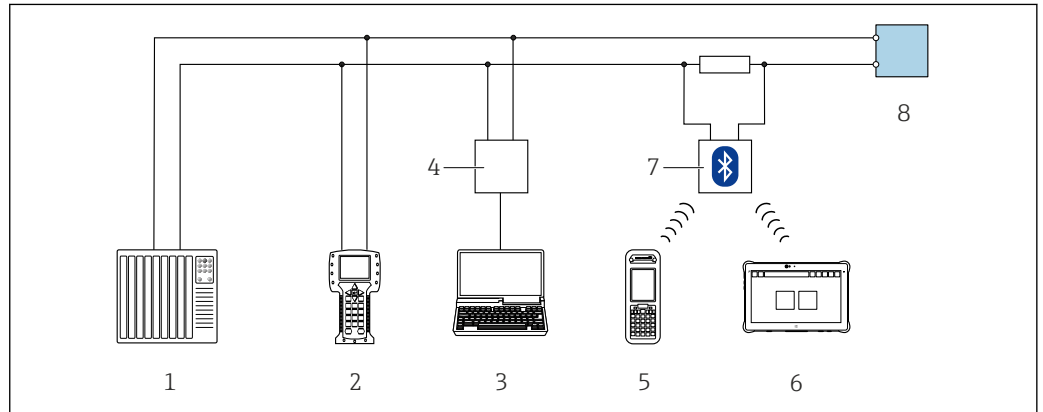
图 48 通过 HART 通信进行远程操作 (有源信号)
