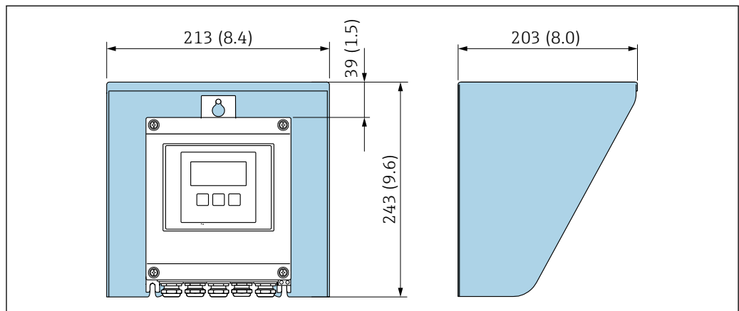
40 Proline 500 (数字) 的防护罩
