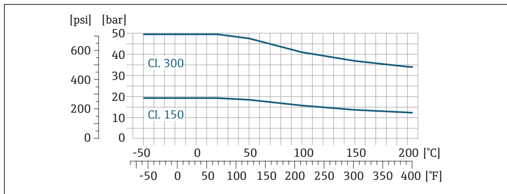
图 31 法兰材质: 1.4301 (304) ; 接液部件材质: 锆 702、钽
