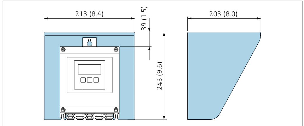
27 Proline 500 (数字) 的防护罩
