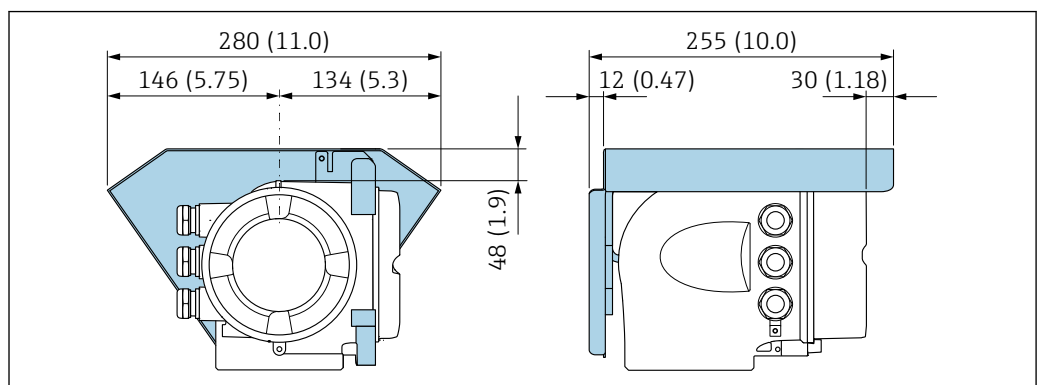
41 Proline 500 (模拟) 的防护罩
