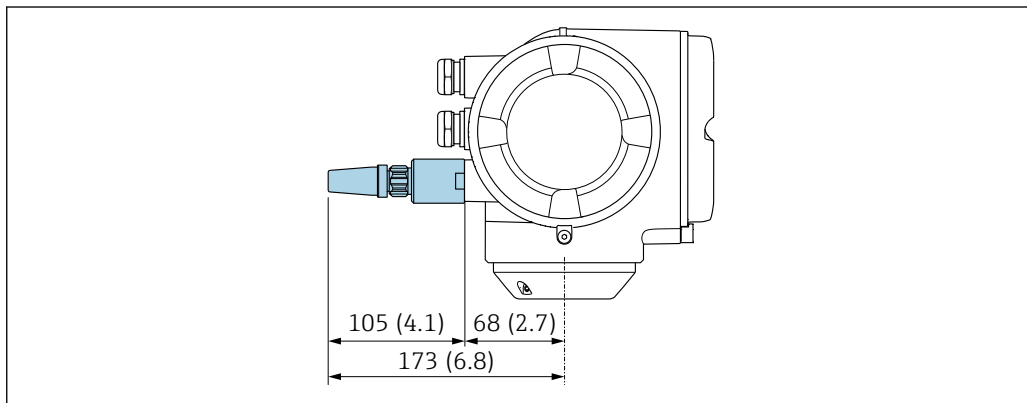
图 38 单位: mm (in)
