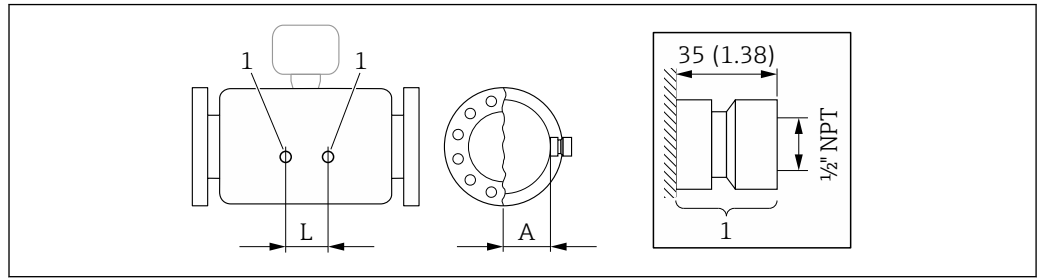
1 吹扫连接 (订购选项“传感器选项”, 选型代号 CH “吹扫连接”)
