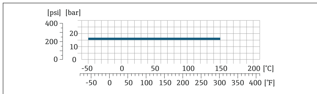
图 36 连接部件材质: 二级钛材
