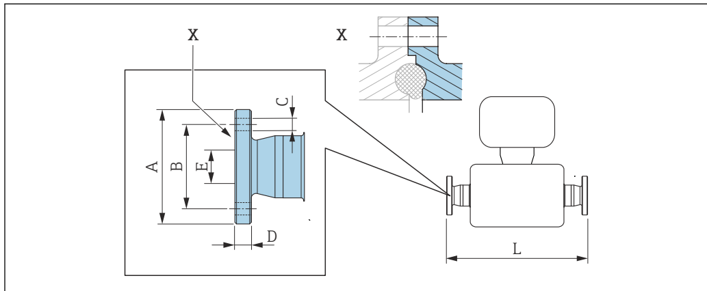
图 38 视图 X: 非对称过程连接; 灰色部分由供应商提供
