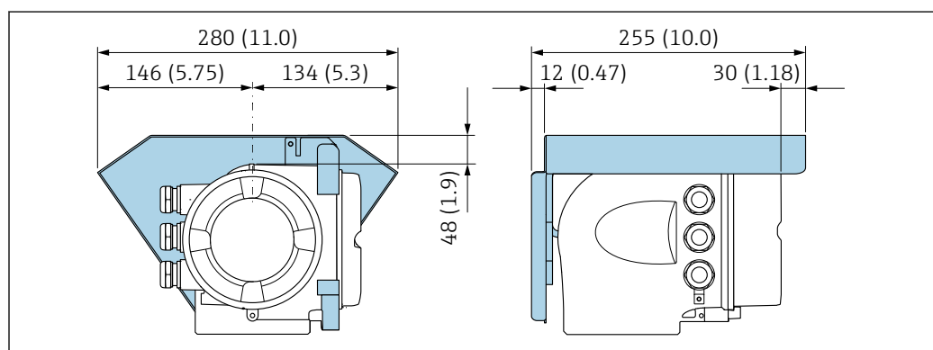
图 46 Proline 500 (模拟) 的防护罩
