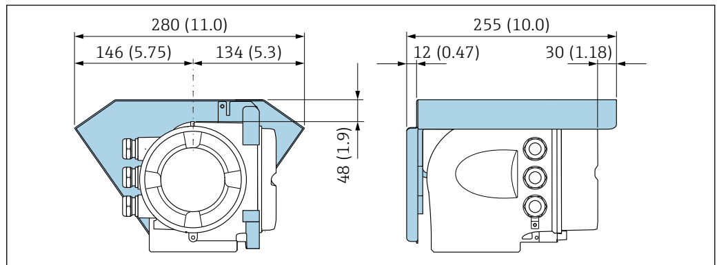
27 Proline 500 (模拟) 的防护罩
