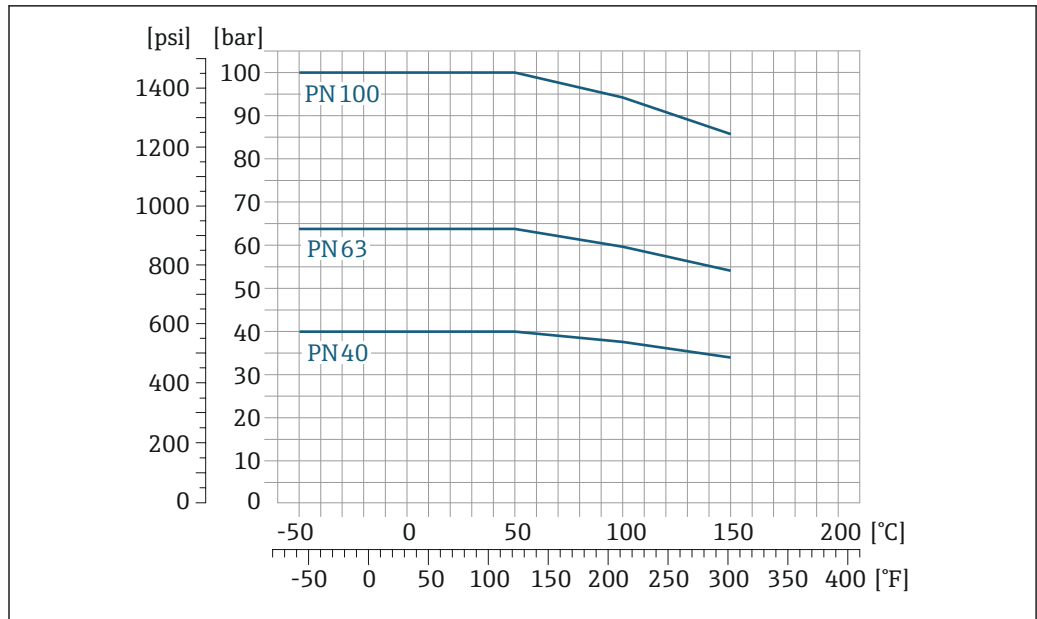
29 法兰材质: 1.4301 (304) ; 接液部件材质: 钛
