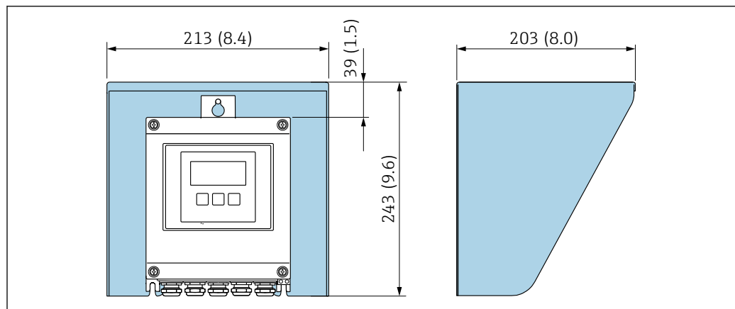
图 45 Proline 500 (数字) 的防护罩
