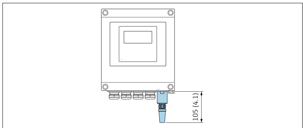
图 41 单位: mm (in)
