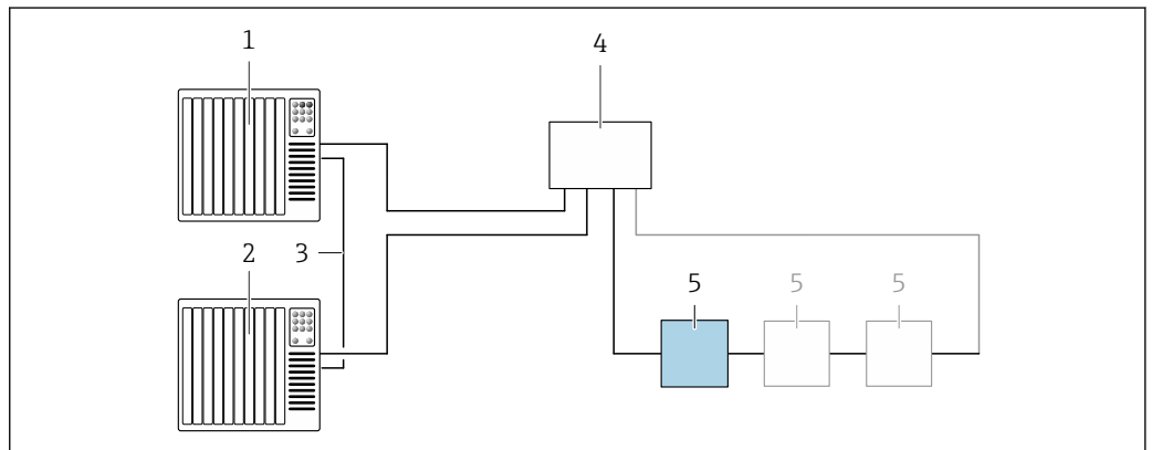
☒ 9 S2 系统冗余的连接示例
