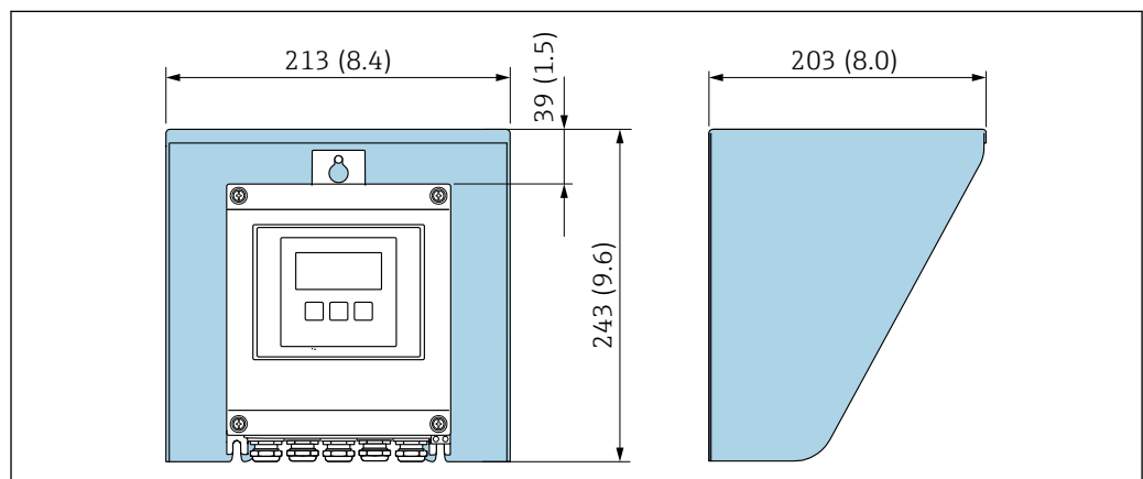
图 41 Proline 500 (数字) 的防护罩
