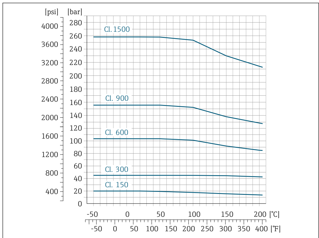
图 31 法兰材质: 不锈钢 1.4410/F53 25Cr Duplex (超级双相钢)
