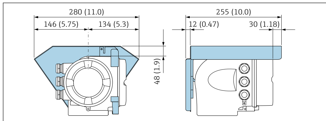
图 36 Proline 500 (模拟) 的防护罩
