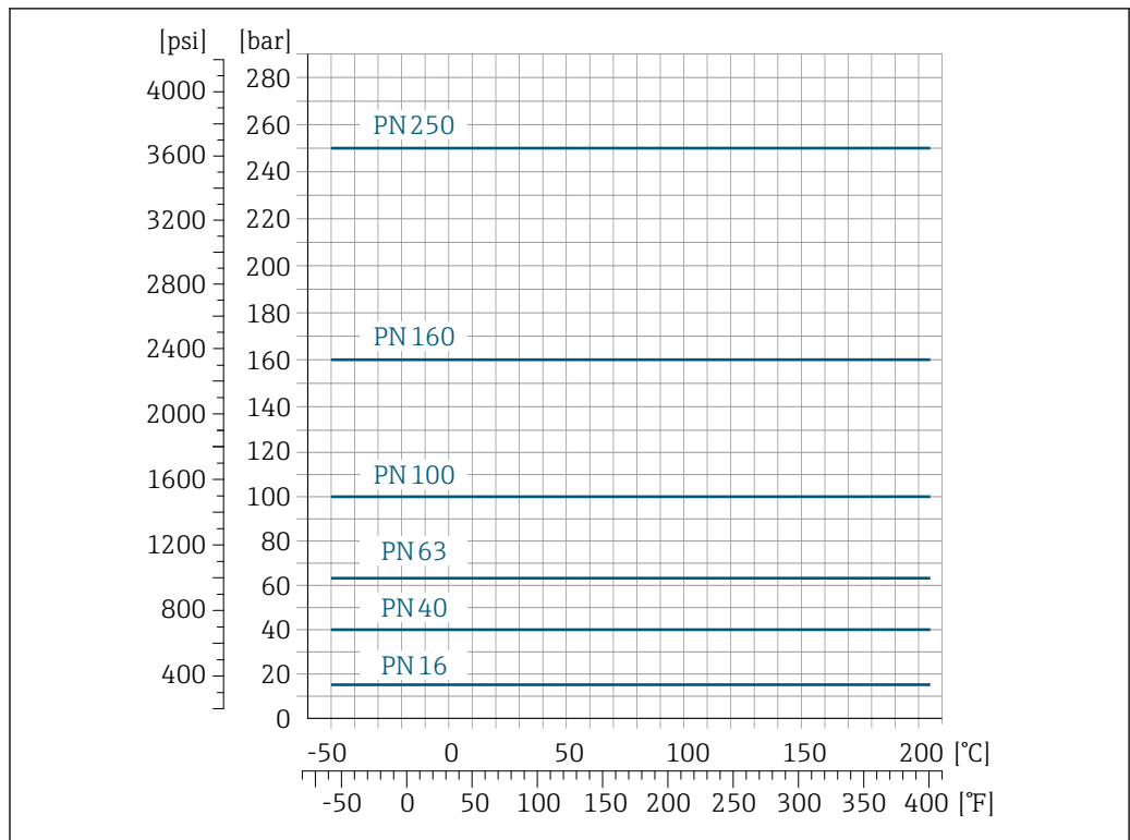
图 30 法兰材质: 不锈钢 1.4410/F53 25Cr Duplex (超级双相钢)
