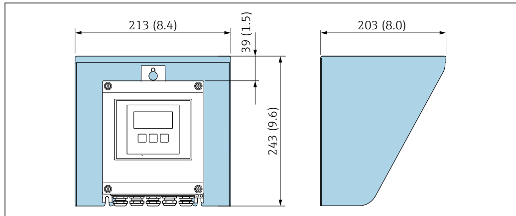
图 35 Proline 500 (数字) 的防护罩
