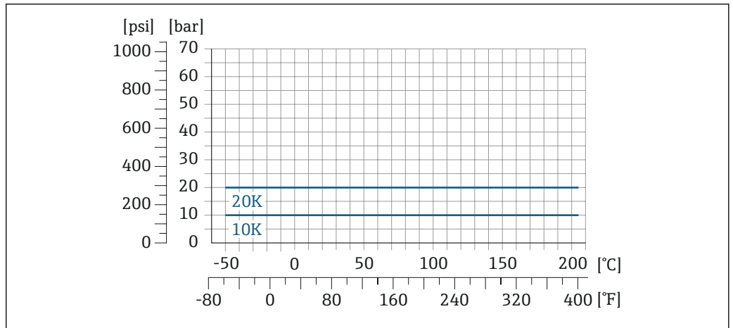
图 32 法兰材质: 不锈钢 1.4410/F53 25Cr Duplex (超级双相钢)
