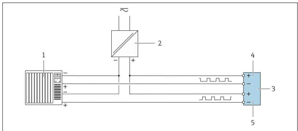
图 23 双脉冲输出(无源信号)的连接实例
