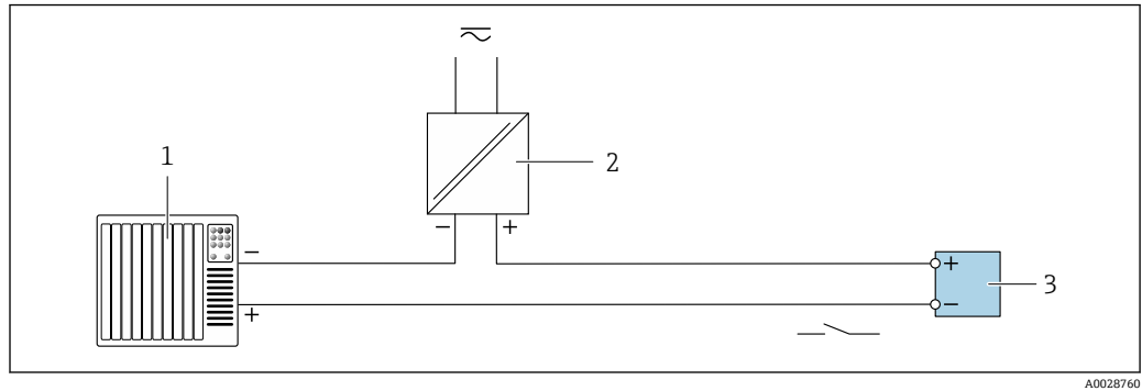
图 21 开关量输出(无源信号)的连接实例
