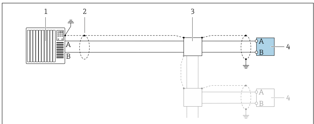
图 17 Modbus RS485 的连接实例，在非危险区和 Zone 2；Cl. I, Div. 2 防爆场合中
