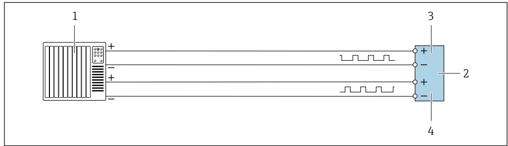
图 22 双脉冲输出(有源信号)的连接实例
