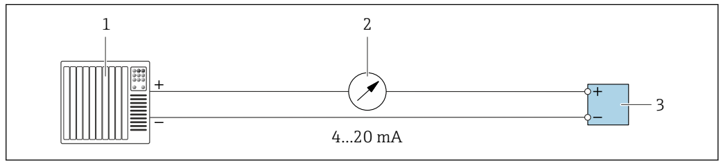
图 18 4...20 mA 有源电流输出的连接示例
