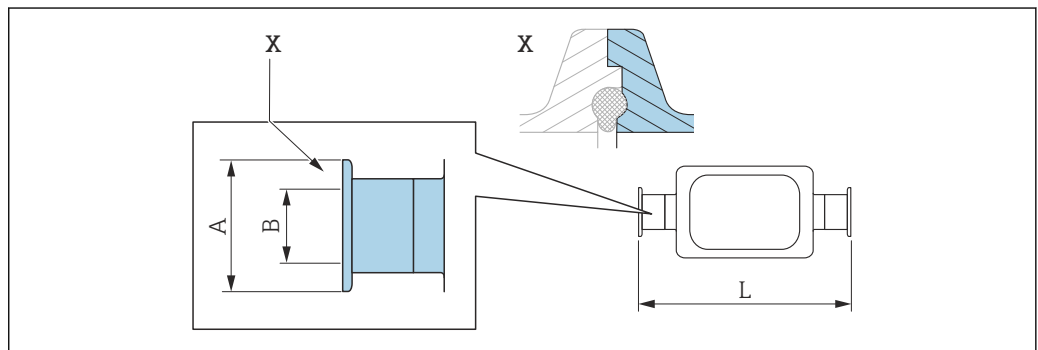
48 视图 X: 非对称过程连接; 蓝色部分由供应商提供
