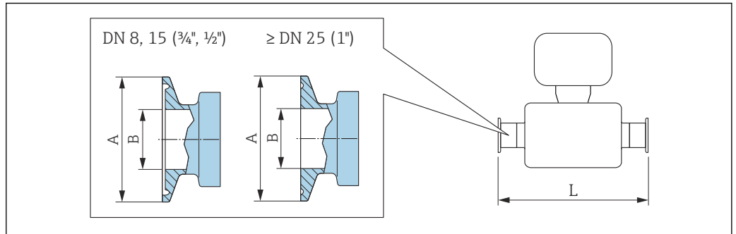
图 44 单位: mm (in)
