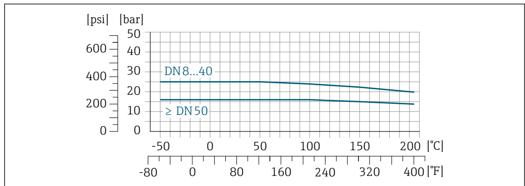
图 33 法兰材质: 1.4435 (316L)
