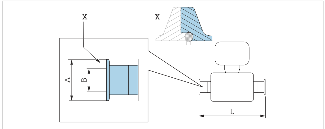
图 60 视图 X: 非对称过程连接; 蓝色部分由供应商提供
