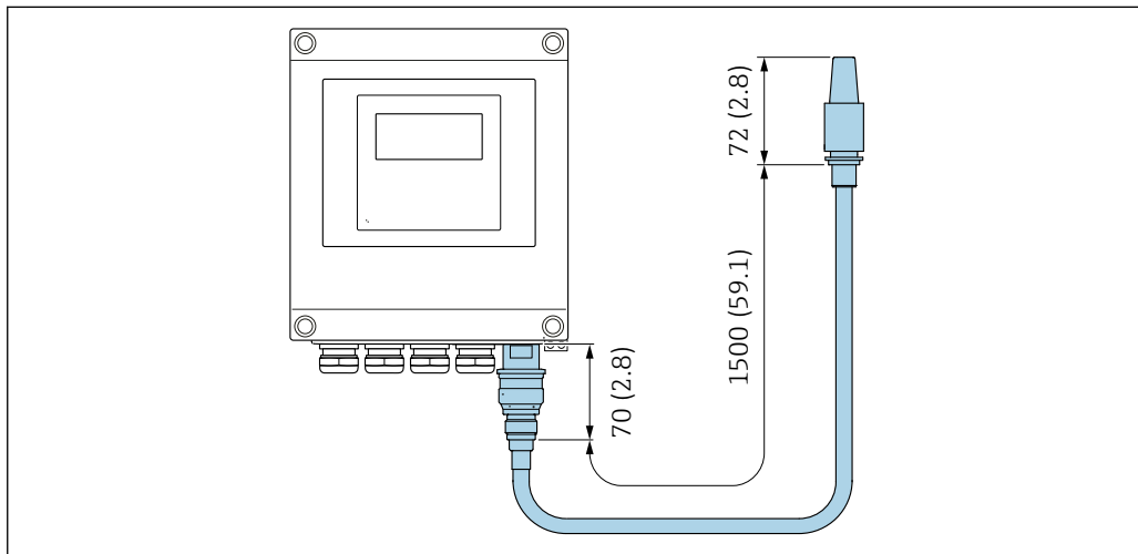
图 66 单位: mm (in)
