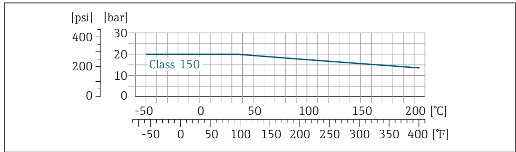
图 31 法兰材质: 1.4404 (F316/F316L)
