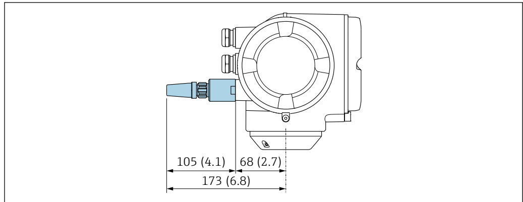
图 56 单位: mm (in)
