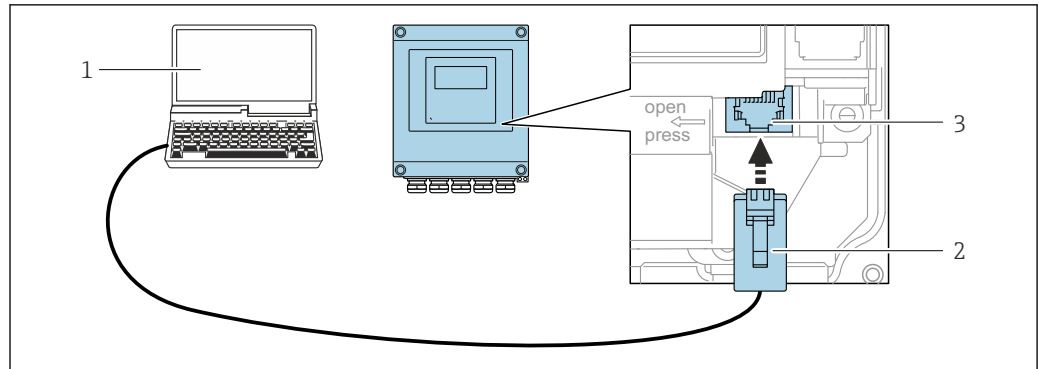
81 通过服务接口 (CDI-RJ45) 连接
