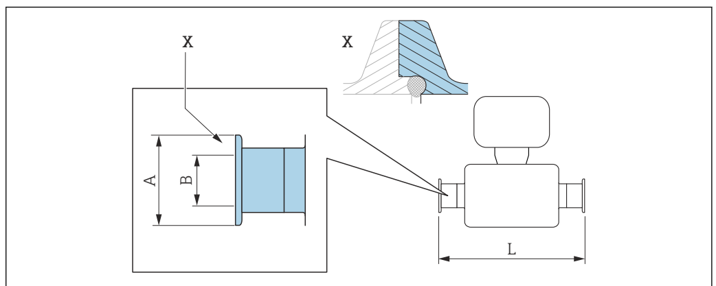
47 视图 X: 非对称过程连接; 蓝色部分由供应商提供
