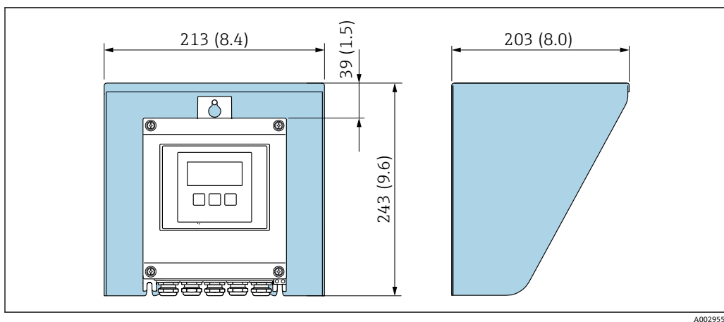
图 63 Proline 500 (数字) 的防护罩
