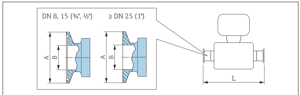
☑ 59 单位: mm (in)
