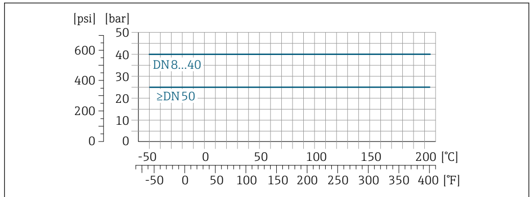
35 转接法兰材质: 1.4435 (316L)
