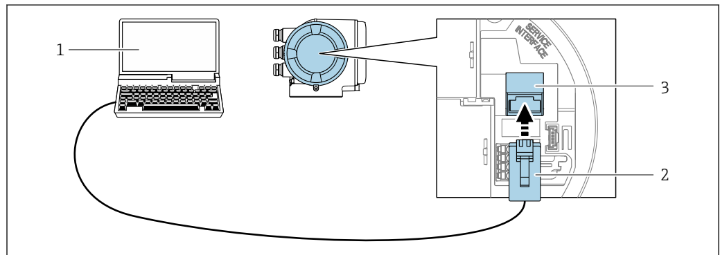
82 通过服务接口 (CDI-RJ45) 连接
