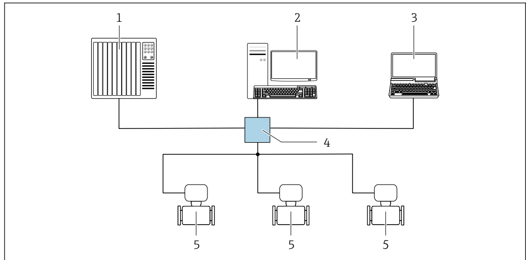
图 77 通过 EtherNet/IP 网络实现远程操作：星形拓扑结构
