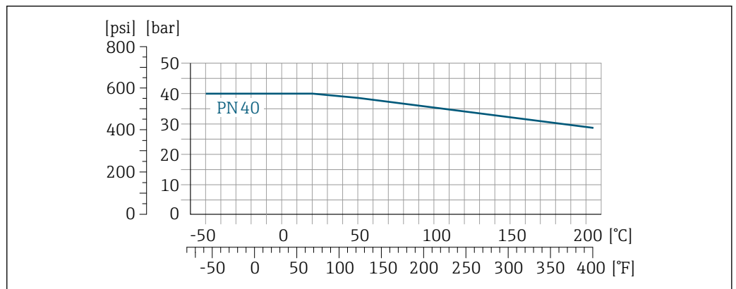
图 30 法兰材质: 1.4404 (F316/F316L)
