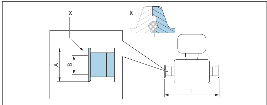
图 45 视图 X: 非对称过程连接; 蓝色部分由供应商提供
