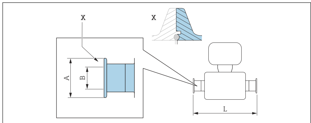
图 46 视图 X: 非对称过程连接; 蓝色部分由供应商提供
