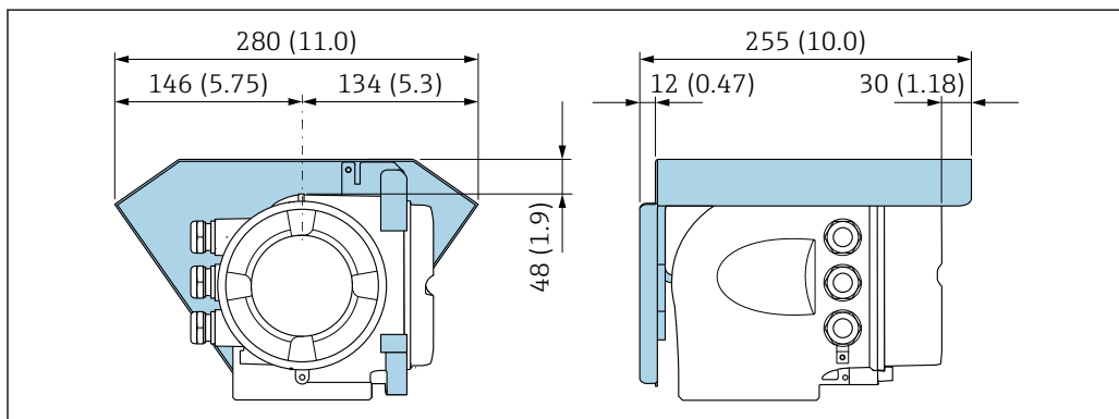
图 64 Proline 500 (模拟) 的防护罩
