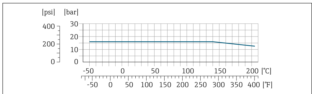
图 34 法兰材质: 1.4435 (316L)
