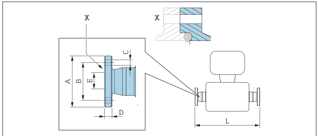
☑ 58 视图 X: 非对称过程连接; 蓝色部分由供应商提供
