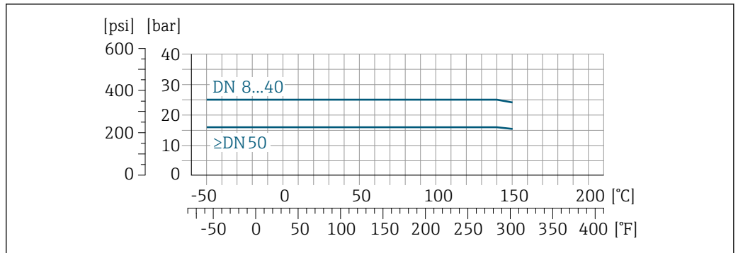
☑ 27 法兰材质: 1.4435 (316L)
