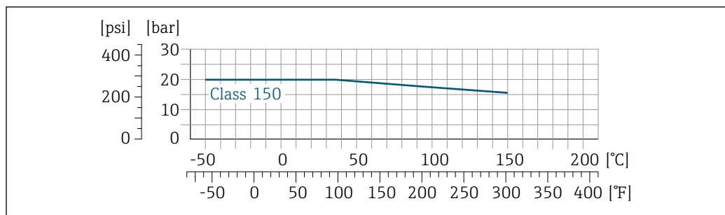
图 25 法兰材质: 1.4404 (F316/F316L)
