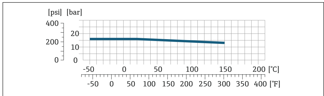
图 30 连接部件材质: 1.4435 (316L)
