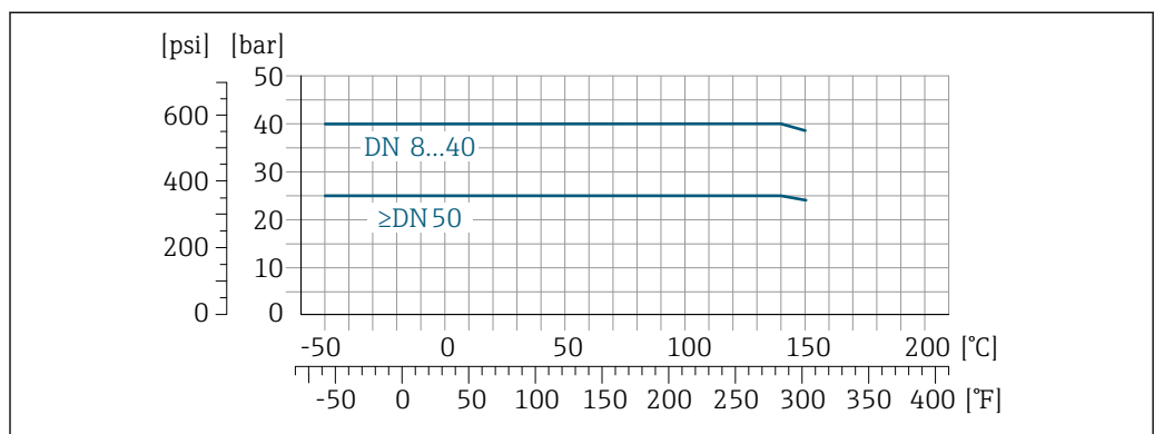
图 32 连接部件材质: 1.4435 (316L)
