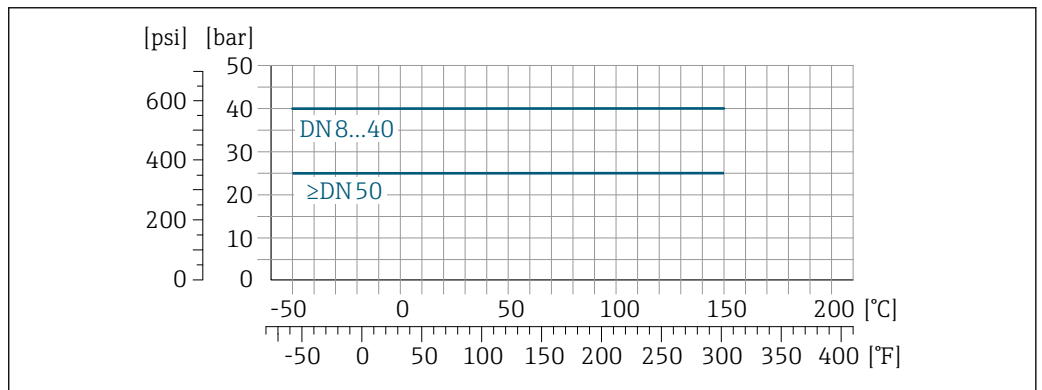
☑ 28 转接法兰材质: 1.4435 (316L)
