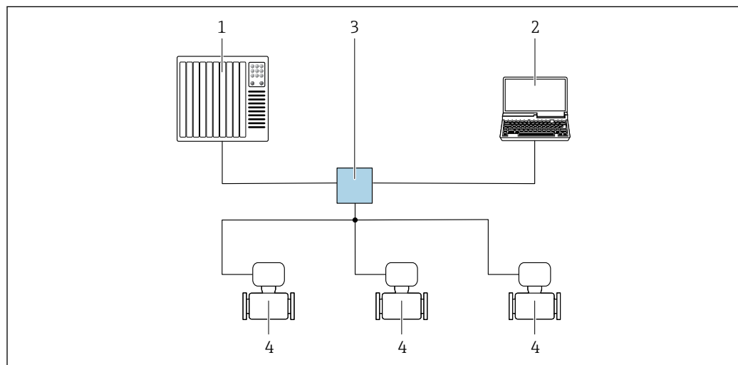
图 55 通过 PROFINET 网络实现远程操作：星形拓扑结构
