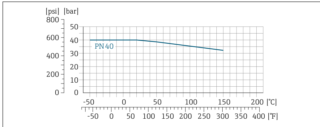
图 24 法兰材质: 1.4404 (F316/F316L)
