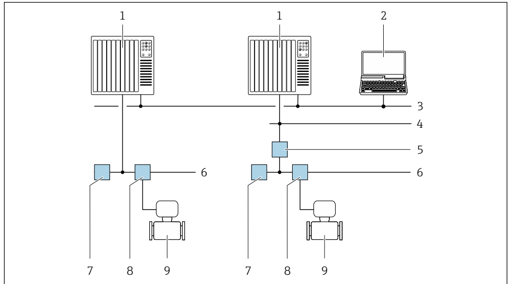
图 49 通过基金会现场总线(FF)网络进行远程操作
