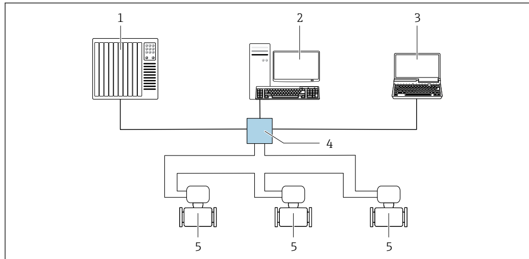
图 54 通过 EtherNet/IP 网络实现远程操作：环形拓扑结构
