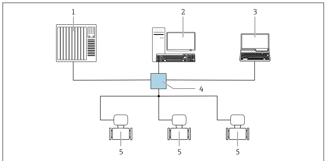
图 53 通过 EtherNet/IP 网络实现远程操作: 星形拓扑结构
