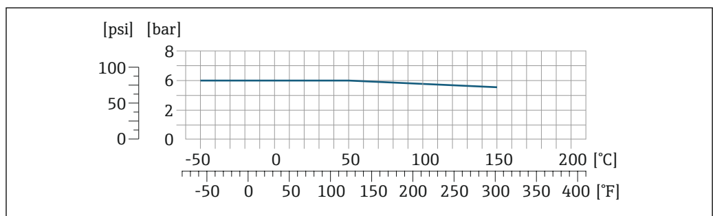
图 31 连接部件材质: 1.4435 (316L)
