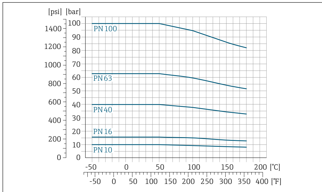
图 24 法兰材质: 1.4404 (316/316L)
