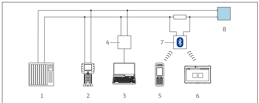
图 40 通过 HART 通信进行远程操作（有源信号）
