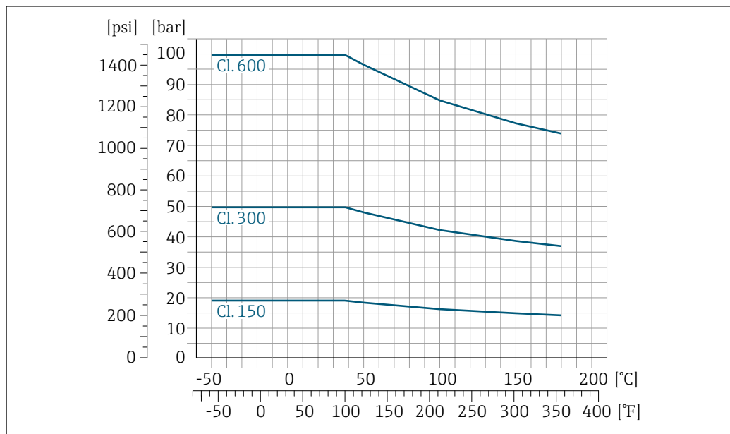
图 25 法兰材质: 1.4404 (316/316L)
