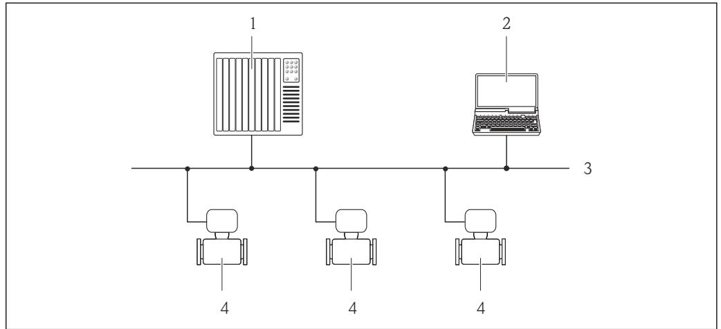
43 通过 PROFIBUS DP 网络进行远程操作
