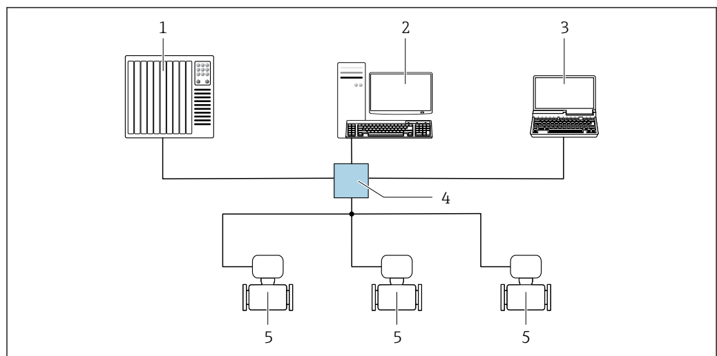
图 46 通过 EtherNet/IP 网络实现远程操作: 星形拓扑结构
