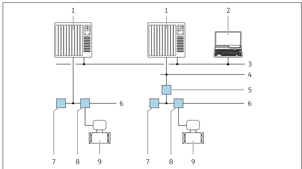
图 42 通过基金会现场总线(FF)网络进行远程操作
