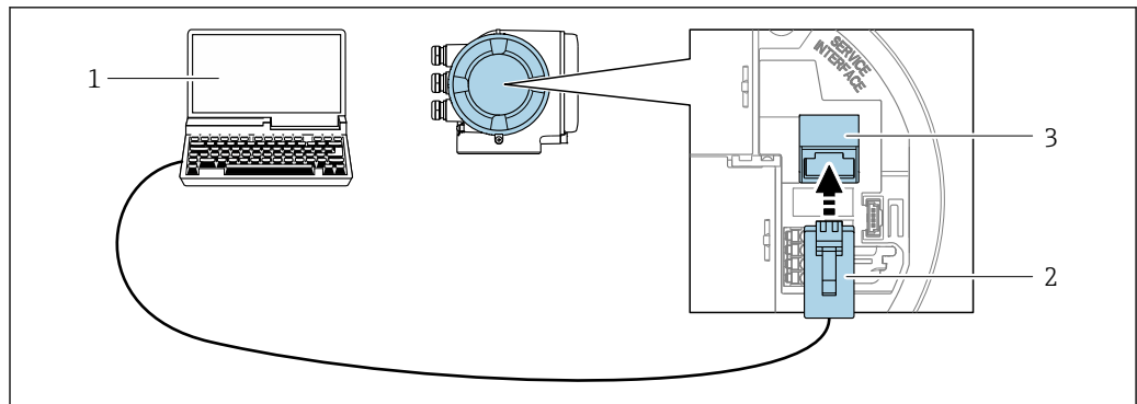
图 50 通过服务接口（CDI-RJ45）连接
