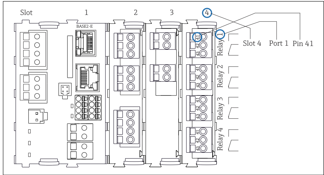
图 7 带常开触点 (NO) (41 号接线端子) 的继电器的接线端子示意图
