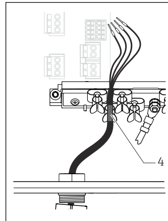
图 37 将电缆安装在接地夹中
