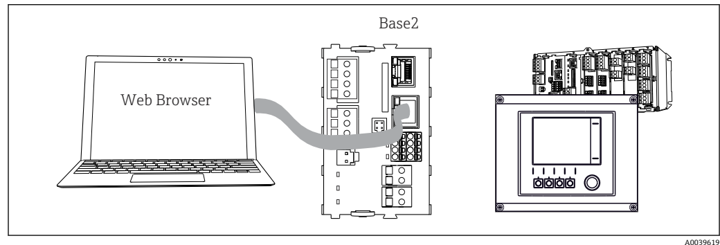
图 81 网页服务器/以太网连接
