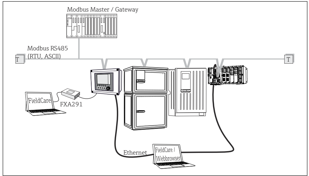
图 30 Modbus RS485
