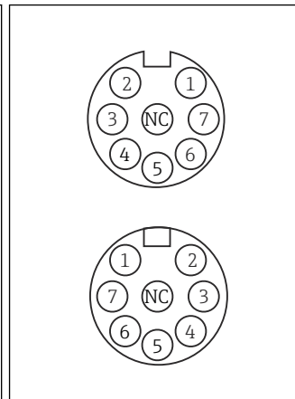
50 M12 连接头引脚分配; 上图为插座; 下图为插头 (均为俯视图) 1 PK (粉) : 24 V 2 GY (灰) : 24 V 接地 3 BN (棕) : 3 V 4 WH (白) : 3 V 接地 5 GN (绿) : Memosens 信号 6 YE (黄) : Memosens 信号 7 悬空 (N C)
