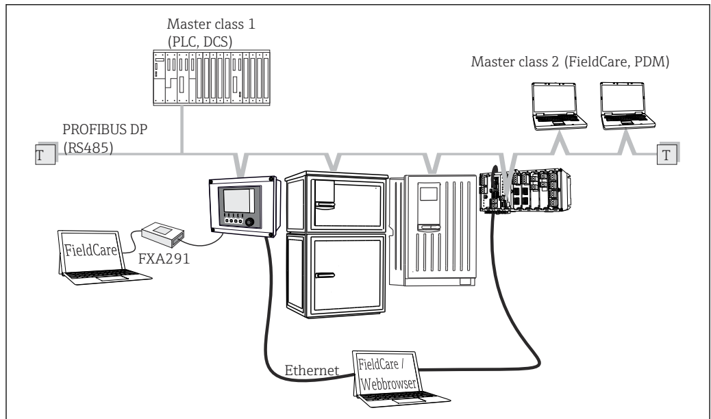
图 29 PROFIBUS DP
