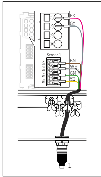
49 M12 连接头连接 (例如在传感器模块上) 1 传感器电缆, 带 M12 插头
