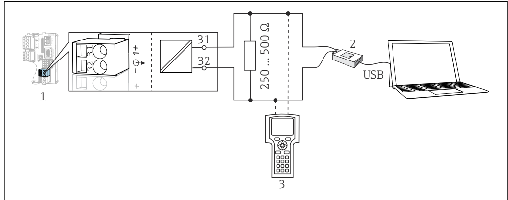
图 28 HART 通信, 使用调制解调器
