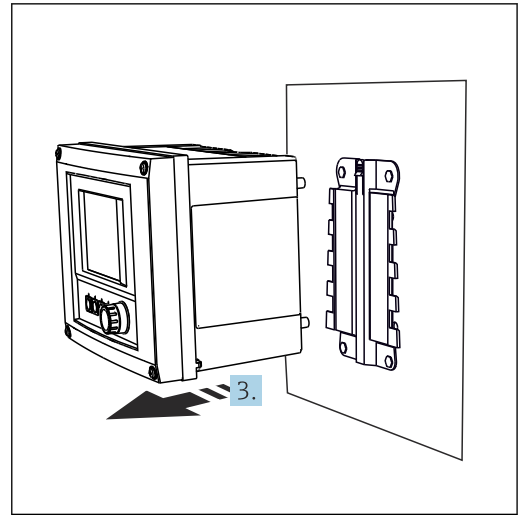
图 26 拆卸
