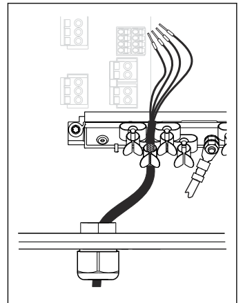
图 38 将电缆安装在接地夹中
