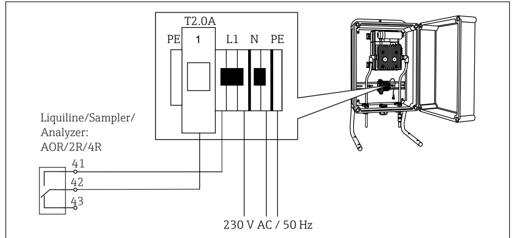
图 64 连接 CAS40D 的清洗单元
