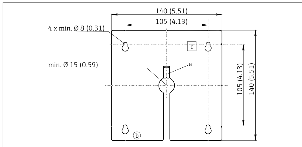
图 14 外接显示单元的安装背板的外形尺寸；单位：mm (in)
