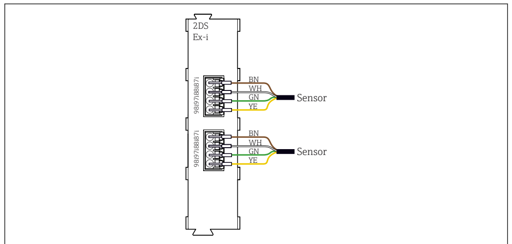
51 传感器和本安 Ex-i 型传感器通信模块 2DS, 不带附加电源
