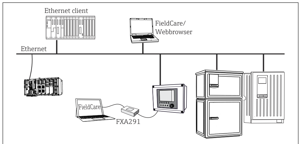
图 31 Modbus TCP 或 EtherNet/IP 或 PROFINET
