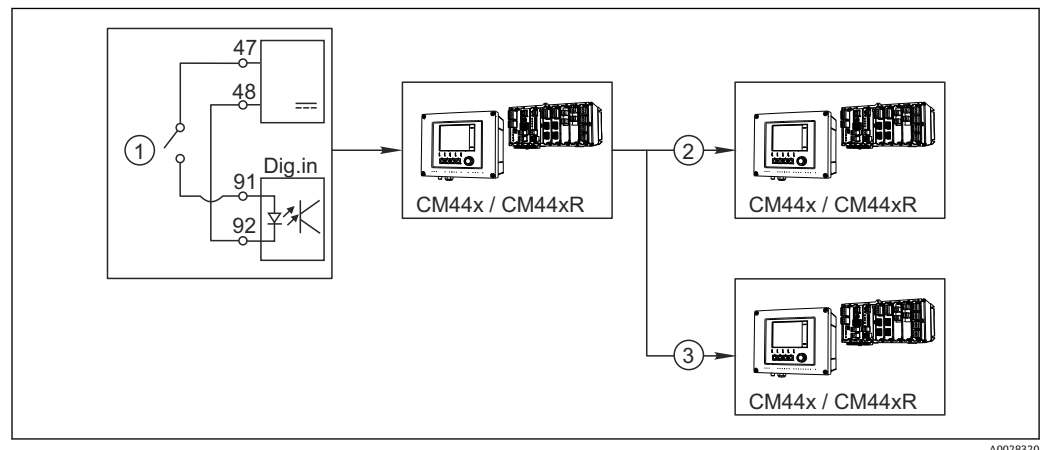
图 88 中央清洗控制实例
