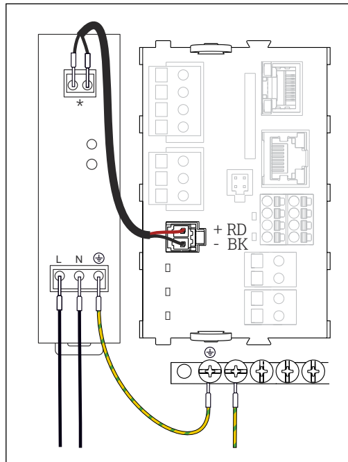
图 41 BASE2-E 模块的电源接线示意图（机柜盘装型设备）
