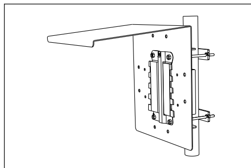
16 管装意图
