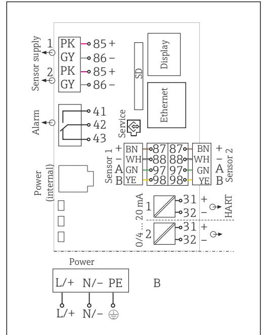
图 40 BASE2-E 模块和扩展供电单元 (B) 的完整接线图
