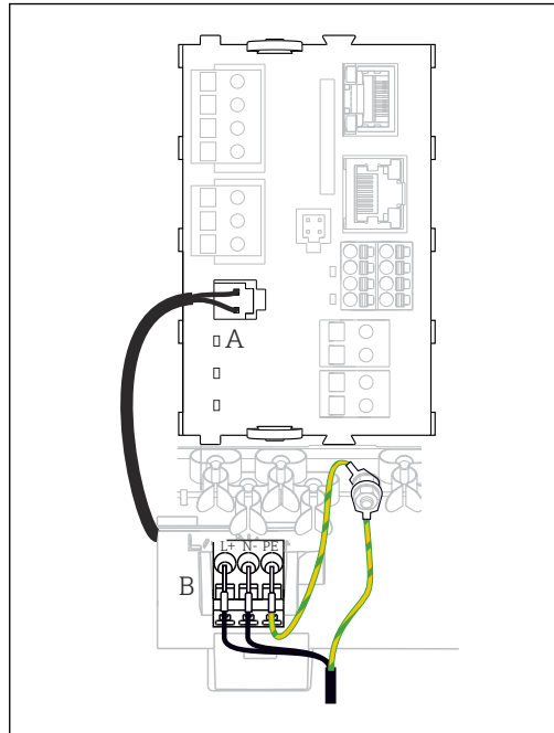
图 39 BASE2-E 电源接线示意图（现场型设备）
