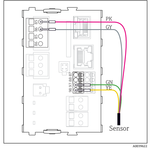
46 Memosens 数字式传感器, 连接附加电源
