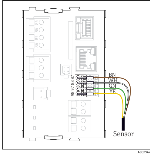
45 Memosens 数字式传感器, 不连接附加电源
