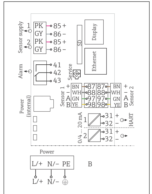
图 42 BASE2-E 模块和外接供电单元 (B) 的完整接线图
