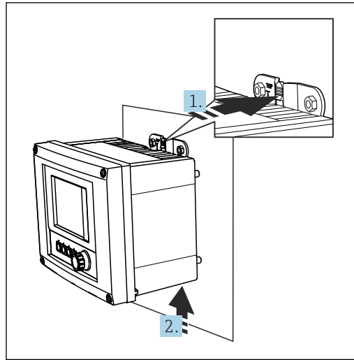
图 25 拆卸
