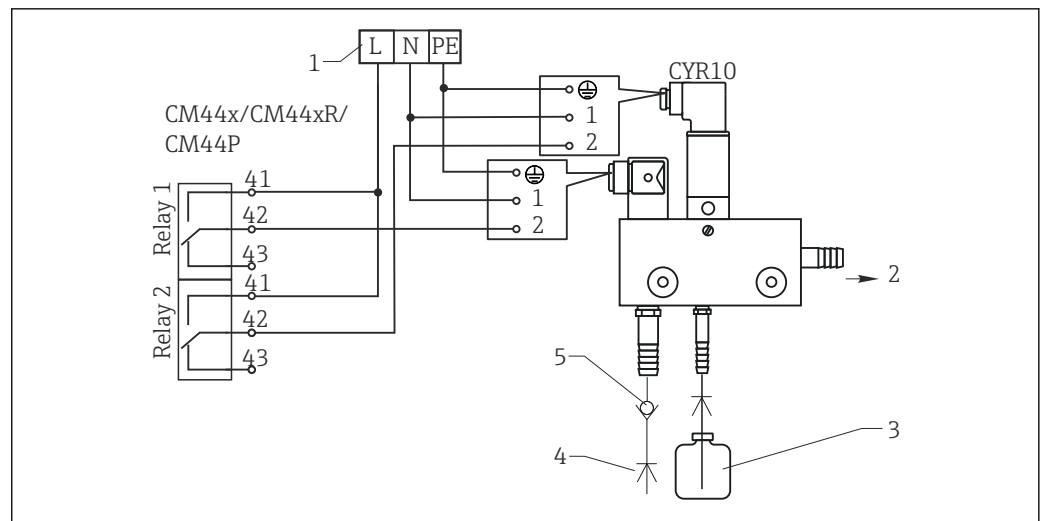
图 65 Chemoclean CYR10 清洗单元接线图
