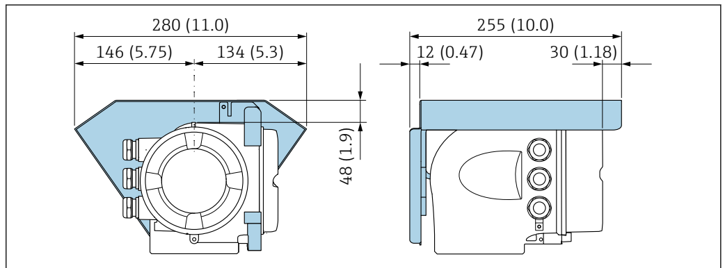
41 Proline 500 的防护罩
