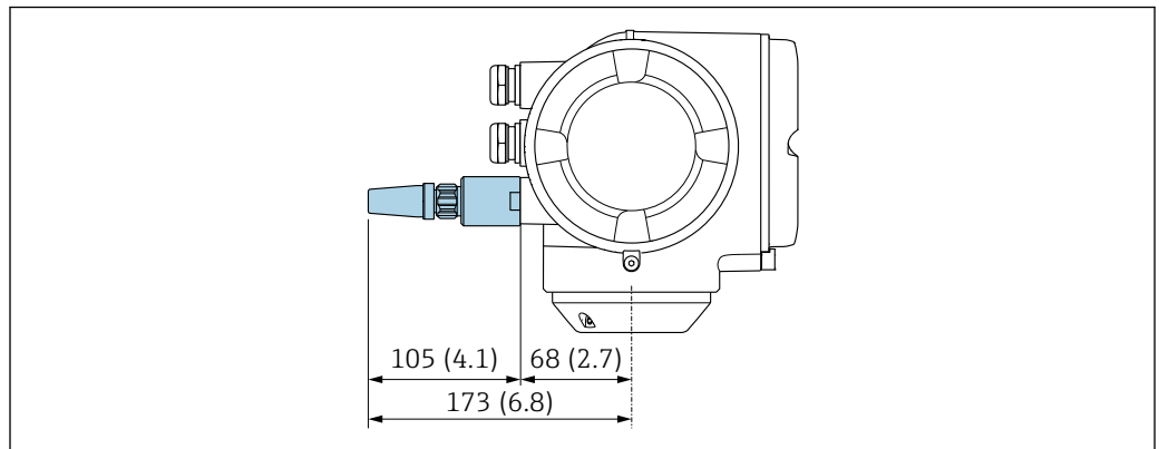
图 50 单位: mm (in)
