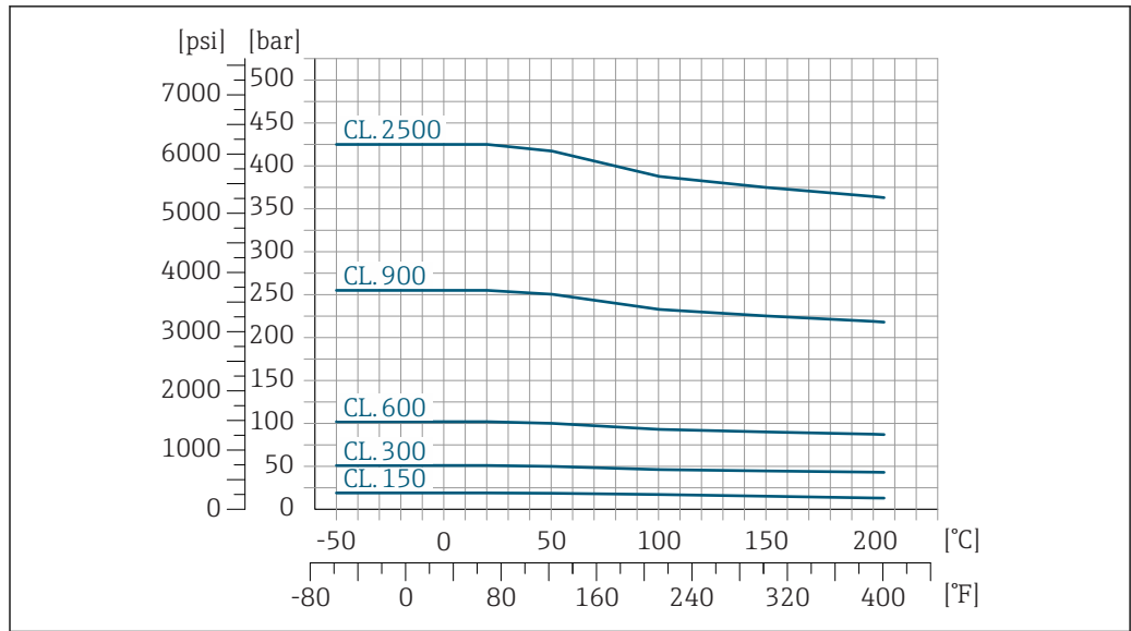
图 31 法兰材质: 1.4404 (316/316L)
