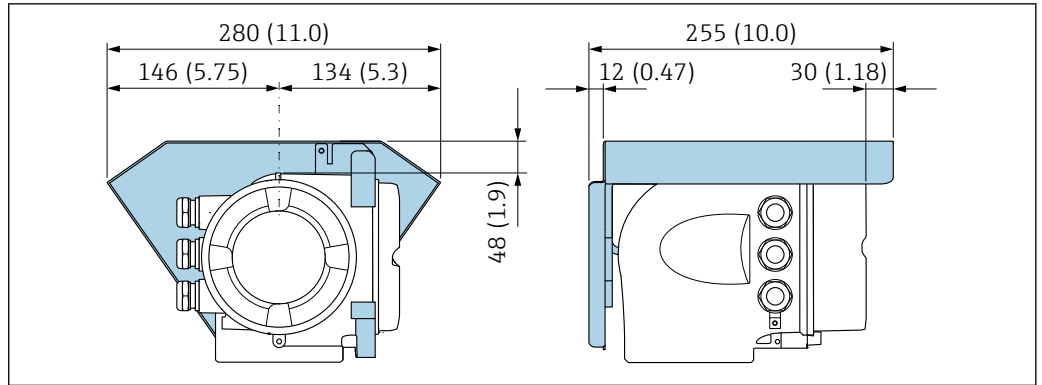
图 26 Proline 500 的防护罩
