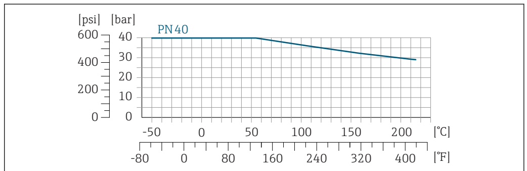
30 松套法兰材质: 1.4301 (F304); 接液部件材质: Alloy C22 2.4602 (UNS N06022)合金
