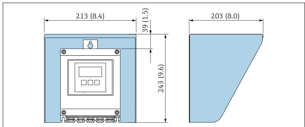
图 25 Proline 500 (数字式) 的防护罩
