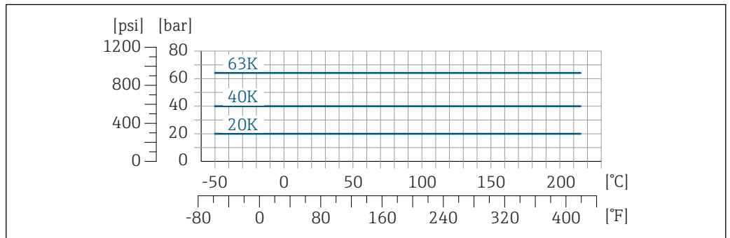
34 法兰材质: 1.4404 (316/316L)或 Alloy C22 2.4602 (UNS N06022)合金
