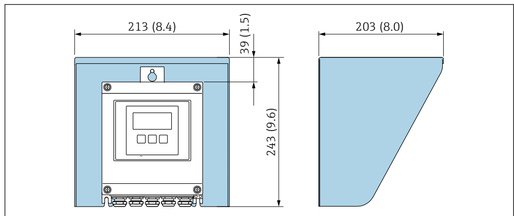
46 Proline 500 (数字式) 的防护罩
