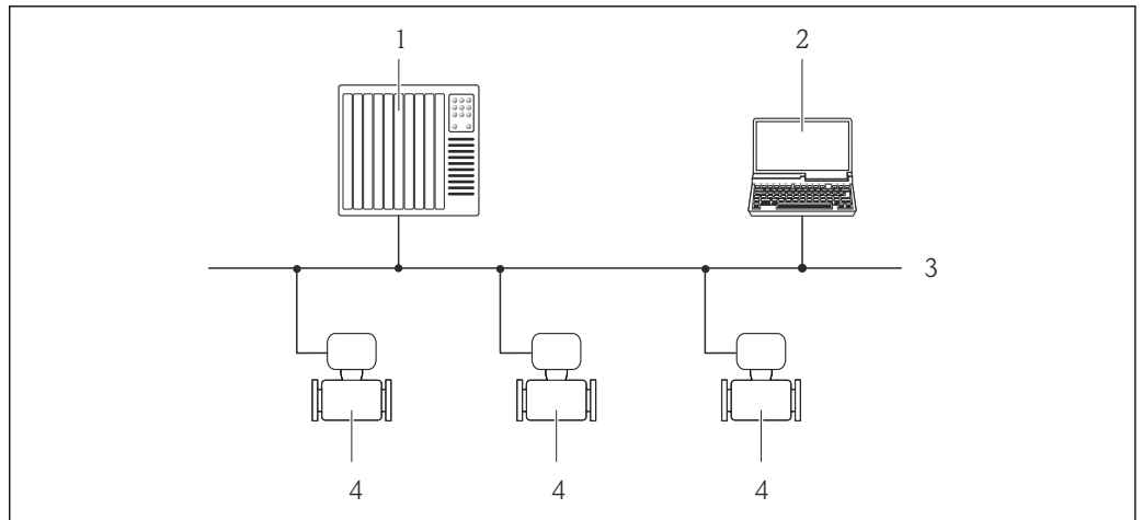
57 通过 PROFIBUS DP 网络进行远程操作
