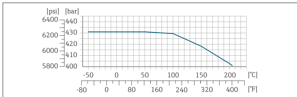
图 38 法兰材质: Alloy C22 2.4602 (UNS N06022)合金
