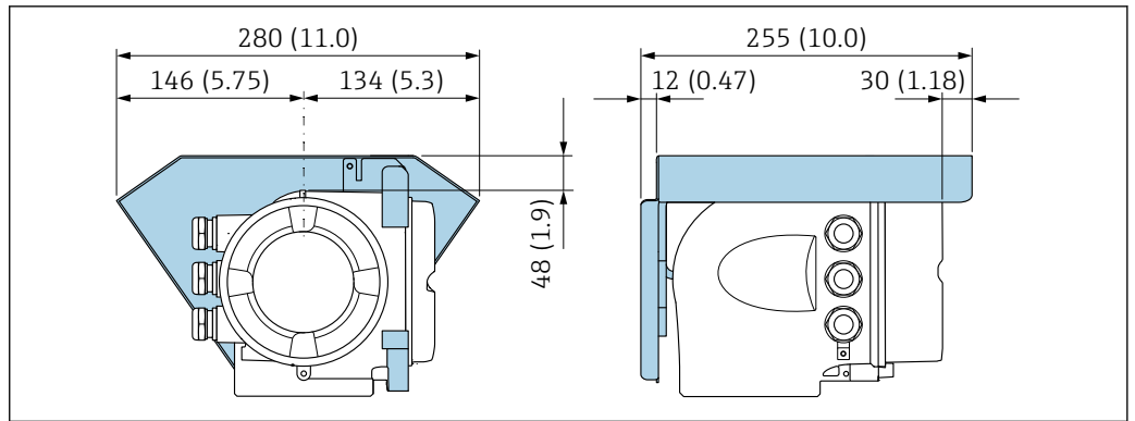
图 47 Proline 500 的防护罩
