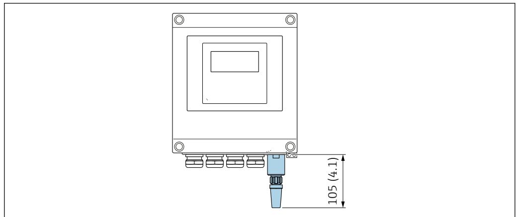
42 单位: mm (in)
