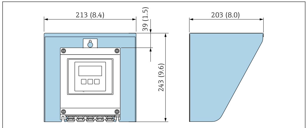
40 Proline 500 (数字式) 的防护罩
