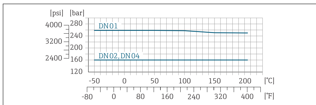
图 37 法兰材质: Alloy C22 2.4602 (UNS N06022)合金
