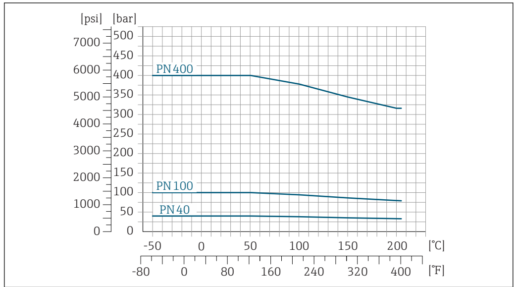
28 法兰材质: 1.4404 (316/316L)
