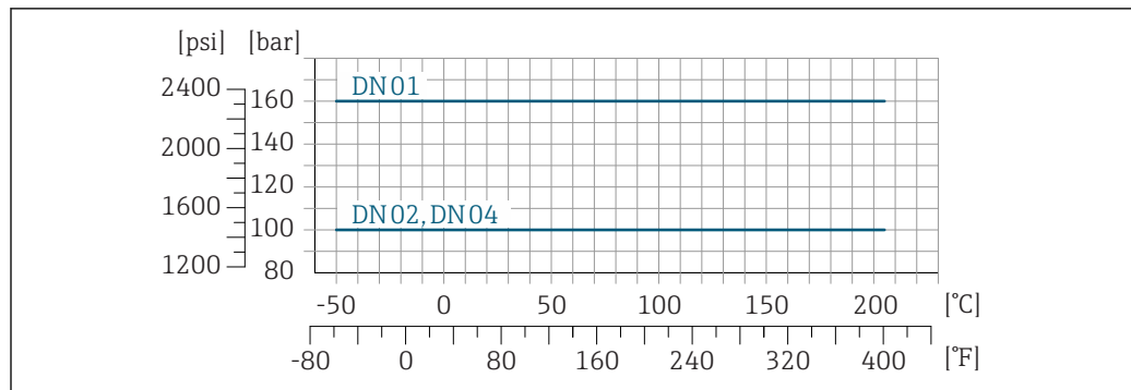
图 36 法兰材质: 1.4404 (316/316L)
