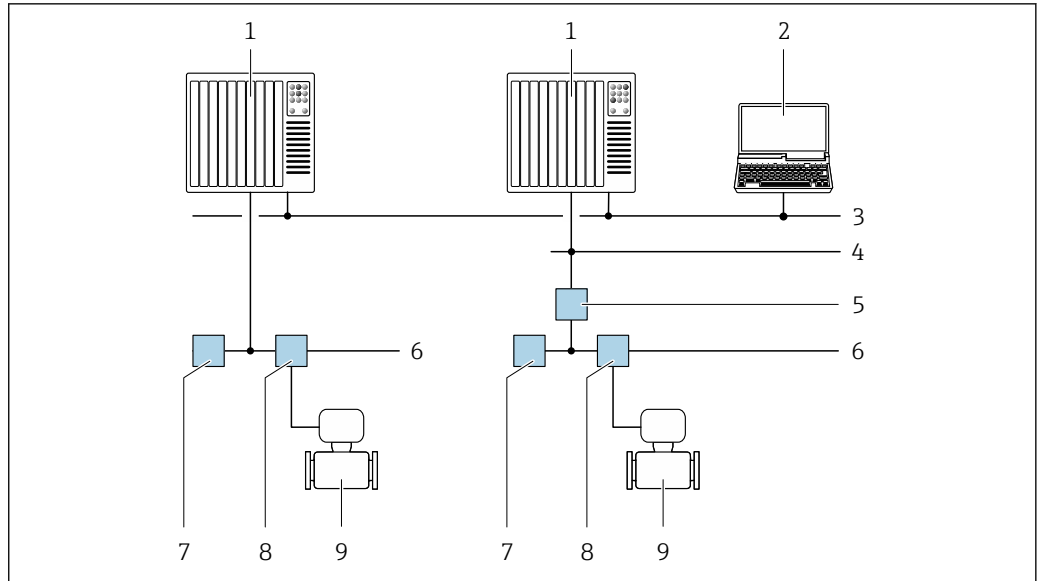
56 通过基金会现场总线(FF)网络进行远程操作
