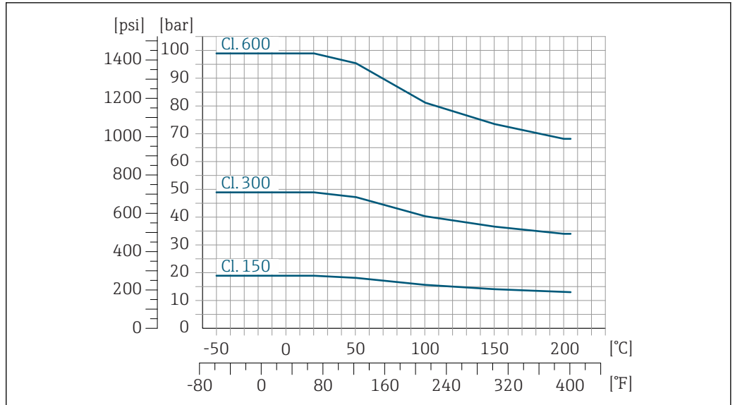
33 松套法兰材质: 1.4301 (F304); 接液部件材质: Alloy C22: 2.4602 (UNS N06022)合金
