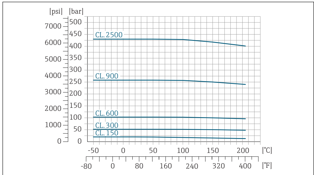
图 32 法兰材质: Alloy C22 2.4602 (UNS N06022)合金
