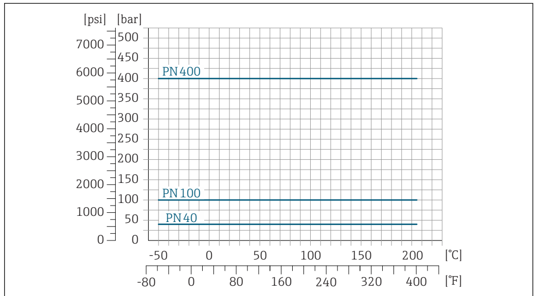
29 法兰材质: Alloy C22 2.4602 (UNS N06022)合金
