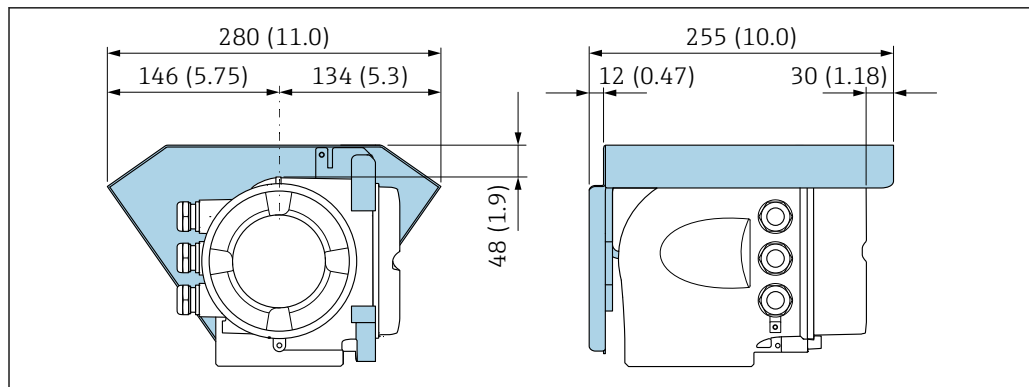
图 43 Proline 500 (模拟) 的防护罩
