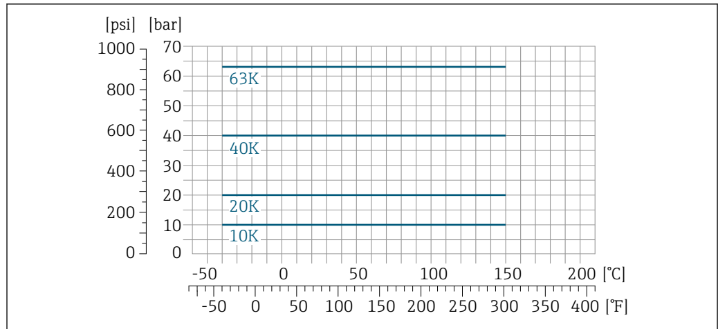
图 33 法兰材质: 1.4404 (F316/F316L)
