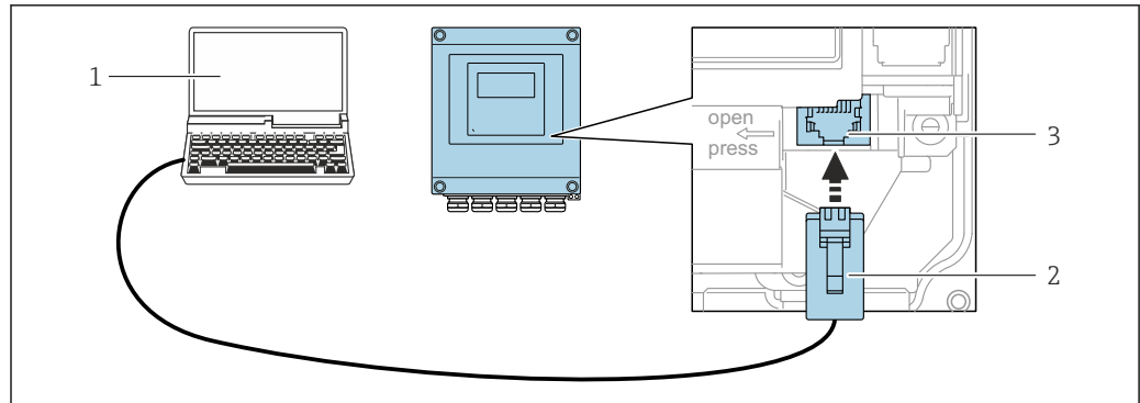
图 66 通过服务接口 (CDI-RJ45) 连接
