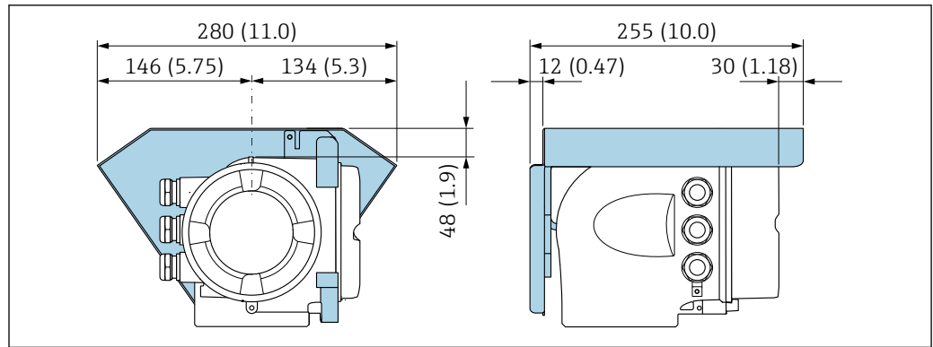
图 49 Proline 500 (模拟) 的防护罩
