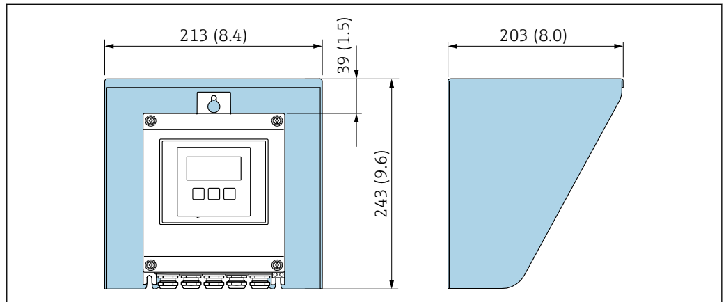
28 Proline 500 (数字) 的防护罩
