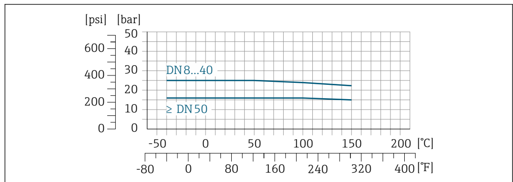
图 34 法兰材质: 1.4404 (316/316L)
