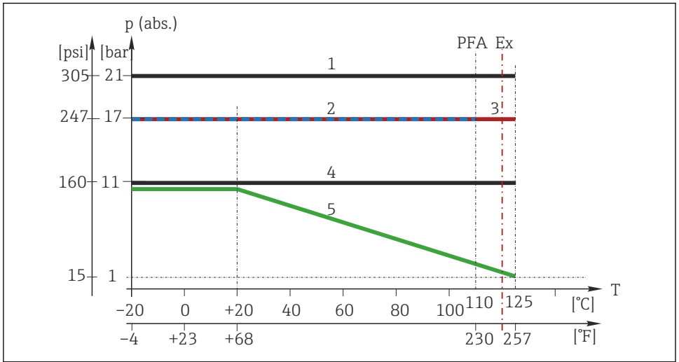
图 11 温压曲线
