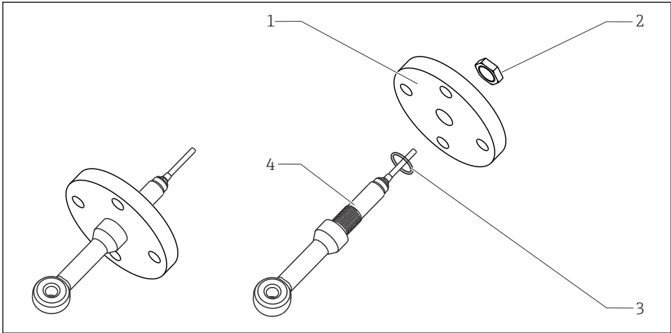
4 接液固定法兰的安装示意图(订购选项“过程连接”，选型代号 3、4)
