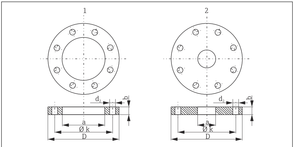
图 13 法兰外形尺寸
