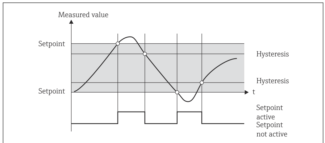
图 13 InBand 工作模式
