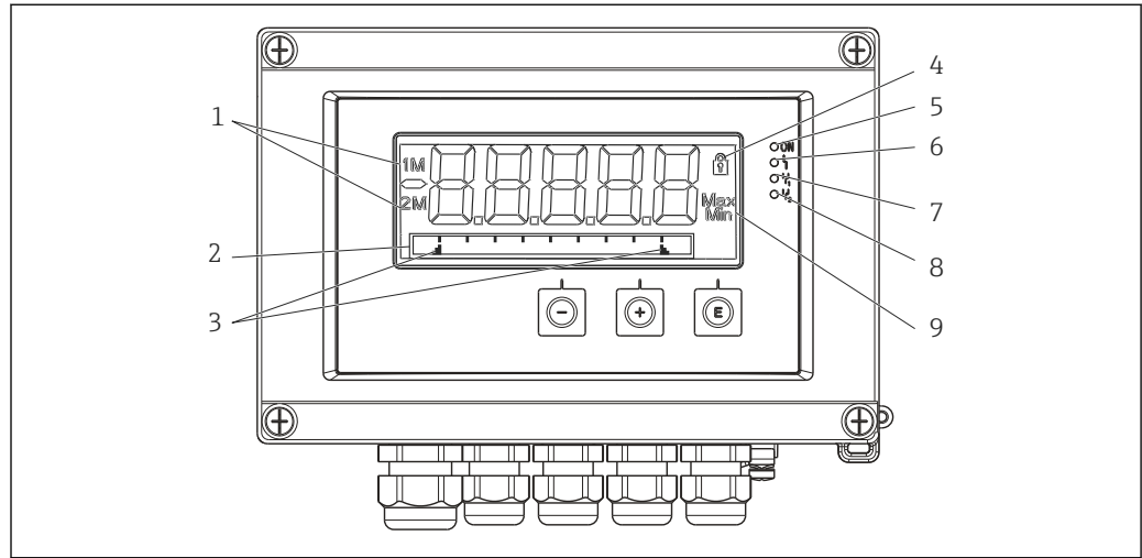
图 20 现场仪表显示屏
