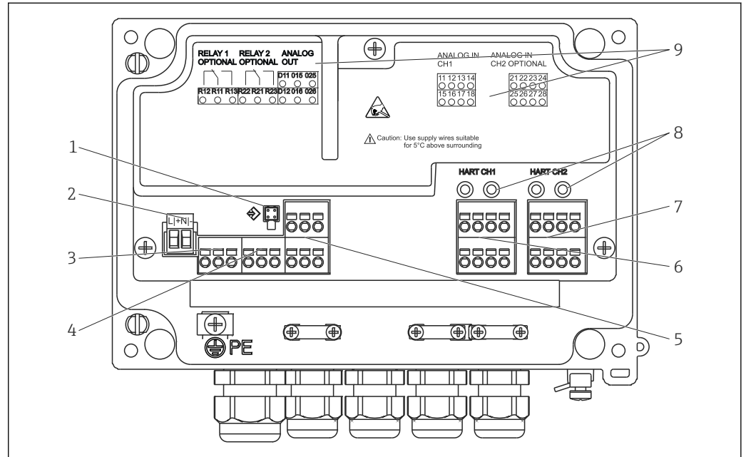
图 18 过程显示仪的内部视图和接线端子分配
