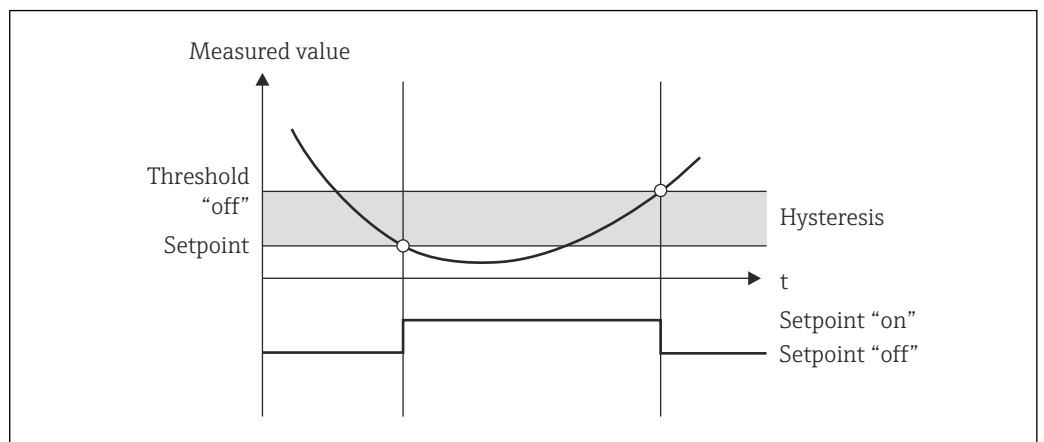
图 9 Min 工作模式
