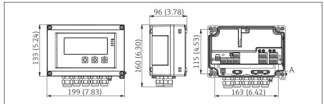
图 1 现场安装测控仪的外形尺寸示意图；单位：mm (in)
