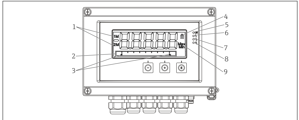
图 7 现场安装测控仪的显示屏
