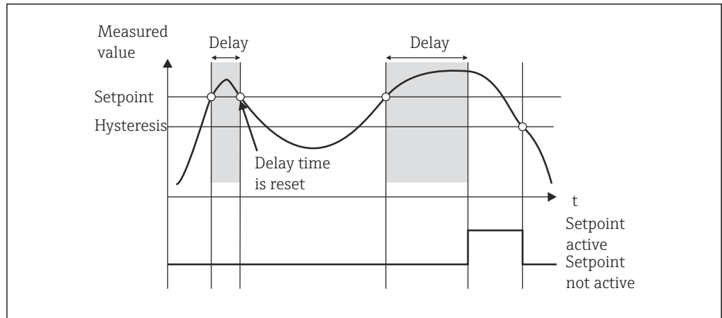
图 14 回差和延迟时间启用
