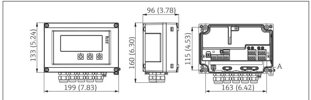
图 19 现场仪表的外形尺寸，单位：mm (in)
