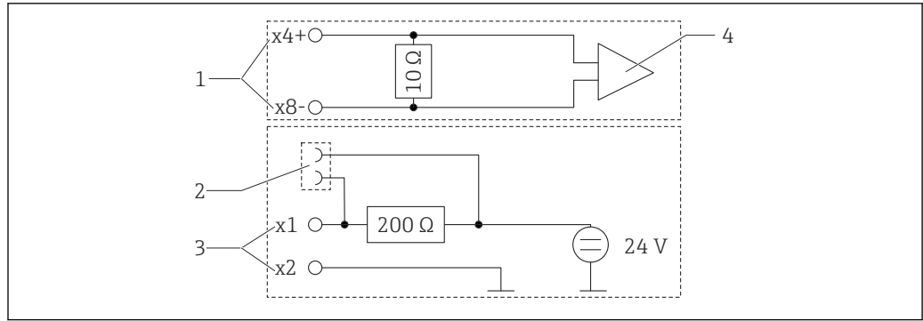
图 5 HART®连接插座的内部回路
