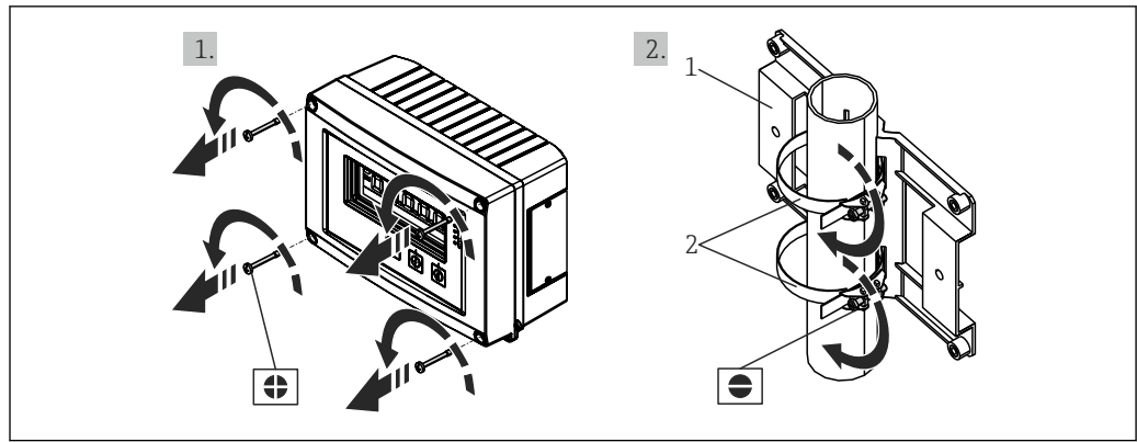
图 2 在管道上安装现场安装测控仪
