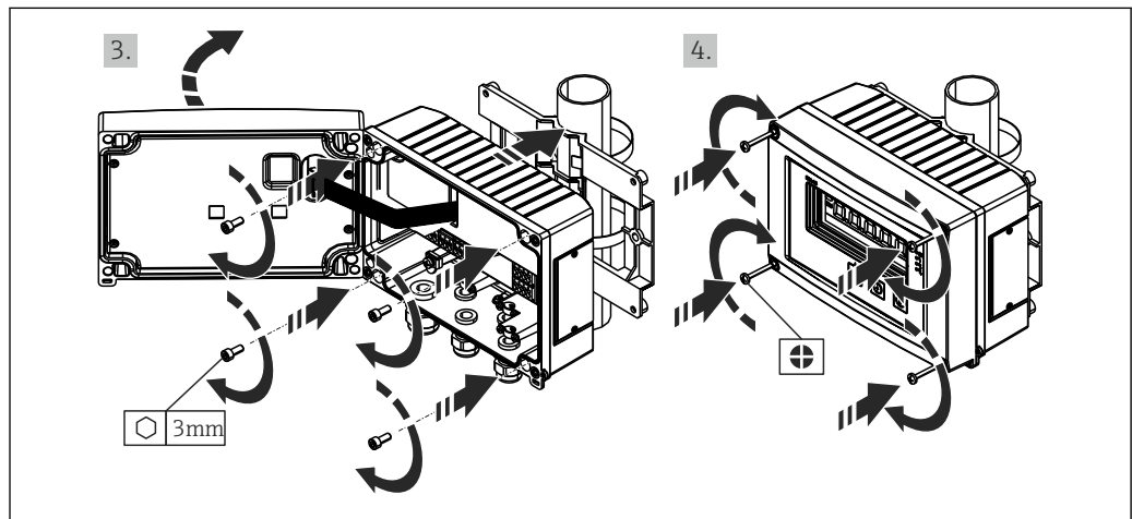
图 3 在管道上安装现场安装测控仪
