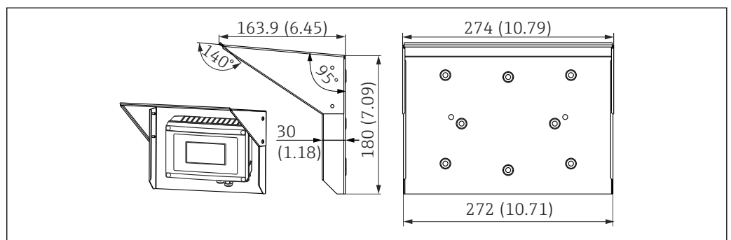
图 21 外形尺寸示意图; 单位: mm (in)
