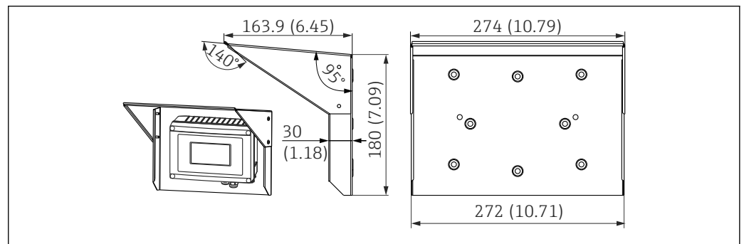
图 17 外形尺寸示意图; 单位: mm (in)
