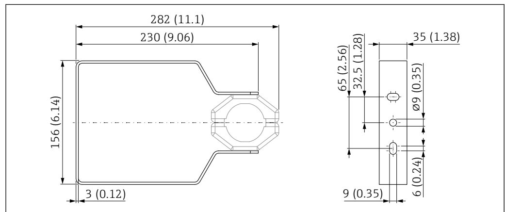
图 41 安装架的外形尺寸示意图。测量单位 mm (in)
