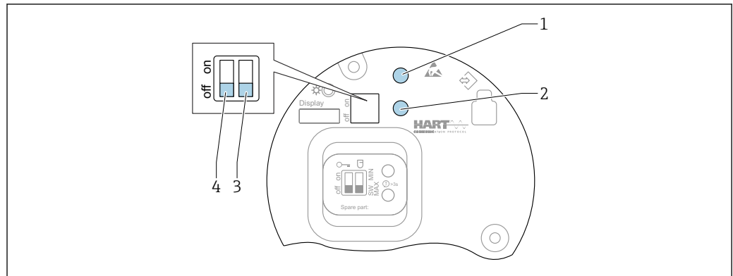
图 36 HART 电子插件上的操作按键和 DIP 开关
