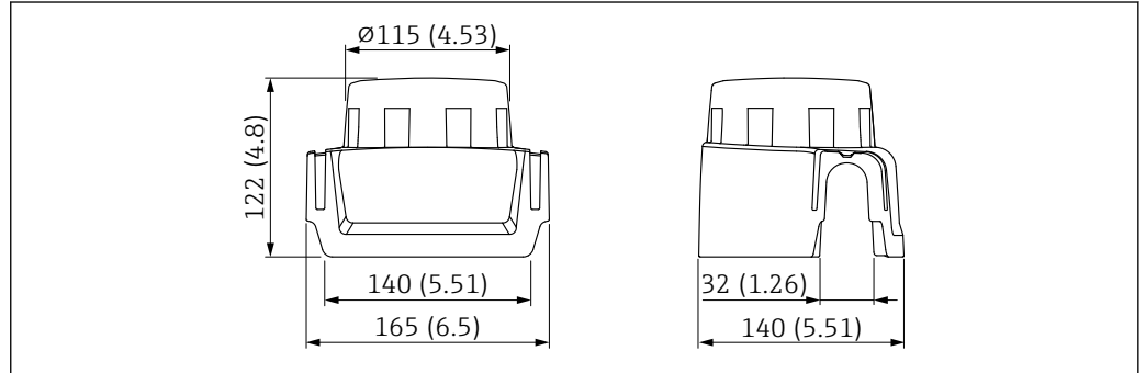
图 39 外形尺寸示意图。测量单位 mm (in)
