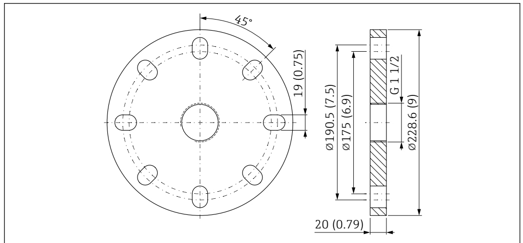
图 32 UNI 4"/DN100/100A 法兰的外形尺寸示意图。测量单位 mm (in)
