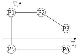
图 13 铝外壳, 带涂层; 过程温度范围: -40 ... +80 °C (-40 ... +176 °F)
