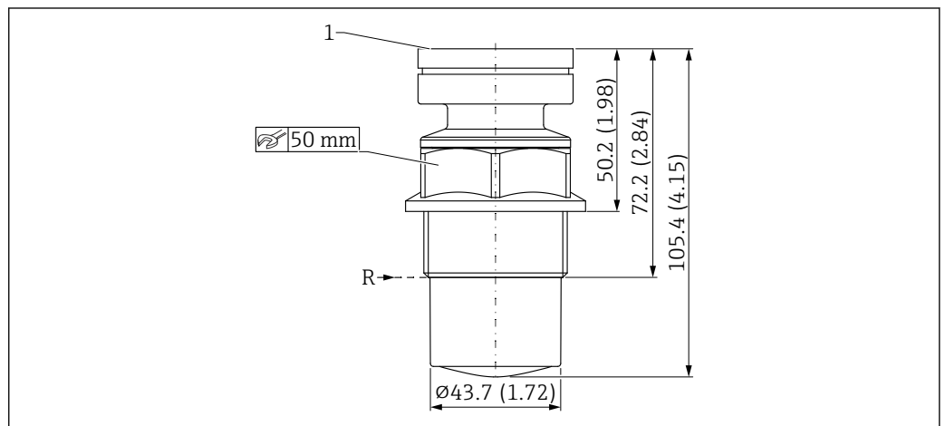
图 24 PVDF 全密封天线 (40 mm (1.5 in) 口径) 的外形尺寸示意图。测量单位 mm (in)
