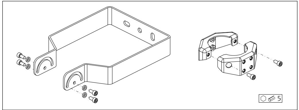
42 安装架（可调节）的供货清单
