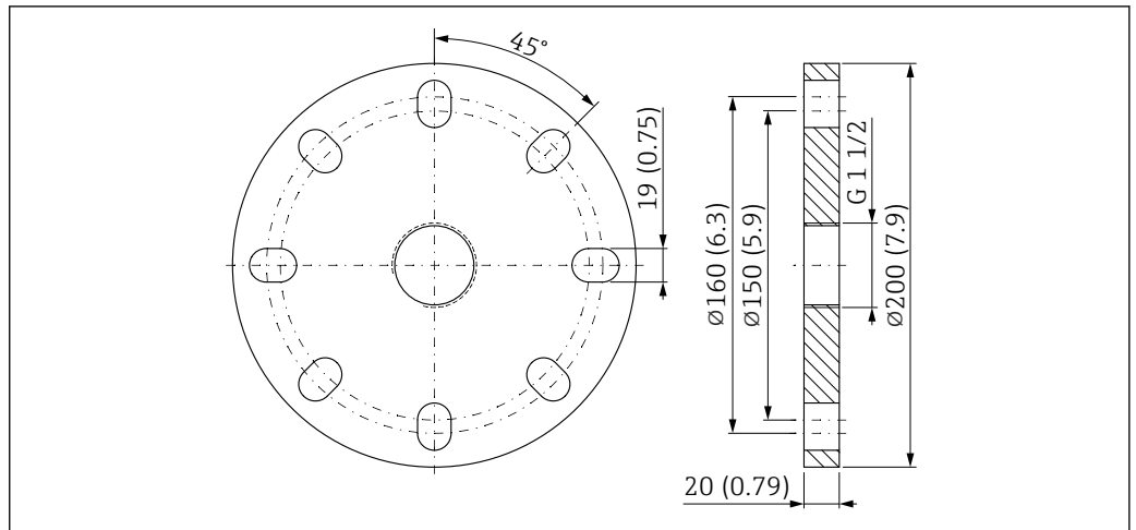
图 31 UNI 3"/DN80/80A 法兰的外形尺寸示意图。测量单位 mm (in)
