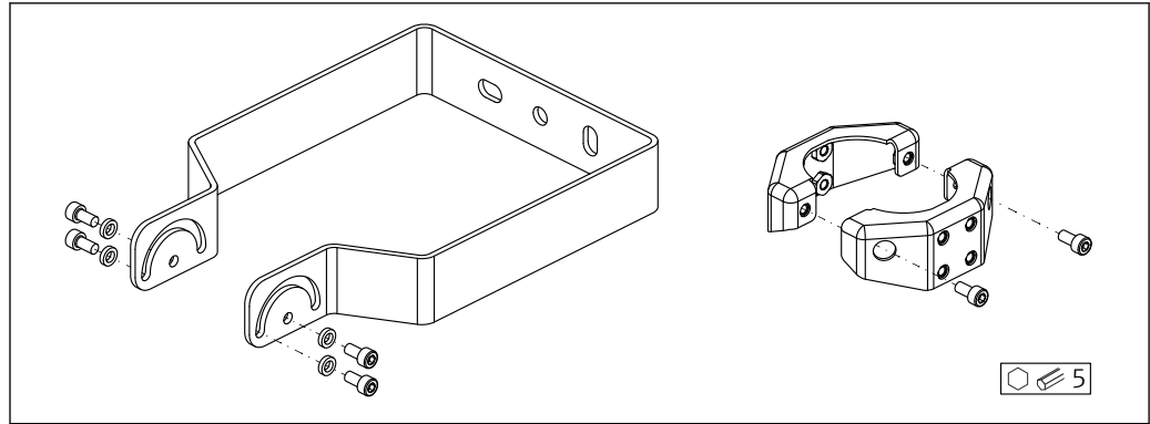
■ 21 安装架（可调节）的供货清单
