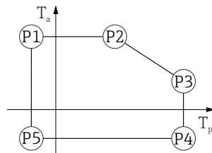
☐ 31 316L 外壳; 过程温度范围: -40 ... +80 °C (-40 ... +176 °F)
