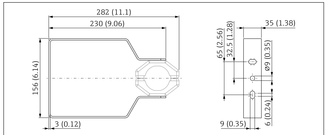
图 20 安装架的外形尺寸示意图。测量单位 mm (in)
