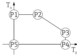
▣ 26 塑料外壳; 过程温度范围: 0 ... +80 °C (+32 ... +176 °F), 适用 CSA C/US 认证型仪表
