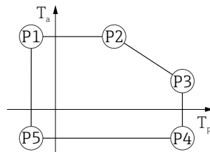
图 25 塑料外壳；过程温度范围：-40 ... +80 °C (-40 ... +176 °F)
