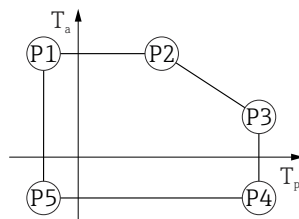
☑ 34 316L 外壳, 卫生型; 过程温度范围: -40 ... +130 °C (-40 ... +266 °F)
