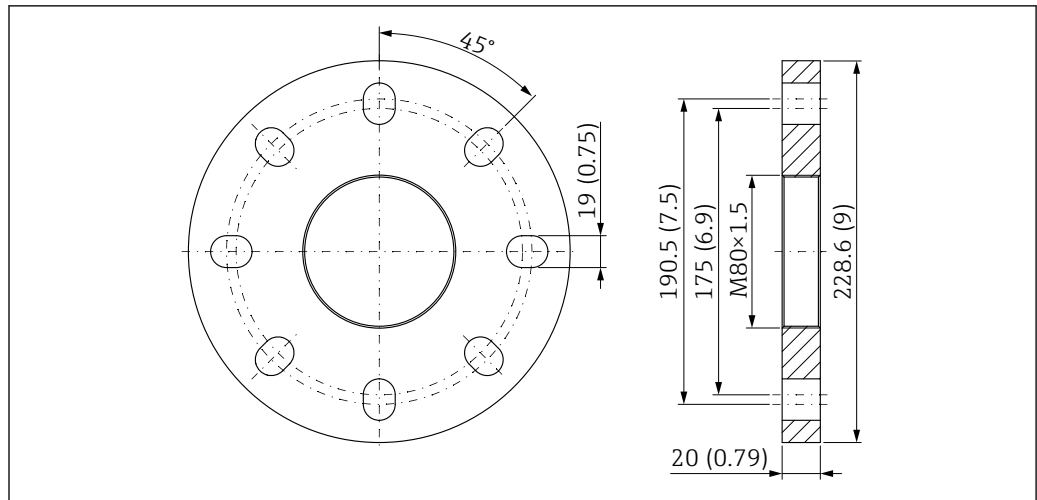
图 50 UNI 4"/DN100/100A 法兰，适用带空气吹扫接口的 PTFE 水滴型天线 (50 mm (2 in)口径)。测量单位 mm (in)
