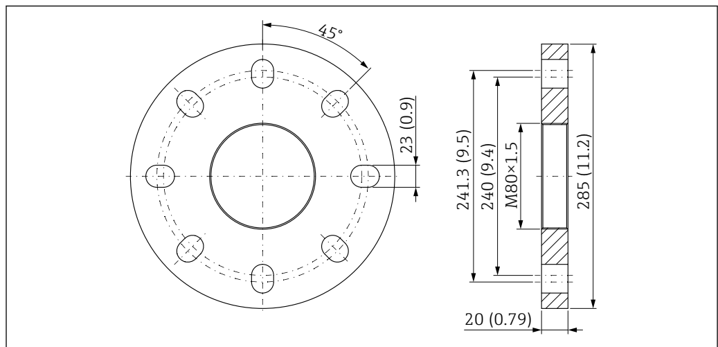
图 51 UNI 6"/DN150/150A 法兰，适用带空气吹扫接口的 PTFE 水滴型天线 (50 mm (2 in)口径)。测量单位 mm (in)
