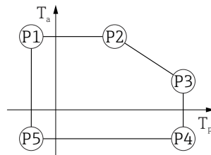
图 12 塑料外壳；过程温度范围：-40 ... +80 °C (-40 ... +176 °F)
