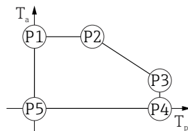
图 13 塑料外壳；过程温度范围：0 ... +80 °C (+32 ... +176 °F)，适用 CSA C/US 认证型仪表
