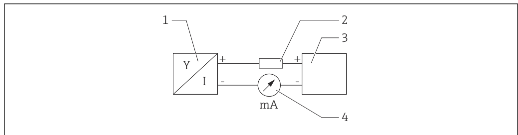
图 7 HART 信号回路连接框图
