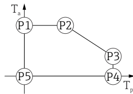
图 32 塑料外壳; 过程温度: 0 ... +280 °C (+32 ... +536 °F), 针对 CSA C/US 认证型仪表
