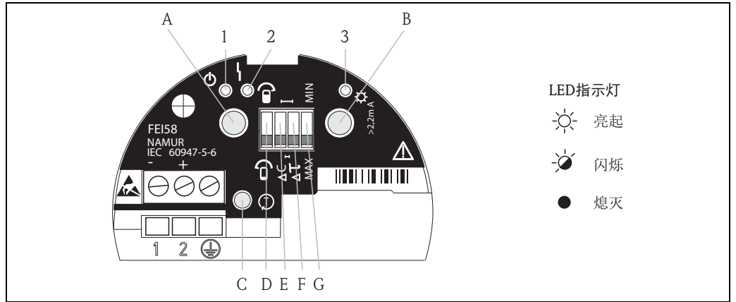
绿色 LED 指示灯 1 (☉: 可以操作); 红色 LED 指示灯 2 (⚡: 故障); 黄色 LED 指示灯 3 (⚡: 开关状态)
