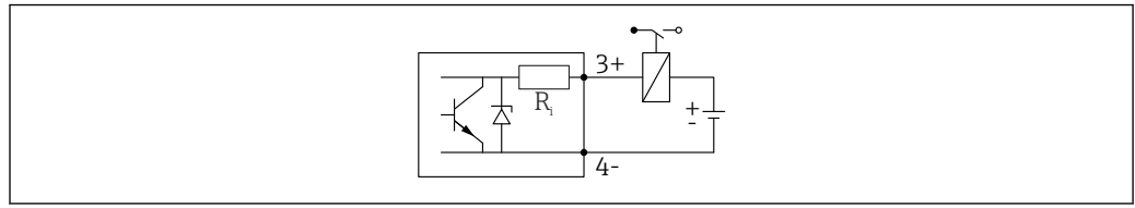
图 12 连接继电器
