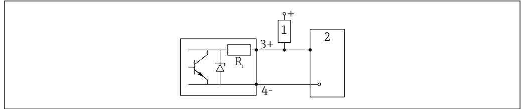
图 13 连接数字量输入
