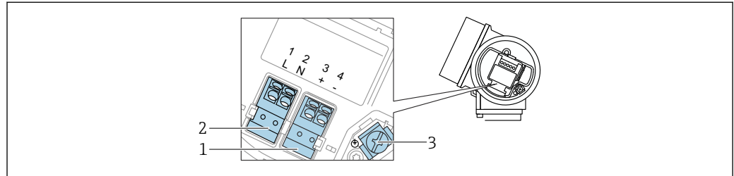
图 9 接线端子分配，四线制：4 ... 20 mA HART (90 ... 253 V AC )
