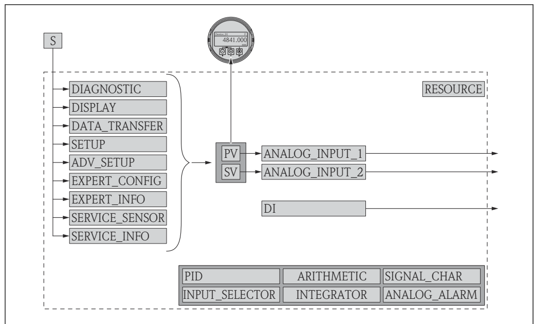
图 21 设备块的出厂设置
