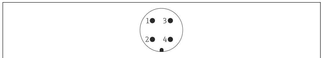
图 14 7/8"插头的针脚分配
