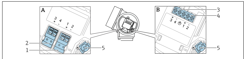
图 10 接线端子分配 PROFIBUS PA / FOUNDATION Fieldbus
