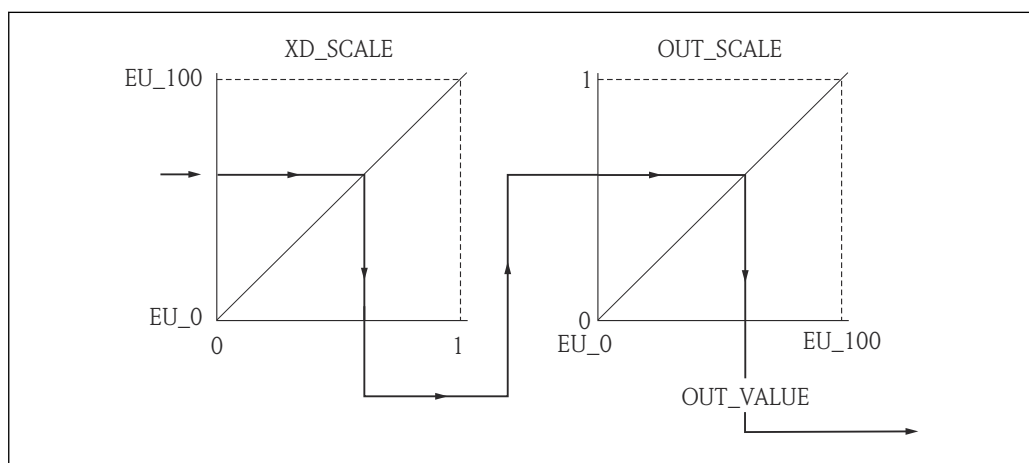
图 25 按比例转换 AI 块中的测量值
