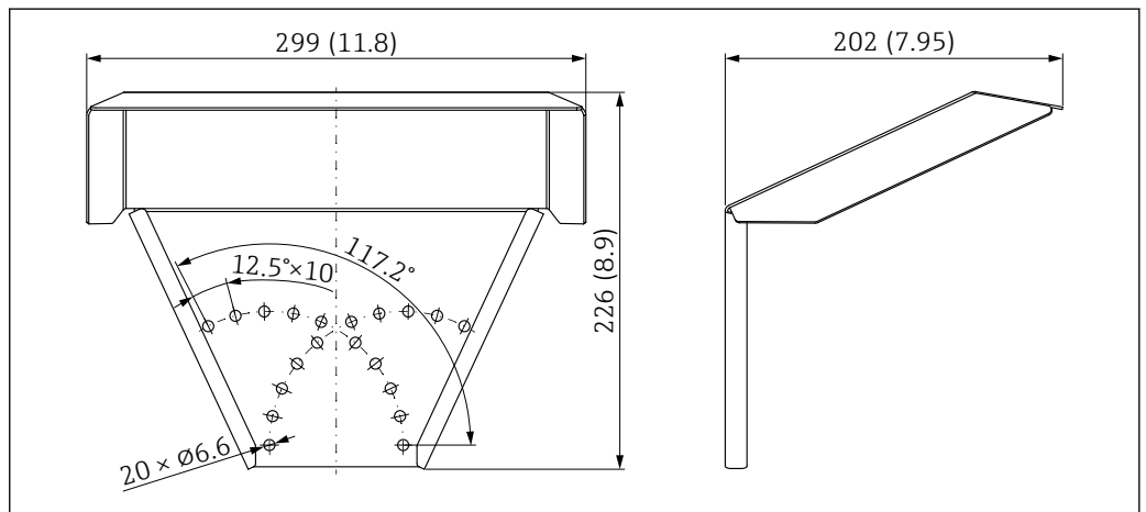
图 32 外形尺寸。测量单位 mm (in)
