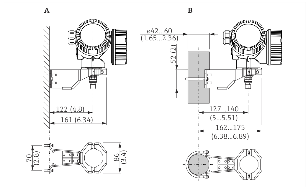
图 7 使用安装架安装电子腔外壳。测量单位 mm (in)
