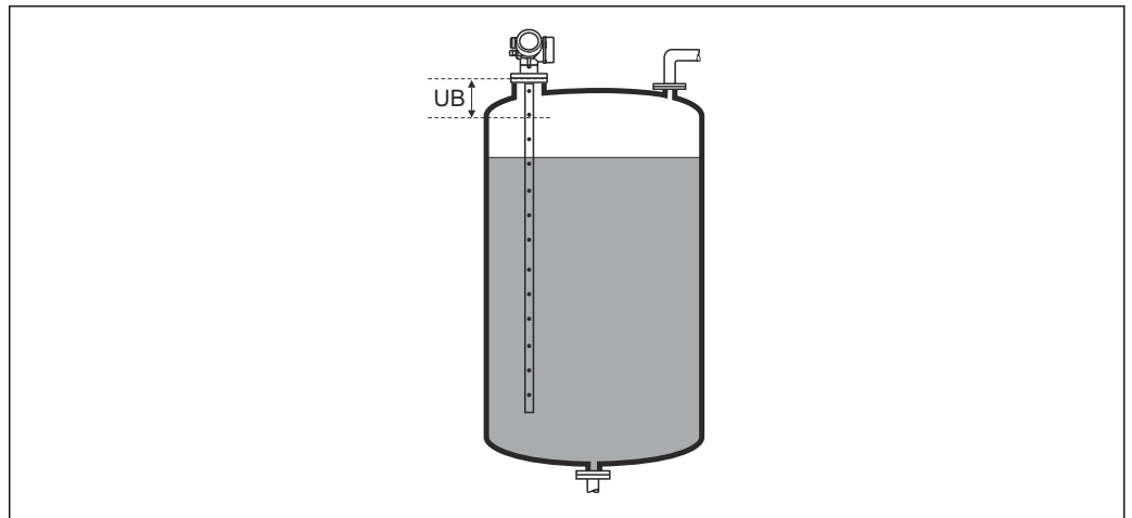
图 39 液位测量的盲区距离 (UB)
