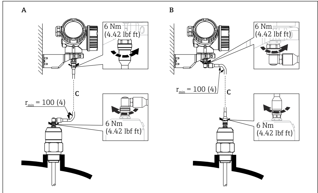
图 8 连接连接电缆。通过以下方式连接电缆：。测量单位 mm (in)
