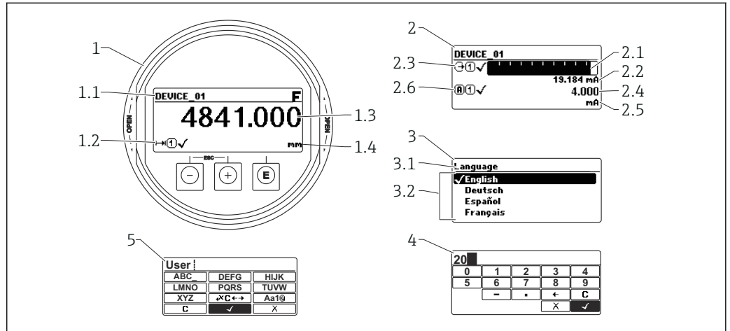
图 19 显示与操作单元的显示格式
