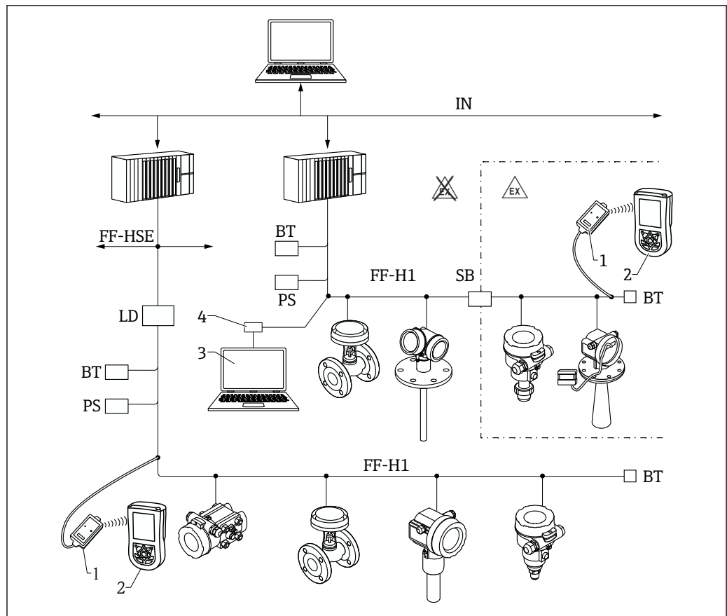
图 59 FOUNDATION Fieldbus 系统架构及其相关部件
