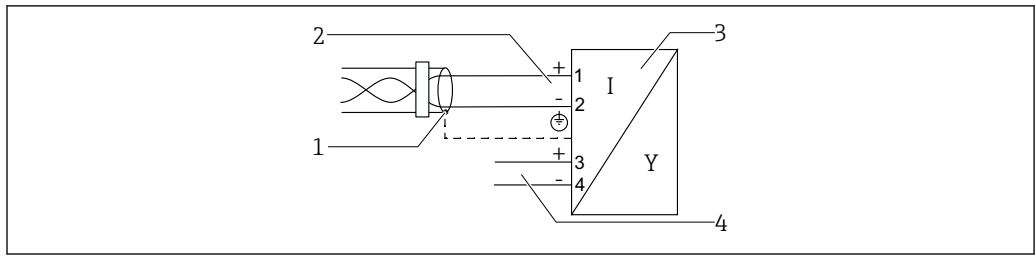
图 23 接线图: PROFIBUS PA / FOUNDATION Fieldbus
