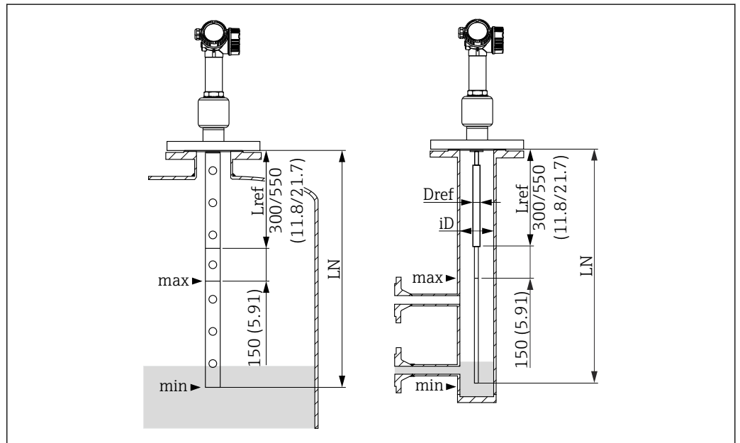
图 33 带气相补偿参考信号的 FMP54；单位：mm (in)
