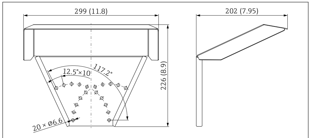
图 64 外形尺寸。测量单位 mm (in)
