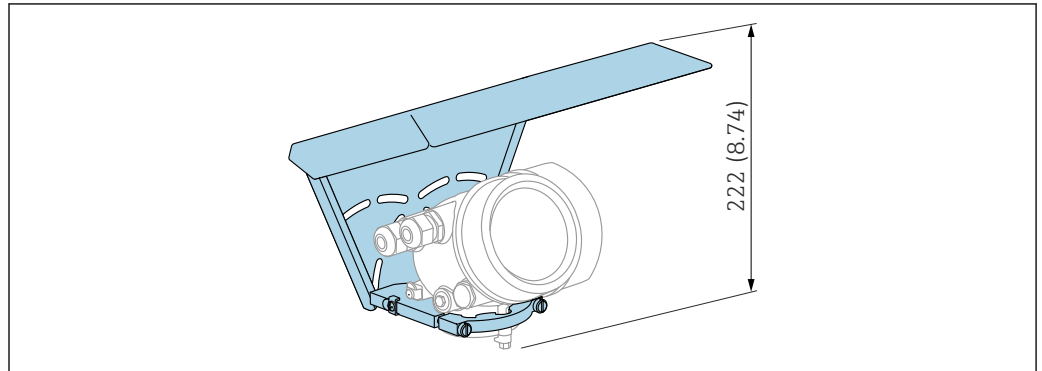
图 63 高度。测量单位 mm (in)
