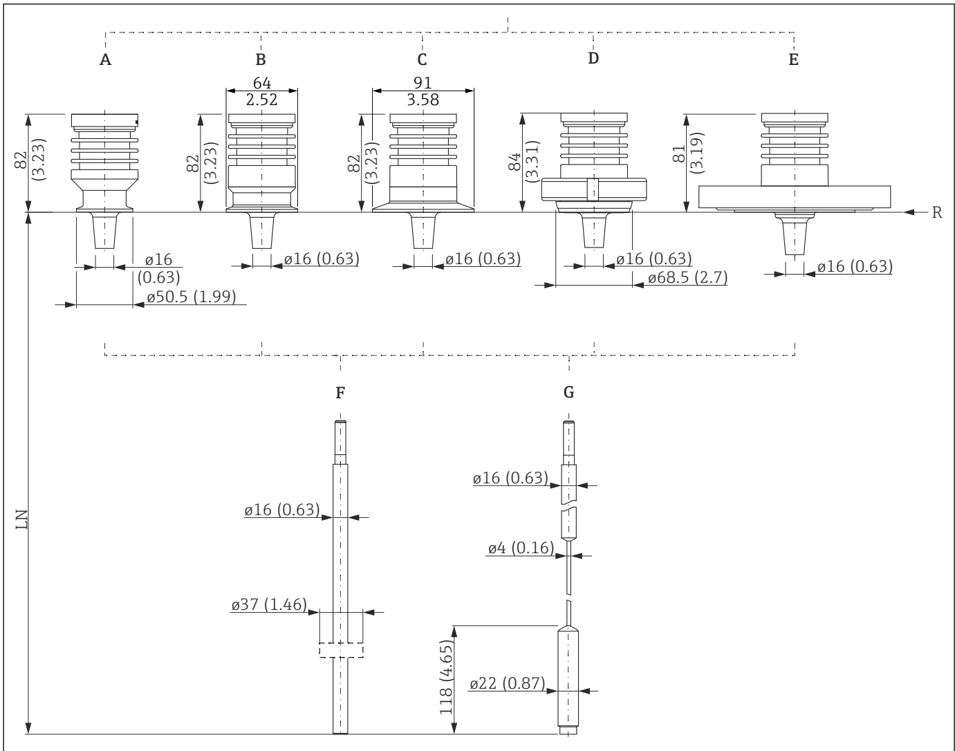
图 49 FMP52: 过程连接和探头。测量单位 mm (in)
