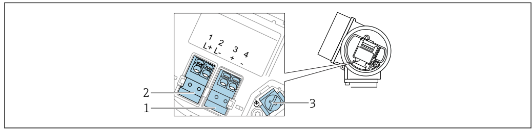
图 18 接线端子分配, 四线制: 4 ... 20 mA HART (10.4 ... 48 V DC )
