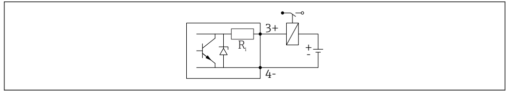
24 连接继电器
