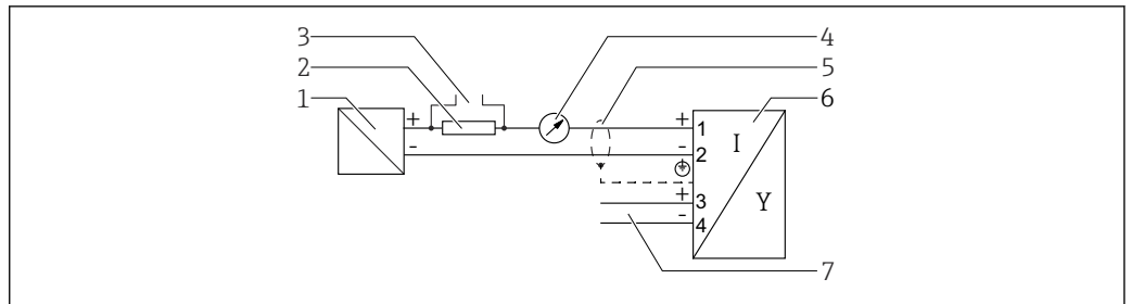
15 接线图：两线制：4 ... 20 mA HART，开关量输出
