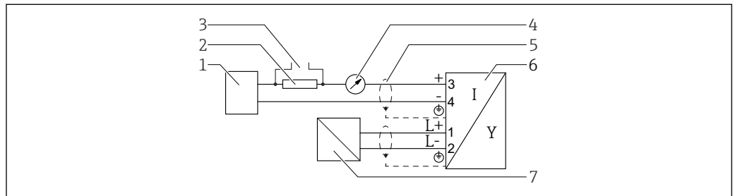
图 19 接线图: 四线制: 4 ... 20 mA HART (10.4 ... 48 V DC )
