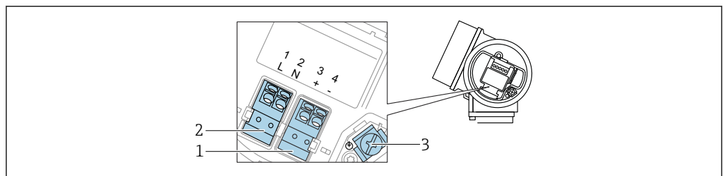
图 20 接线端子分配, 四线制: 4 ... 20 mA HART (90 ... 253 V AC )
