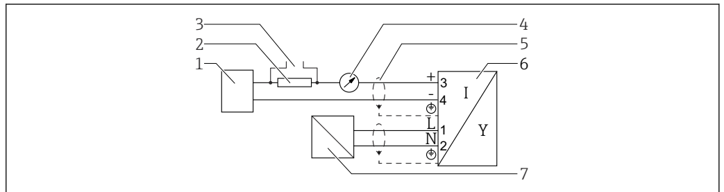
21 接线图: 四线制: 4 ... 20 mA HART (90 ... 253 V AC )
