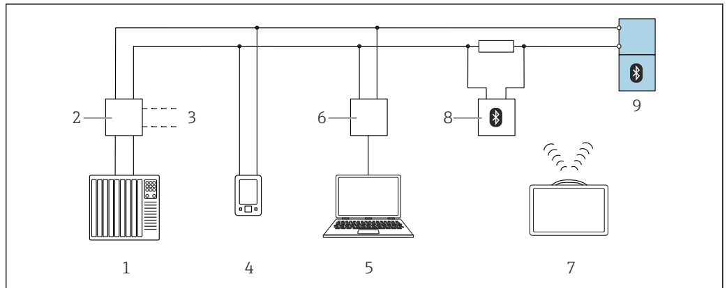
图 58 通过 HART 通信实现远程操作
