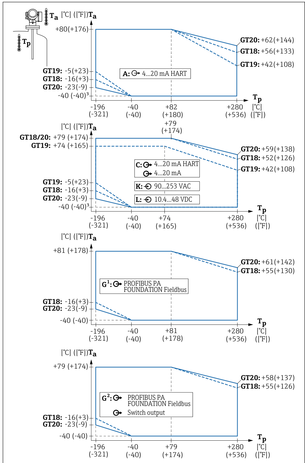
温度曲线: FMP54, 增温型 (XT), 最高+280 °C (+536 °F)
