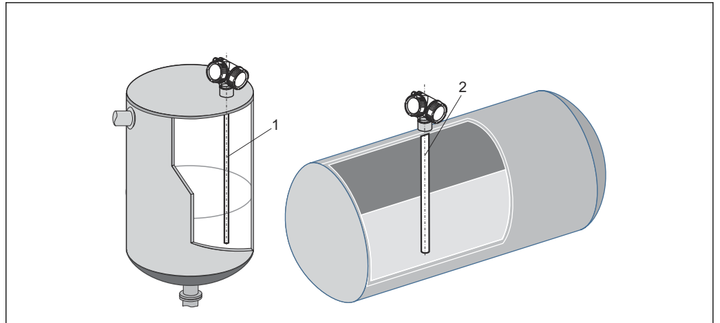
1 同轴探头
