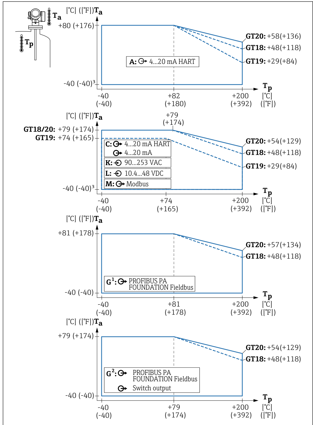
温度曲线: FMP51, 带 G \frac{3}{4} 或 NPT \frac{3}{4} 螺纹连接
