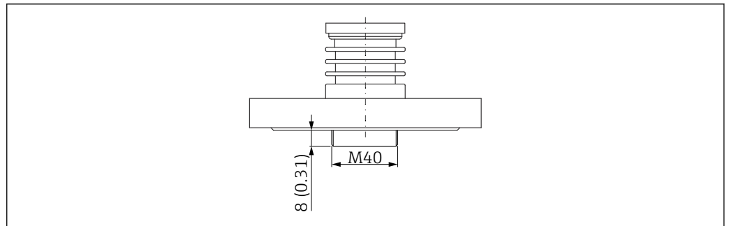
48 AlloyC 材质法兰的外形尺寸。测量单位 mm (in)
