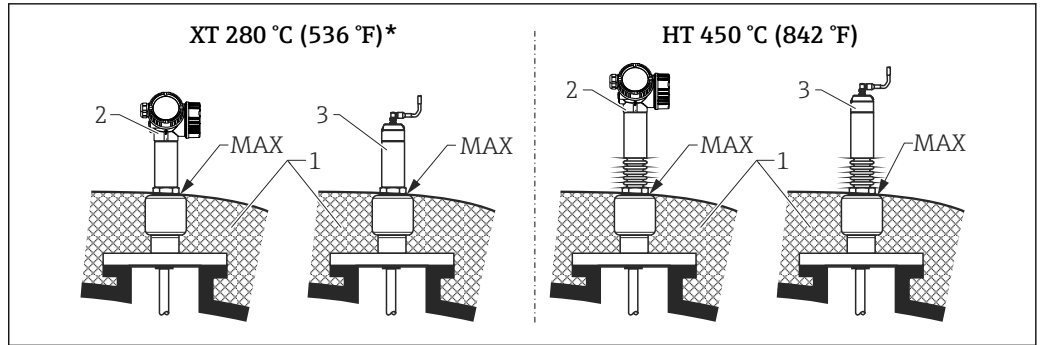
图 40 法兰过程连接 - 增温型 (XT) 和高温型 (HT) 仪表
