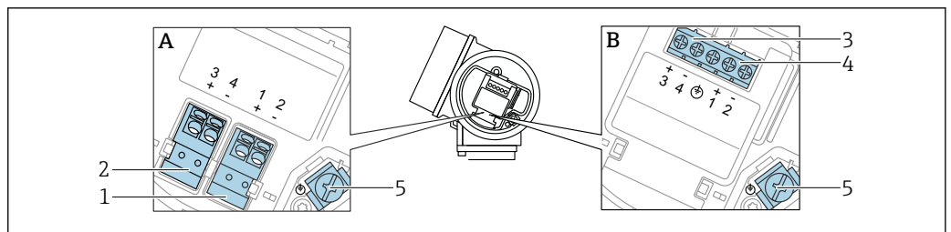
16 接线端子分配，两线制：4 ... 20 mA HART，4 ... 20 mA
