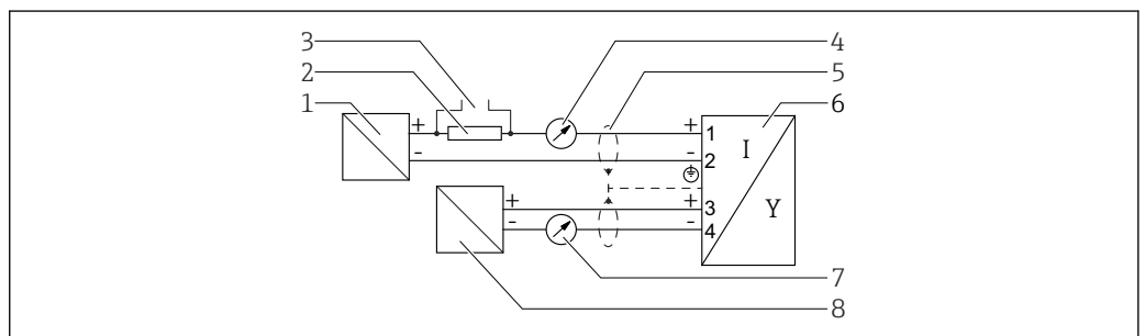
17 接线图：两线制：4 ... 20 mA HART，4 ... 20 mA
