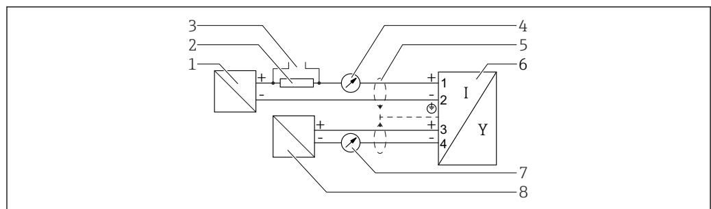
图 12 接线图：两线制：4 ... 20 mA HART，4 ... 20 mA
