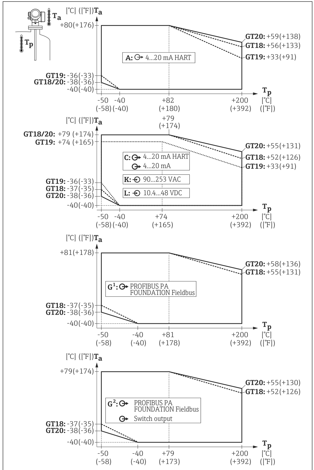
温度曲线: FMP55
