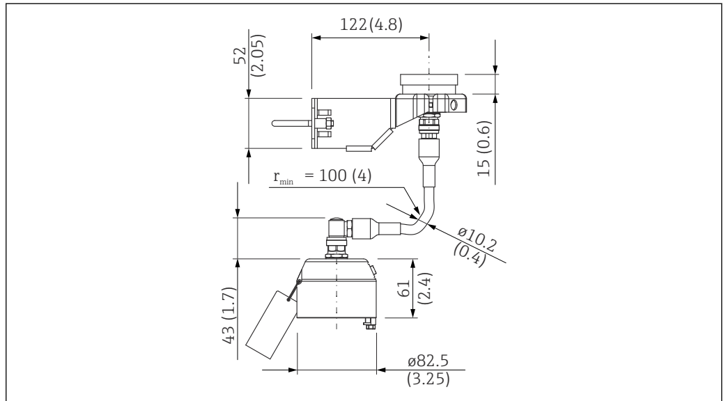
图 33 分体式探头的连接尺寸；连接电缆长度为订购长度。测量单位 mm (in)
