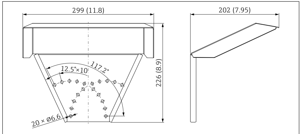
图 48 外形尺寸。测量单位 mm (in)
