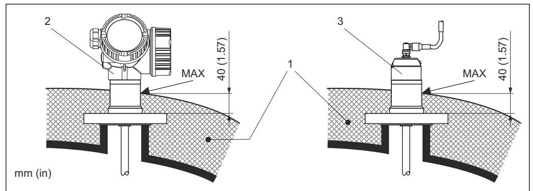
28 法兰过程连接
