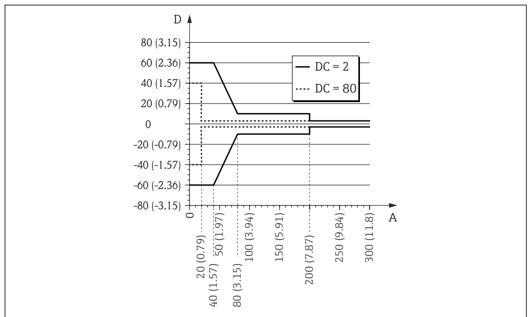
图 24 杆式探头和同轴探头底部附近的测量误差
