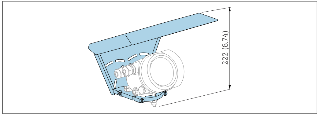
图 47 高度。测量单位 mm (in)
