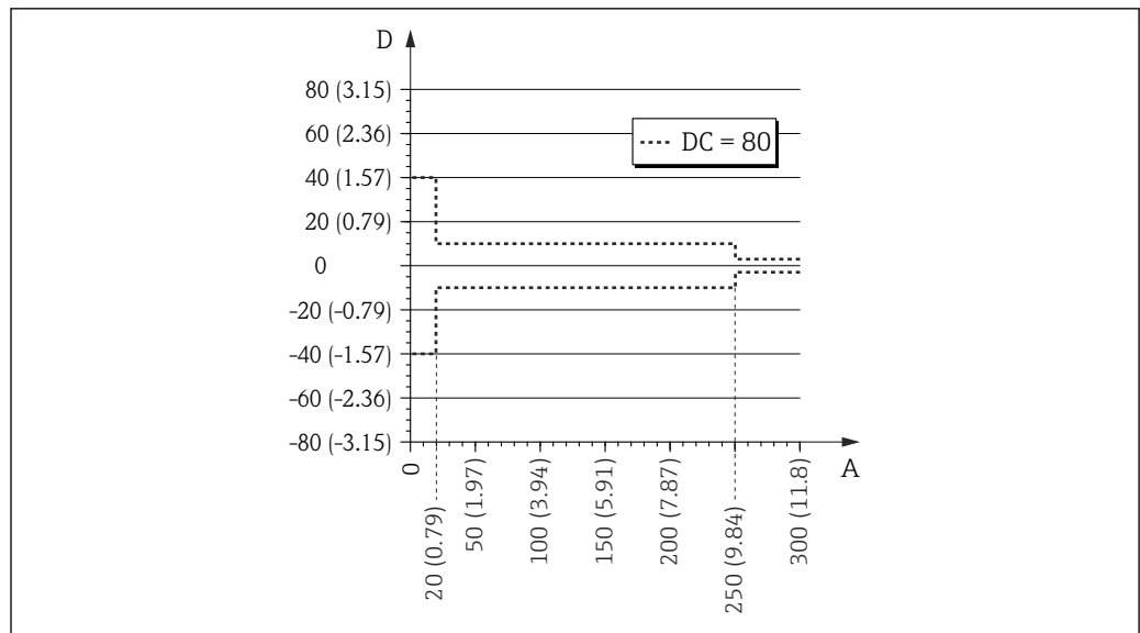
25 缆式探头底部的测量误差
