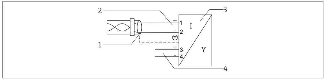
18 接线图: PROFIBUS PA / FOUNDATION Fieldbus
