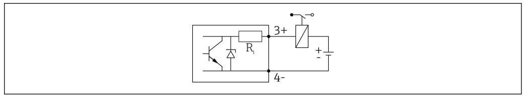
14 连接继电器
