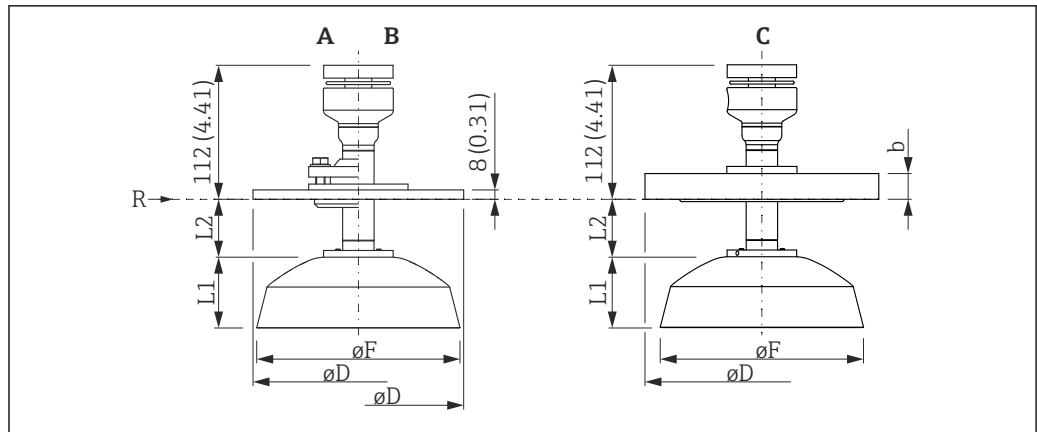
图 38 带抛物面天线的 FMR57 的外形尺寸示意图；单位：mm (in)
