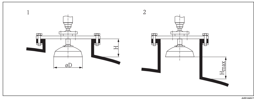
图 9 带抛物面天线的 Micropilot 的安装短管安装示意图
