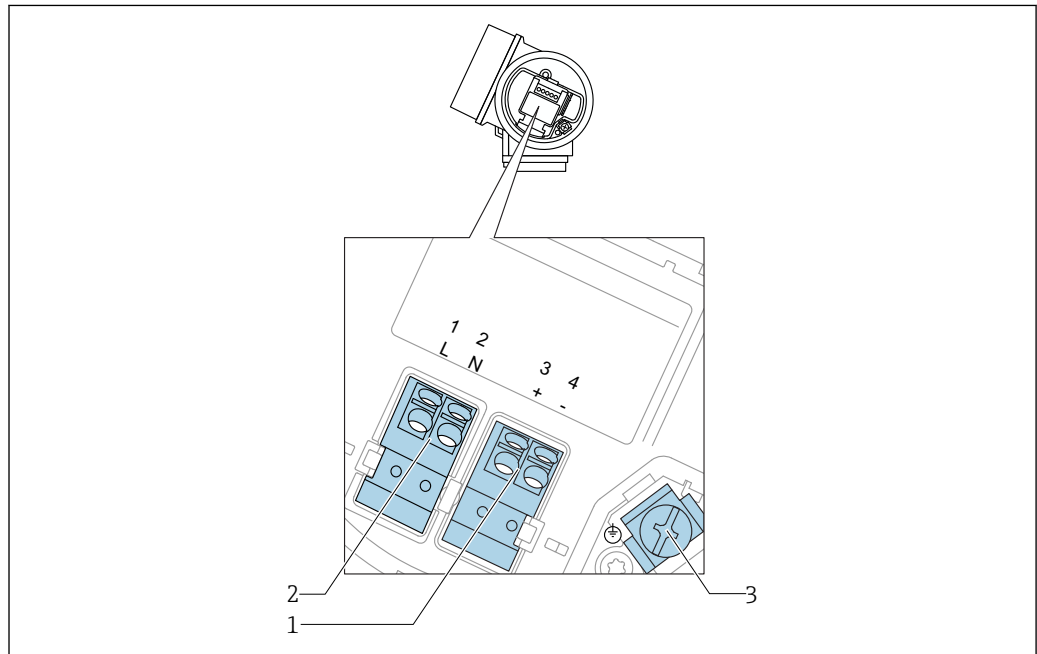
图 20 接线端子分配：四线制；4...20 mA HART (90 ... 253 V AC )
