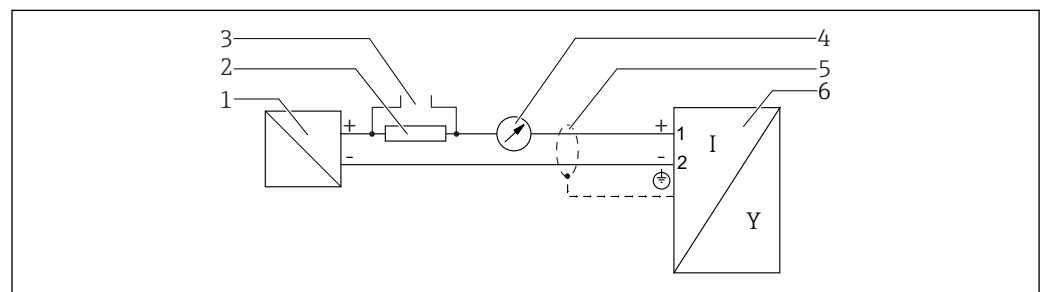
图 13 接线图：两线制；4...20 mA HART
