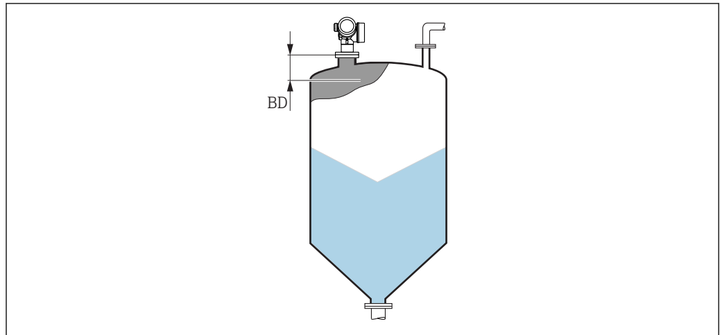
图 55 固体测量时的盲区距离 (BD)
