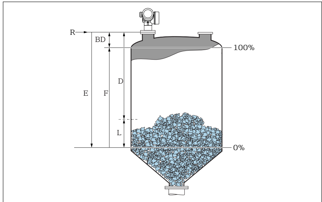
图 41 料位测量的设置参数
