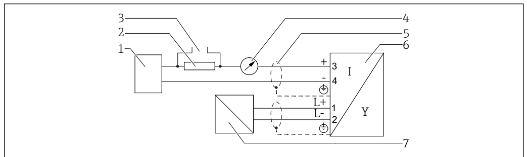
19 接线端子分配: 四线制; 4...20 mA HART (10.4 ... 48 V DC )
