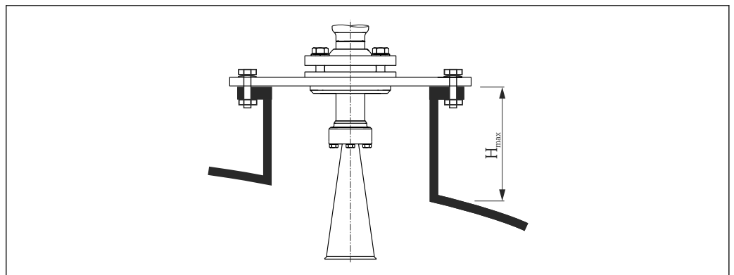
图 8 喇叭天线的安装短管高度 (FMR57)
