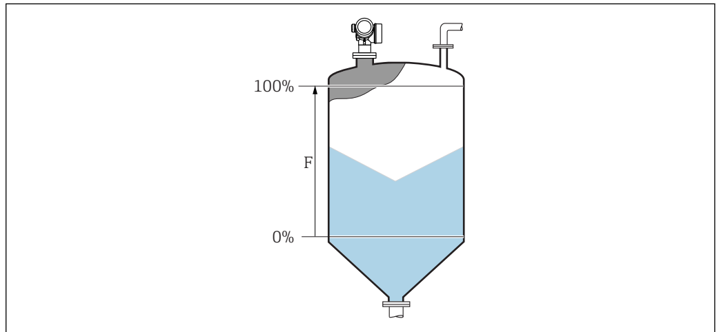
48 料位测量时的满标 (F)
