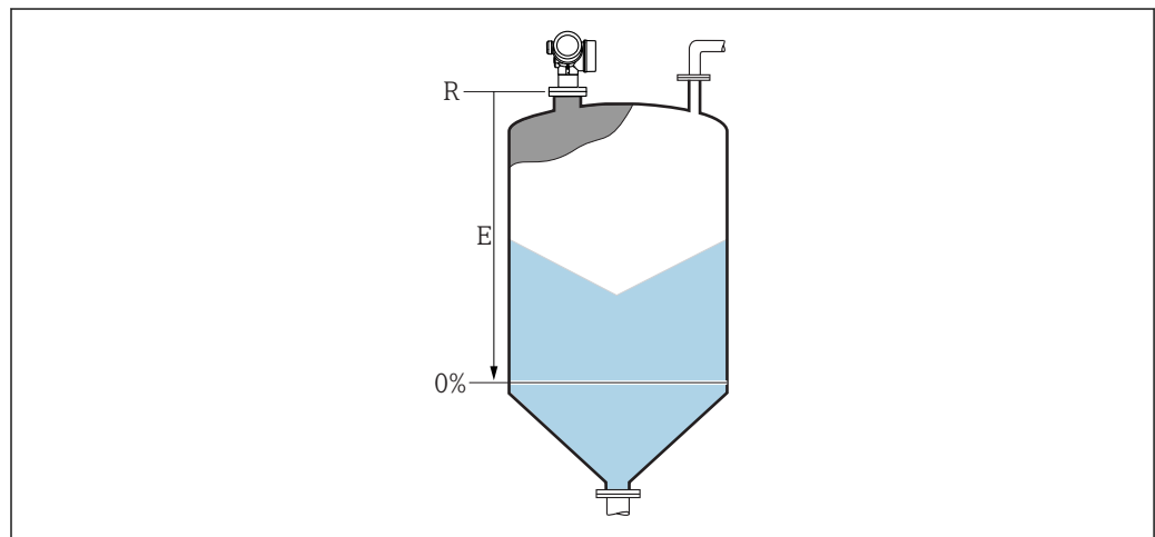
☑ 47 料位测量时的空标 (E)
