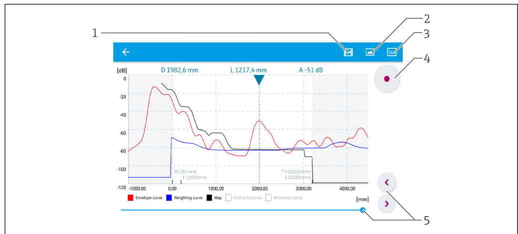
图 38 在 SmartBlue 中显示包络线； Android 视图
