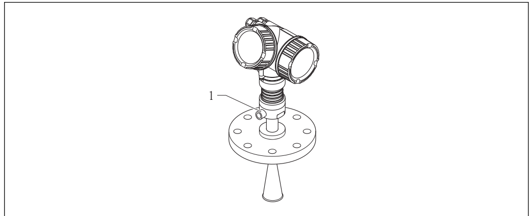
图 11 带空气吹扫接口的 Micropilot FMR57
