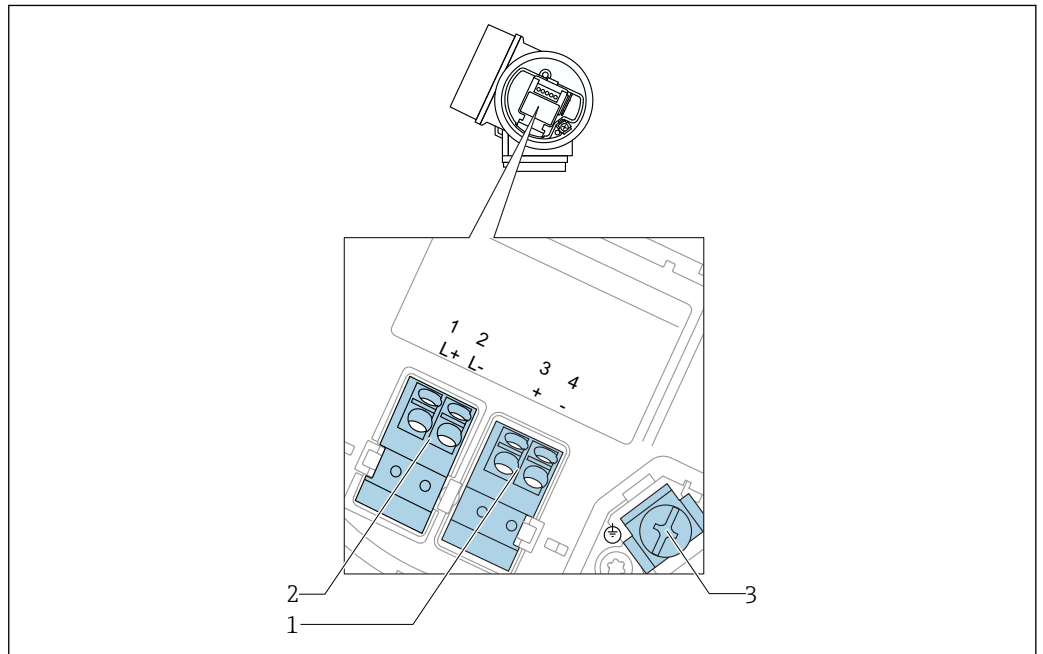
18 接线端子分配: 四线制; 4...20 mA HART (10.4 ... 48 V DC )
