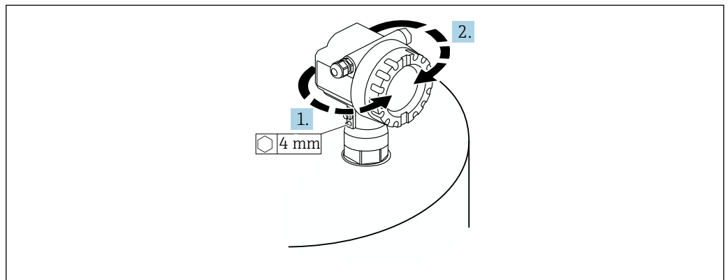
图 13 旋转 F12 或 T12 外壳（实例：F12 外壳）
