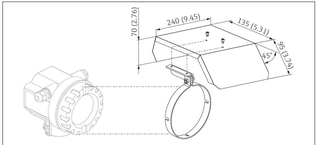
图 31 F12 或 T12 外壳防护罩。测量单位 mm (in)
