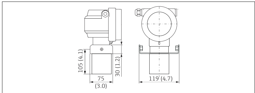
19 外形尺寸，带安装架。测量单位 mm (in)
