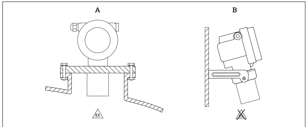
图 12 安装实例
