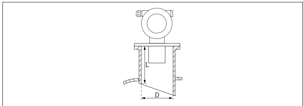
图 15 短管长度 L 与短管直径 D 示意图
