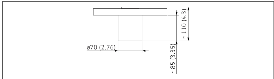
18 传感器外形尺寸。测量单位 mm (in)
