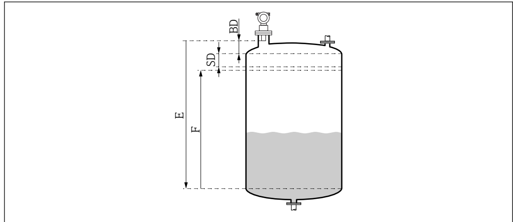
图 14 正常设备操作参数
