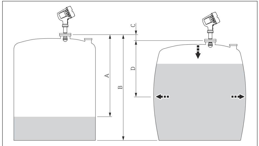
图 36 静压式储罐变形校正 (HyTD)
