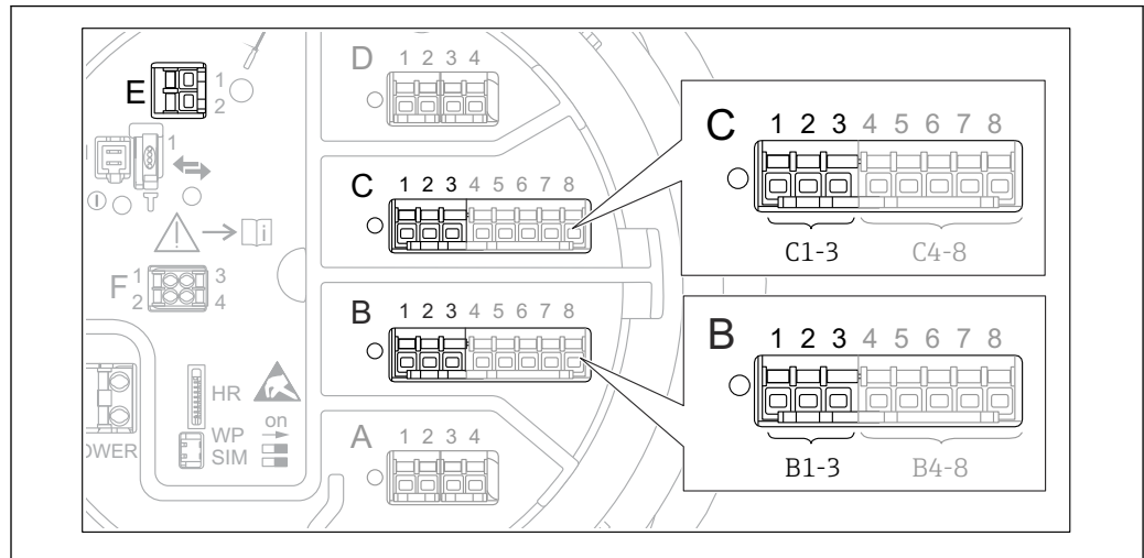
图 28 HART 回路的可能接线端子
