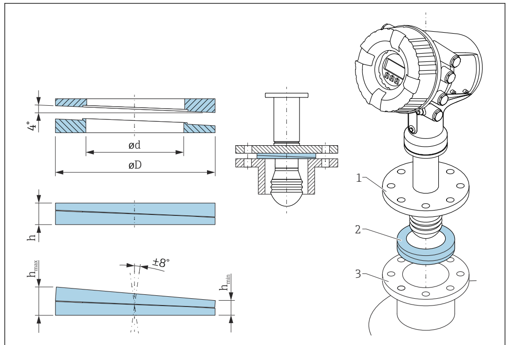
图 48 可调角度密封圈用于调节天线位置，角度调节范围为±8°
