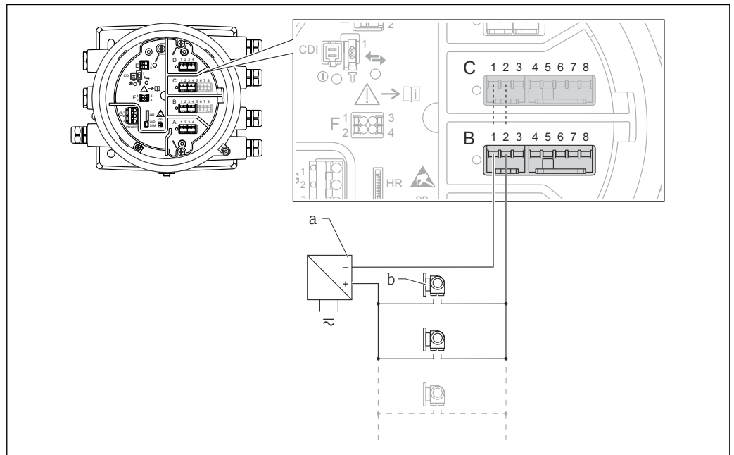
图 12 HART 主站模式下的无源模拟量输入/输出模块
