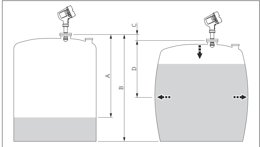
图 34 静压式储罐变形校正 (HyTD)
