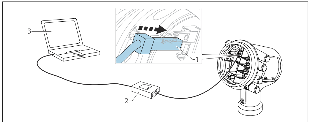
图 23 通过服务接口操作
