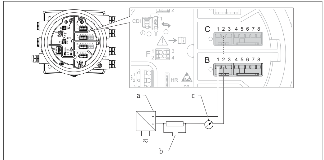
图 8 输出模式下的无源模拟量输入/输出模块
