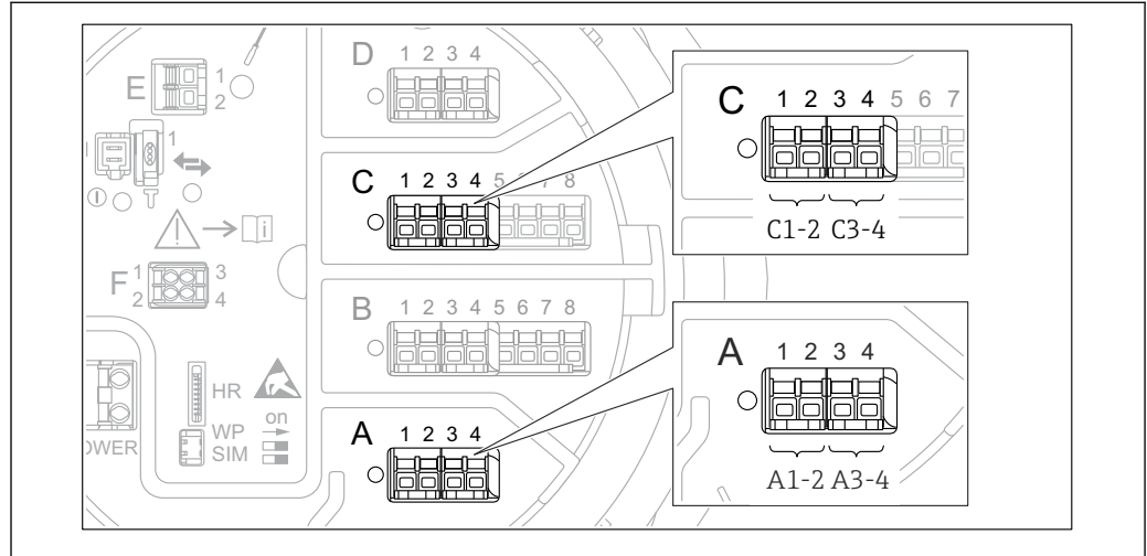
图 48 数字量输入或输出的名称 (实例)
