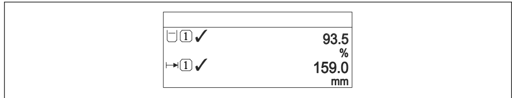
图 61 “显示格式” = “2 个数值”
