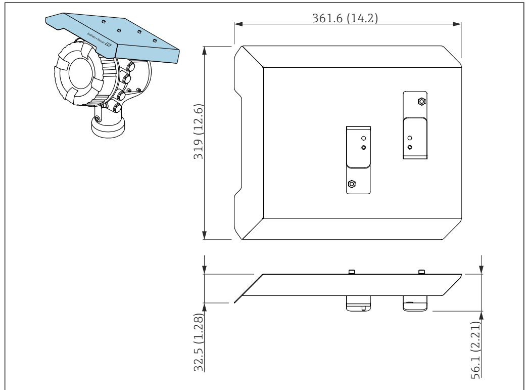
图 45 防护罩的外形尺寸示意图；单位：mm (in)
