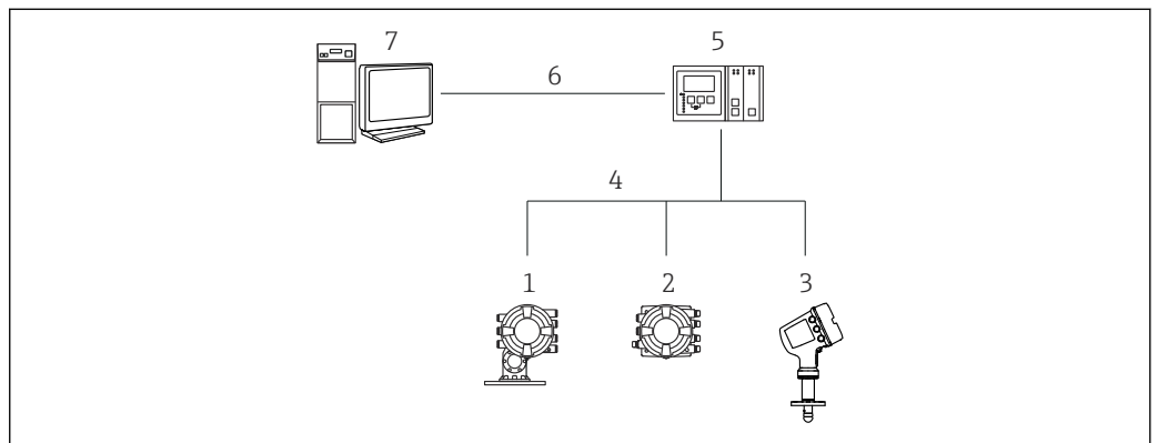
图 24 通过 Tankvision 储罐扫描仪 NXA820 连接雷达液位测量设备至 FieldCare
