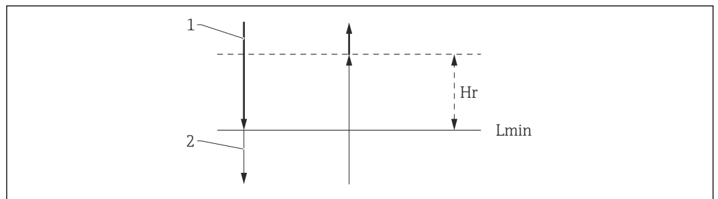
图 56 HTMS 单点回差控制范围
