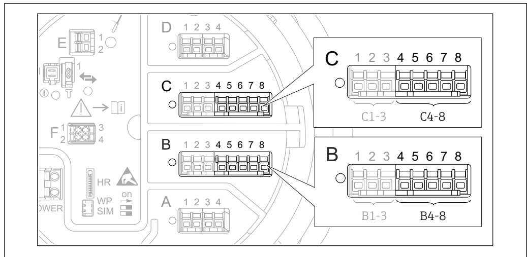
图 31 已连接 RTD 的模拟量输入/输出模块的可能安装位置。设备的订货号确定当前使用的模块 → 图 18。
