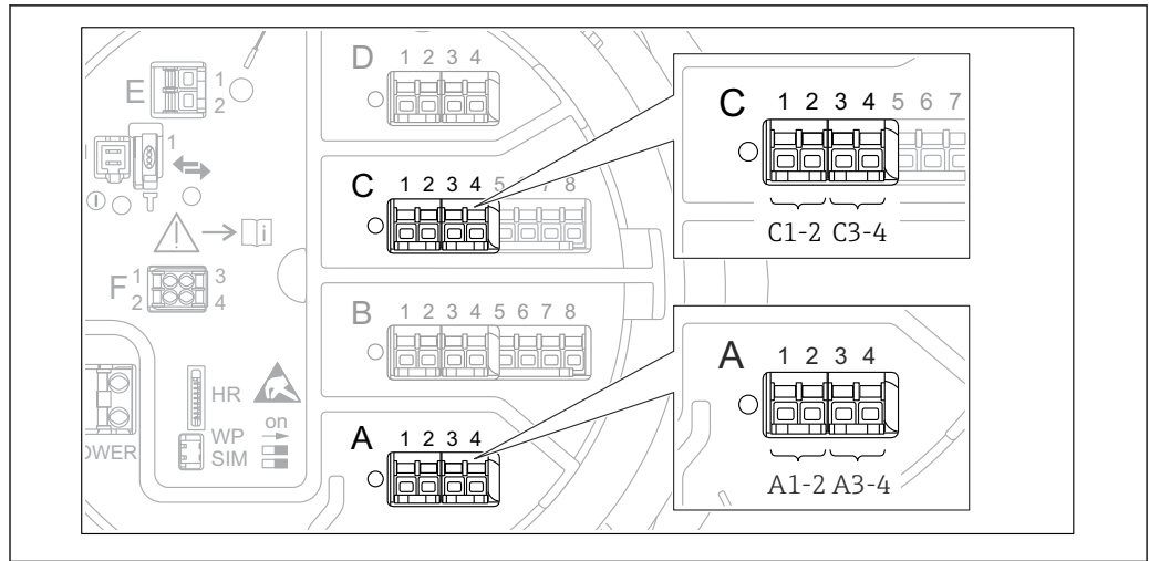
图 33 数字量输入/输出模块的可能安装位置 (示例)；订货号确定数字量输入模块的数量和位置→ 18。
