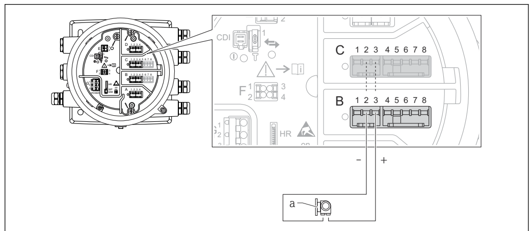
图 12 输入模式下的有源模拟量输入/输出模块
