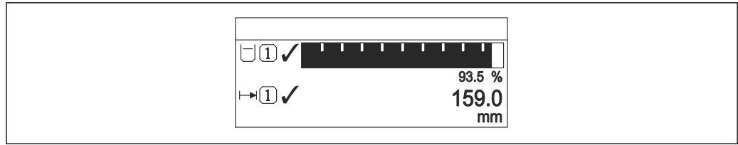
图 60 “显示格式” = “1 个棒图+1 个数值”
