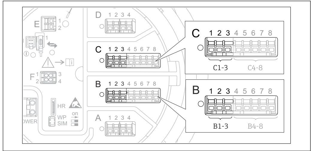
图 47 “Analog I/O”子菜单的接线端子（分别为“B1-3”或“C1-3”）
