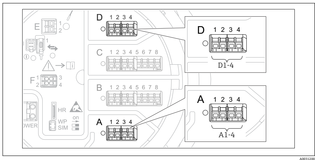
图 41 WM550 模块的可能安装位置（实例）；取决于设备型号，上述模块还可以安装在插槽 B 或 C 中 → 图 18。
