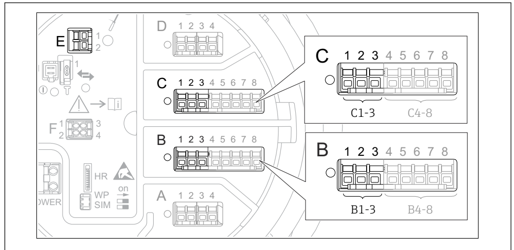
图 26 HART 回路的可能接线端子
