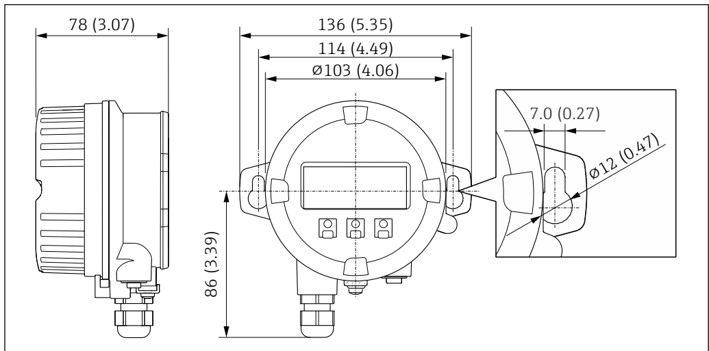
图 25 单位: mm (in)
