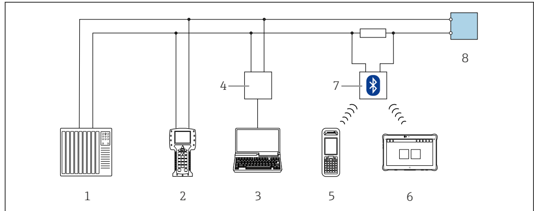
图 31 通过 HART 通信进行远程操作（有源信号）
