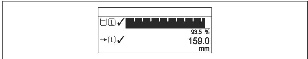
图 54 “显示格式” = “1 个棒图+1 个数值”
