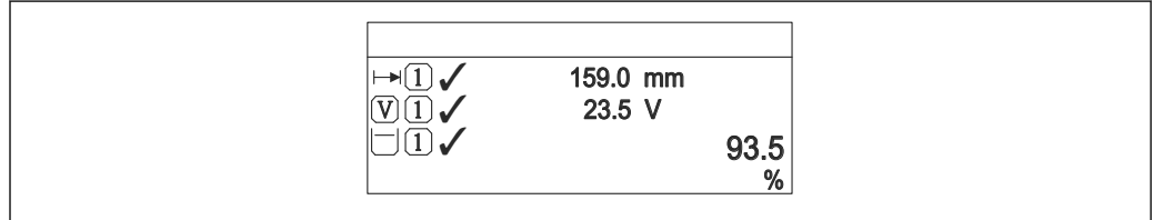
图 56 “显示格式” = “1 个数值(大)+2 个数值”
