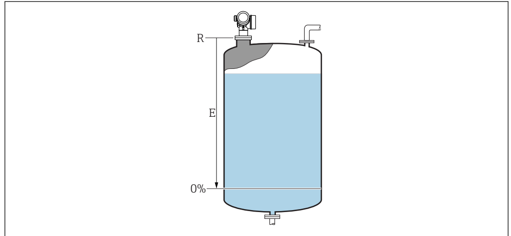
图 44 液位测量时的空标 (E)
