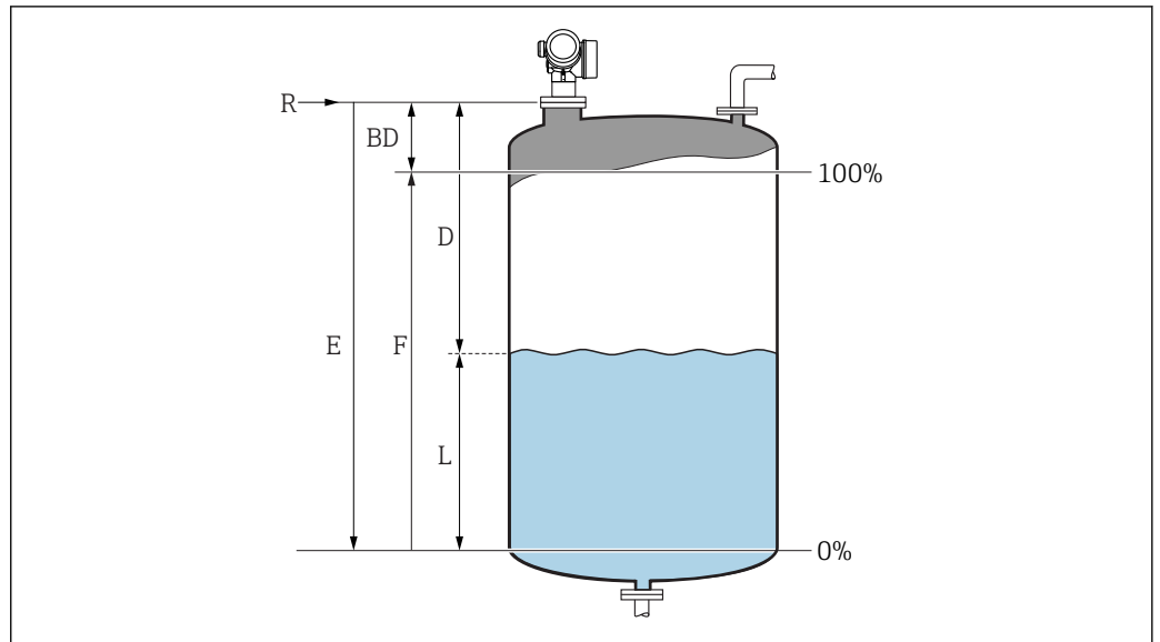
图 39 液位测量的设置参数
