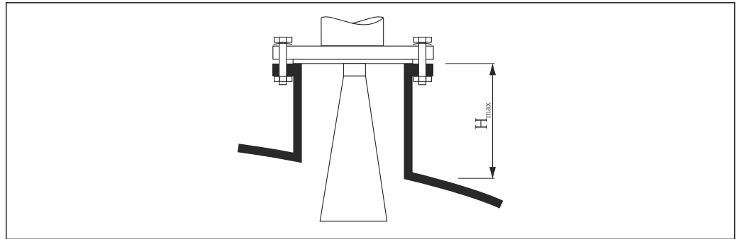
图 6 喇叭天线的安装短管高度 (FMR51) 示意图
