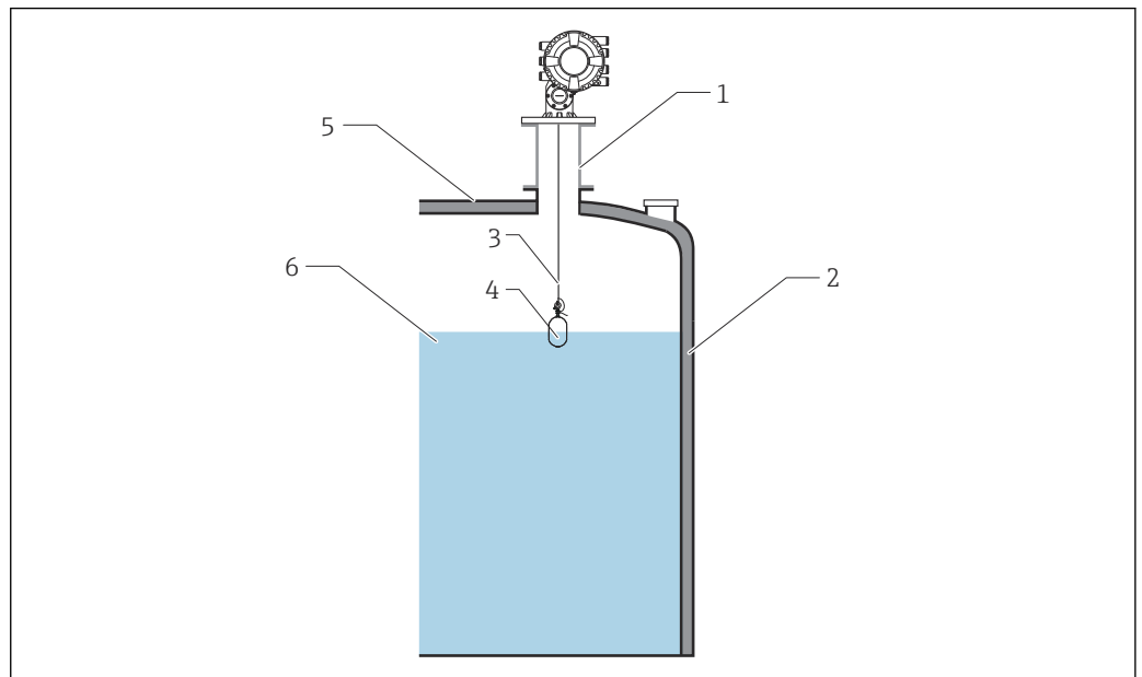
18 过程密封
