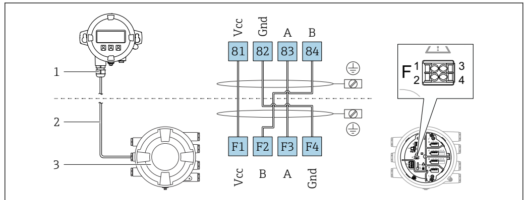
图 13 分离型显示与操作单元 DKX001 连接至罐旁指示仪 (NMR8x、NMS8x 或 NRF8x)
