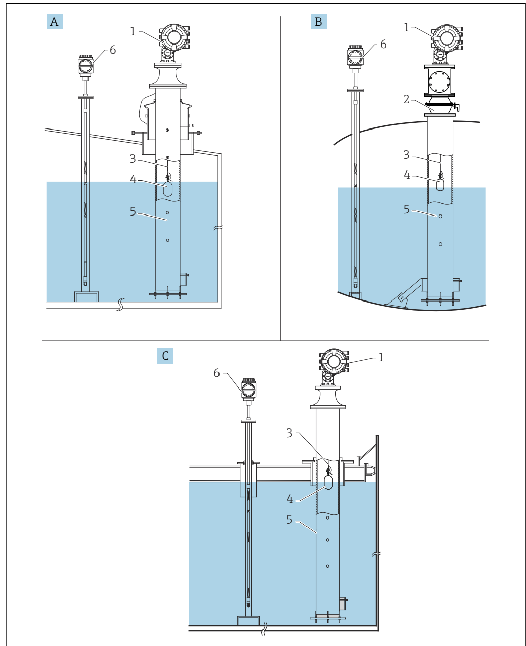
图 5 典型罐体安装方式示意图
