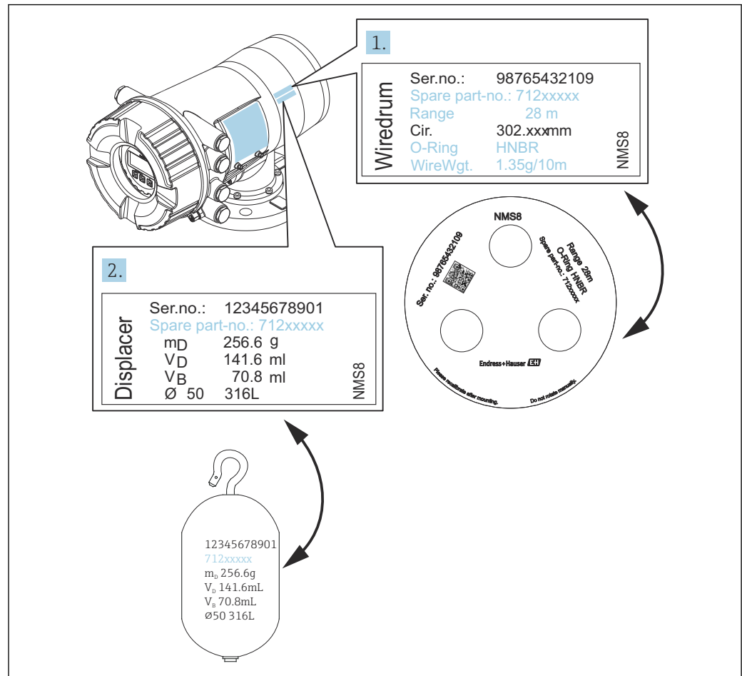
14 验证浮子和轮鼓
