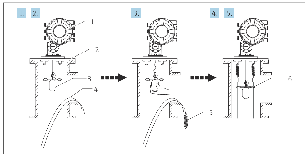
11 安装导向钢丝
