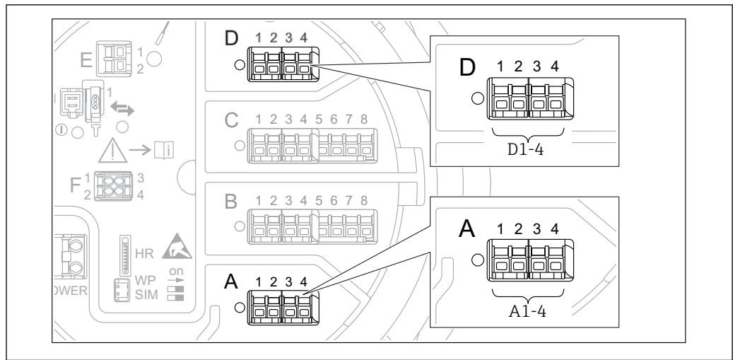
图 71 Modbus 模块的可能安装位置示例；取决于仪表型号，上述模块可以安装在插槽 B 或 C 中 → 45。
