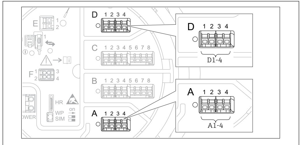
图 92 “Modbus”、“V1”或“WM550”模块名称实例；取决于设备型号，上述模块可以安装在插槽 B 或插槽 C 中。
