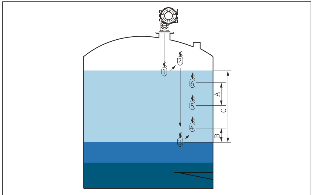
图 56 界面梯度位移（数字显示浮子的移动顺序）示意图
