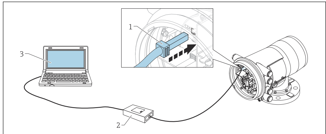
图 39 通过服务接口操作
