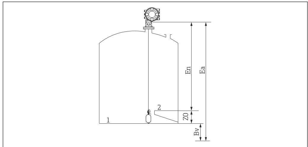
图 50 敞开式无液体储罐
