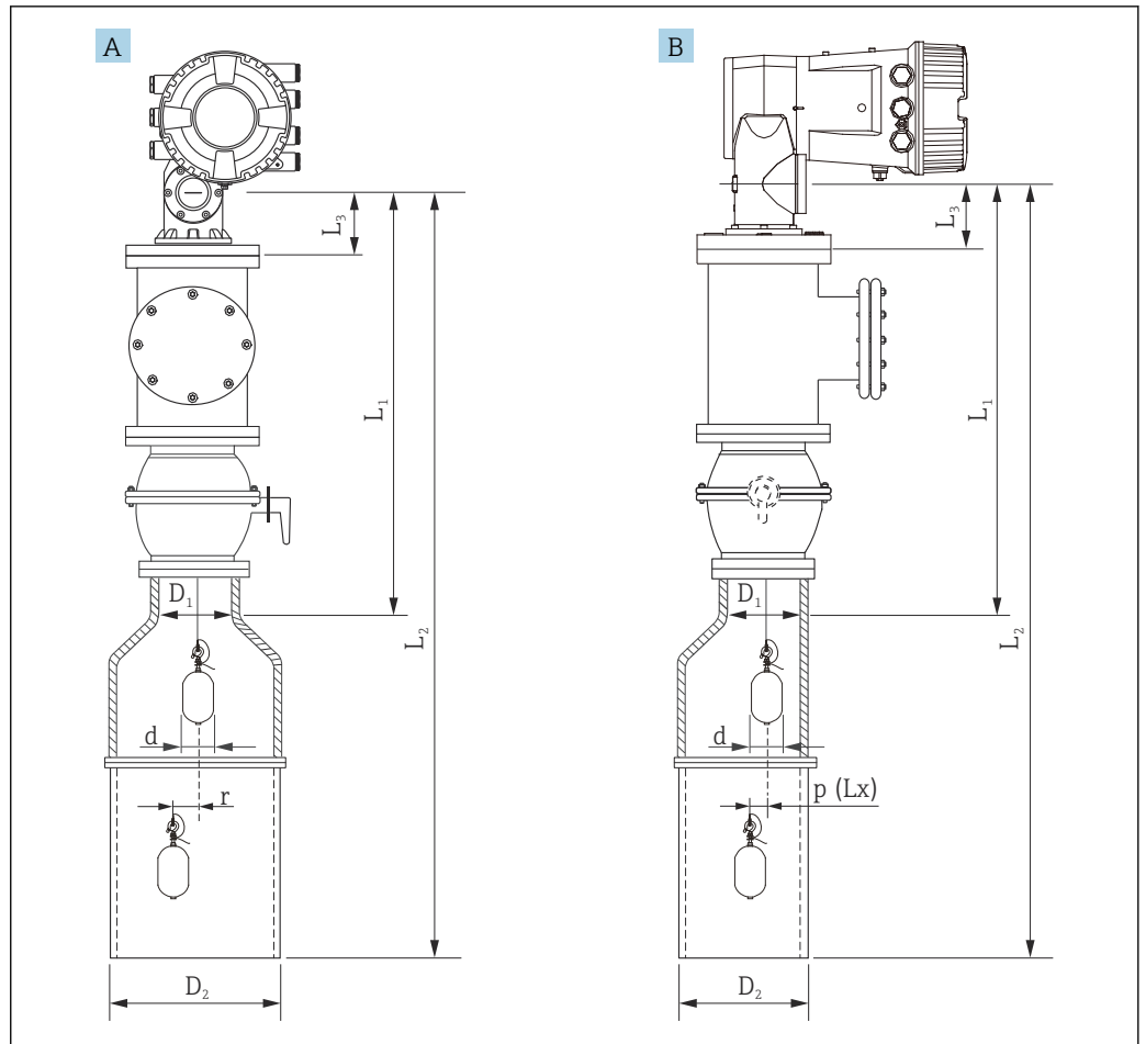
8 非对中导波管的安装示意图
