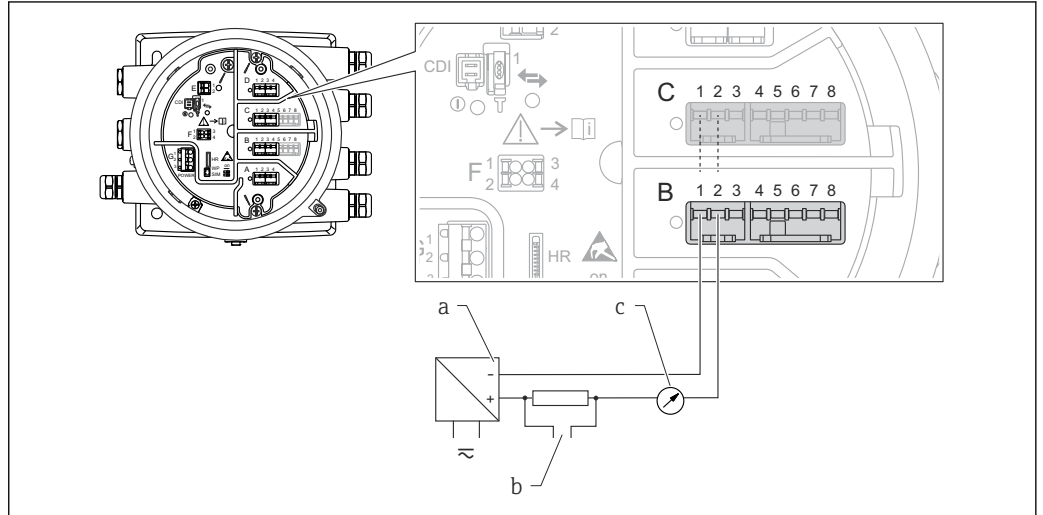
图 22 输出模式下的无源模拟量输入/输出模块
