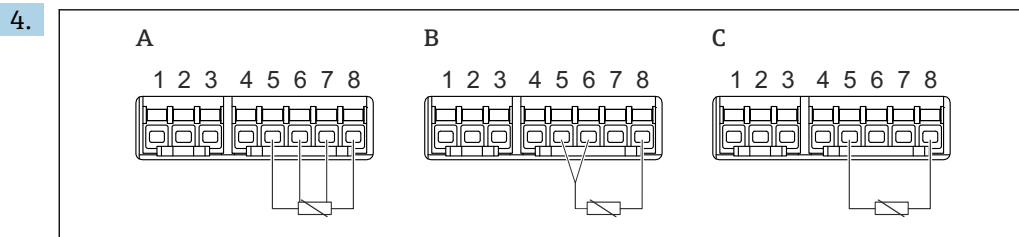
图 64 热电阻连接方式
