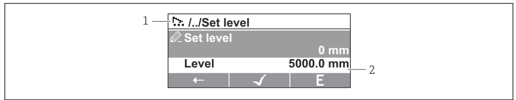
图 32 显示单元上的设置向导界面
