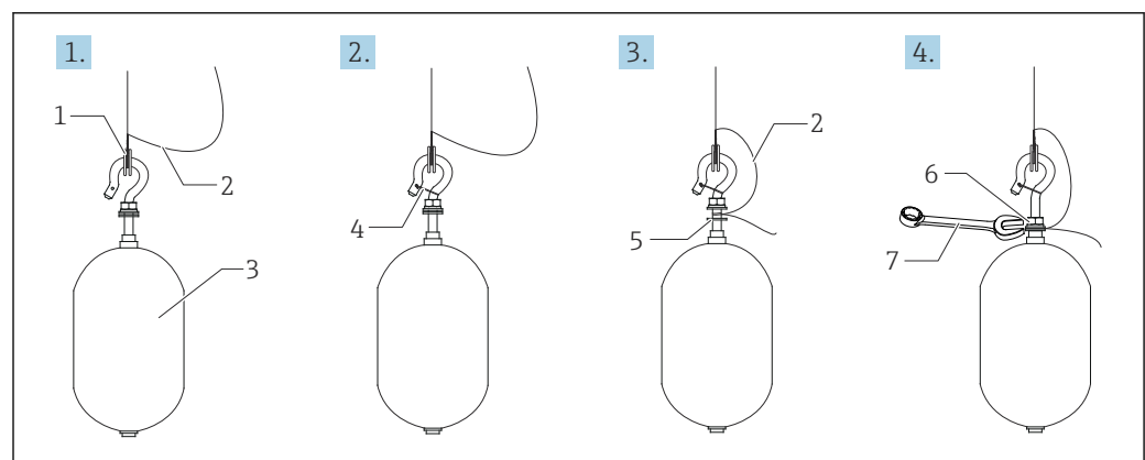
图 16 浮子安装示意图
