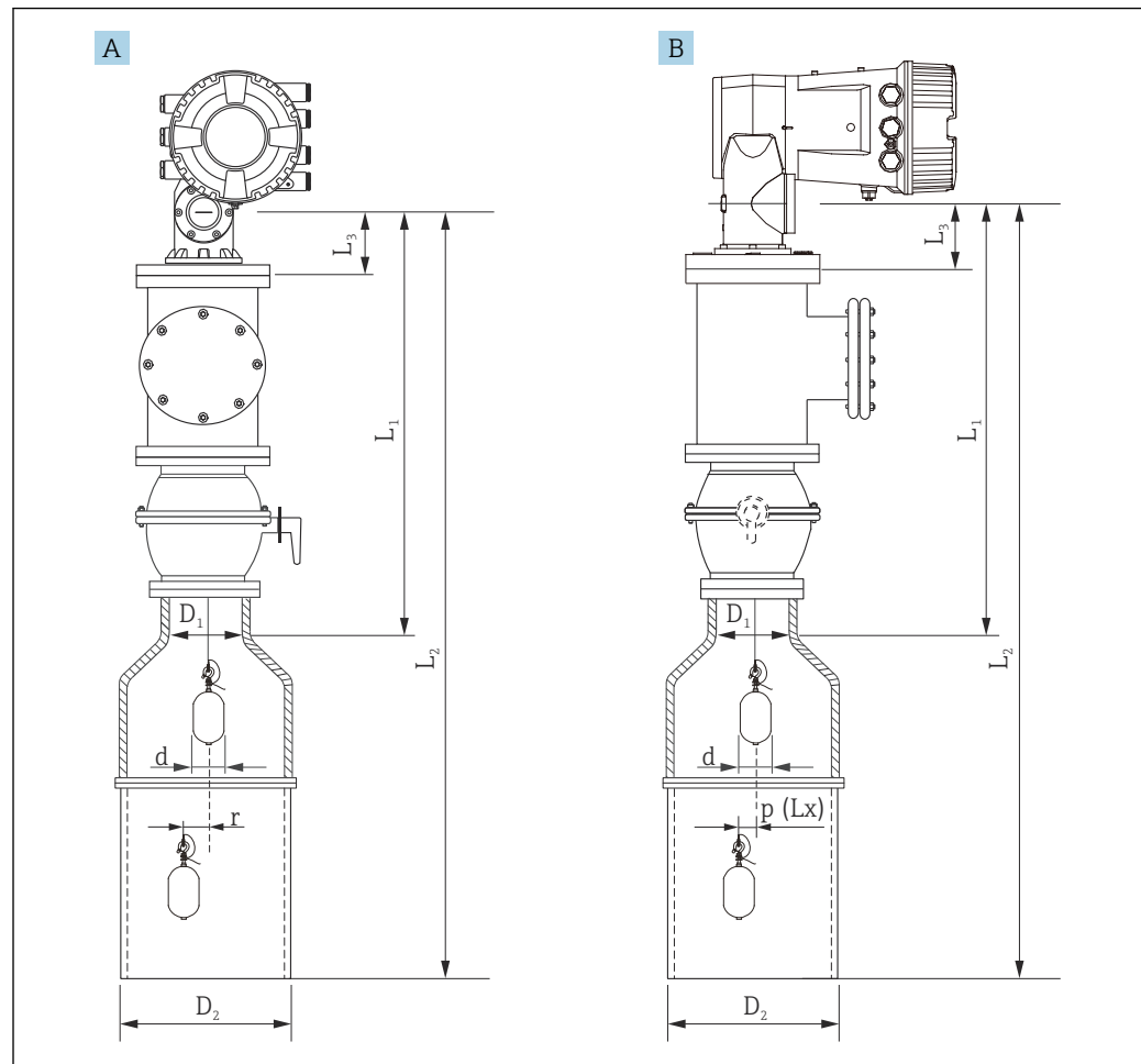
图 7 对中导波管的安装示意图
