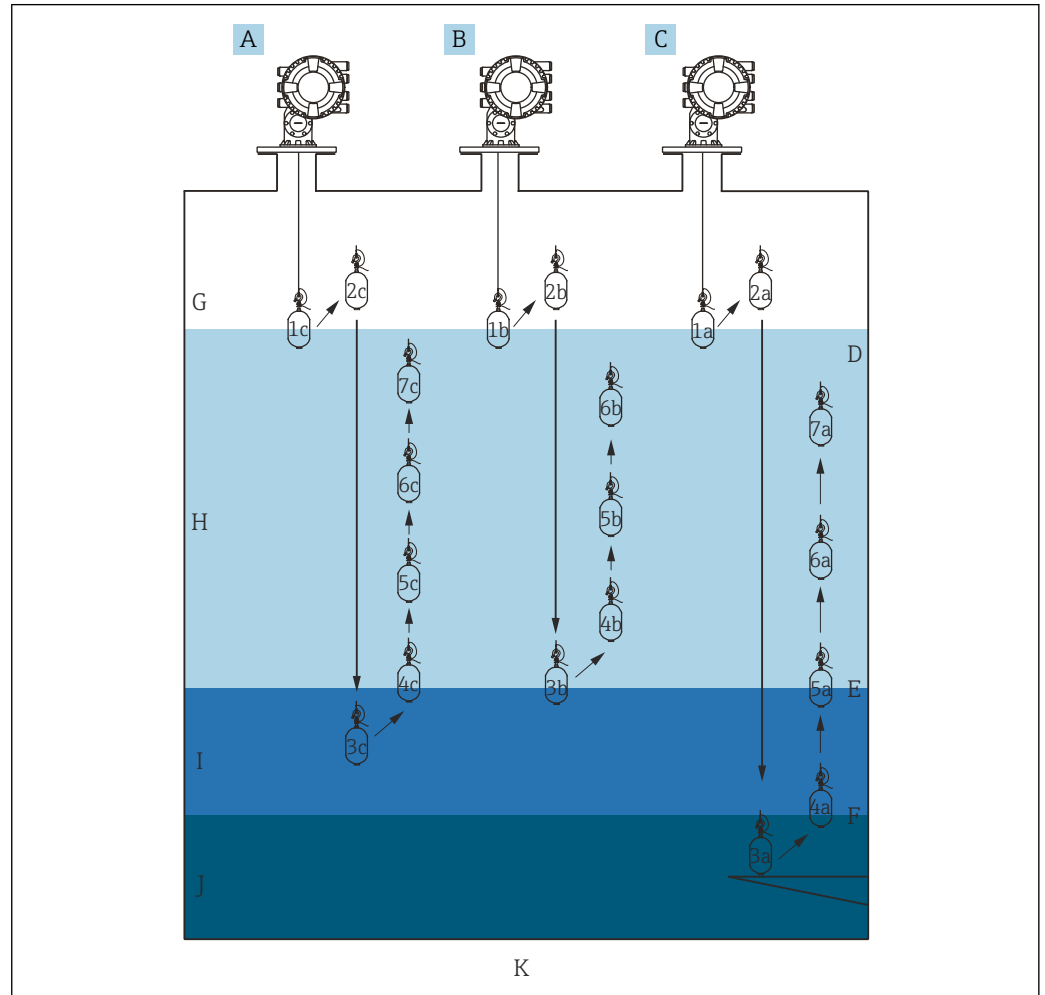
图 54 密度梯度概述 (1a、2a、3a...显示浮子移动顺序) 示意图
