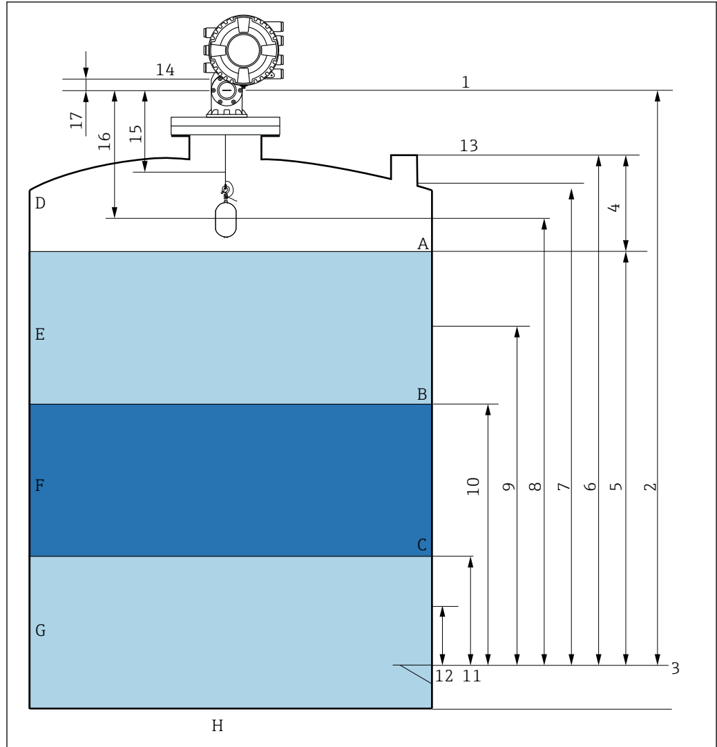
图 41 NMS8x 安装术语 (例如 NMS81)
