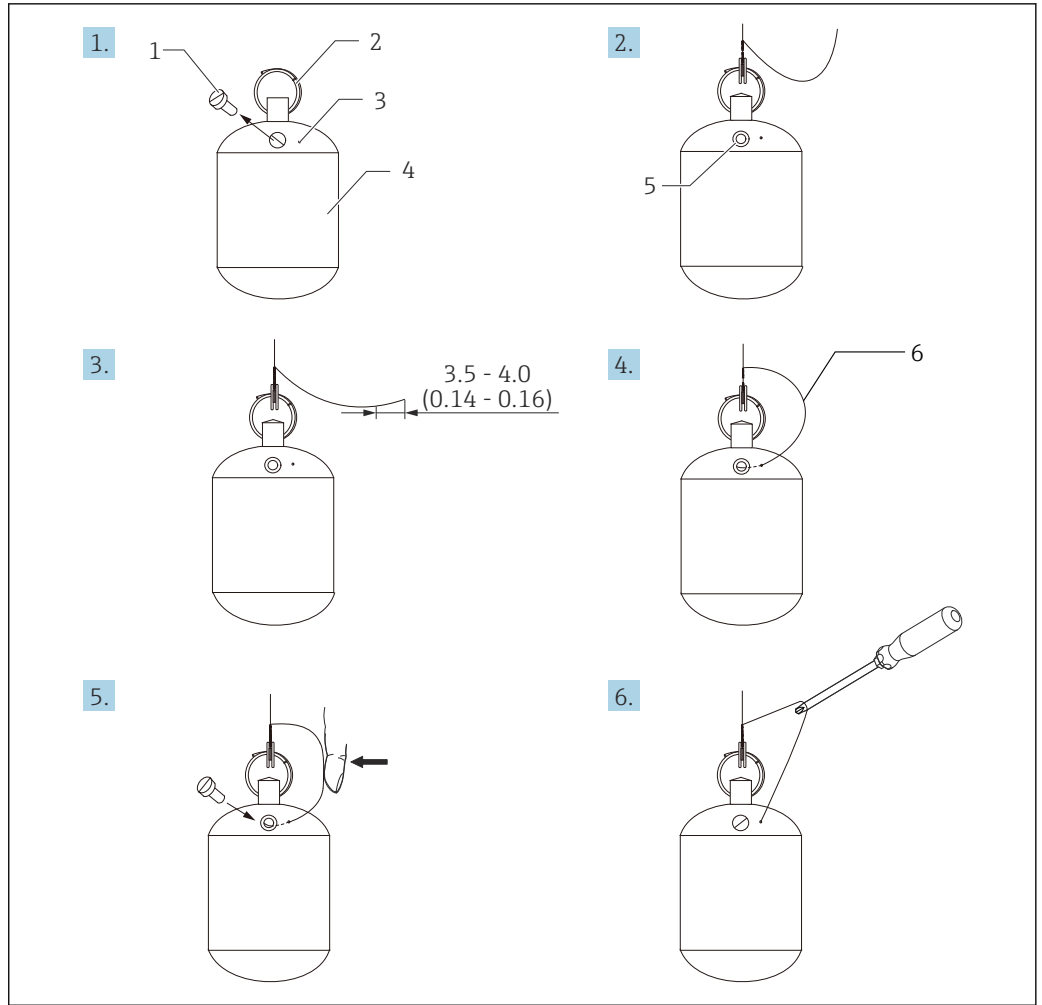
图 17 PTFE 材质型浮子的安装示意图；单位：mm (in)
