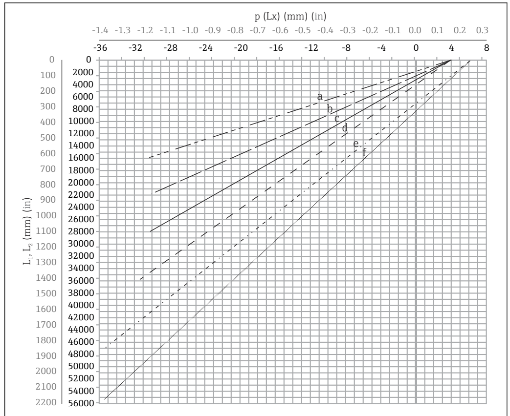
图 9 测量范围内的浮子横向偏差示意图
