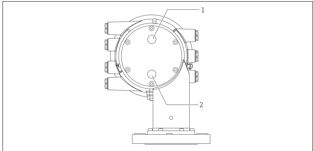
图 82 清洗短管和气体吹扫短管的连接孔口
