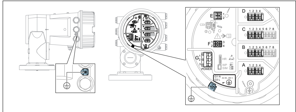
图 18 端子接线腔（典型实例）和接地端子示意图
