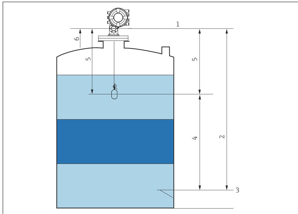
图 85 执行待机液位测量罐表命令期间，浮子等待液位上升
