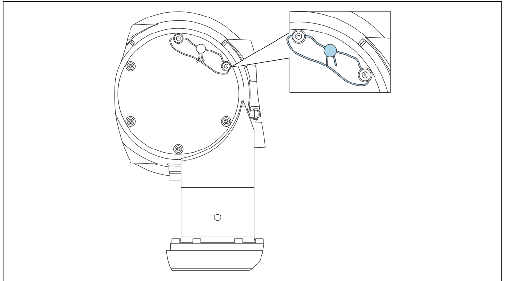
图 36 后盖板密封 (图例为 NMS80)
