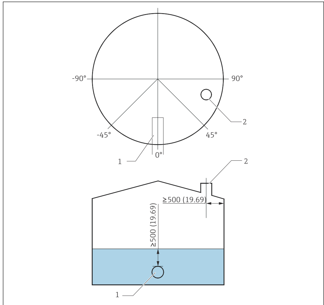
图 13 NMS8x 的推荐安装位置和最低测量液位；单位：mm (in)
