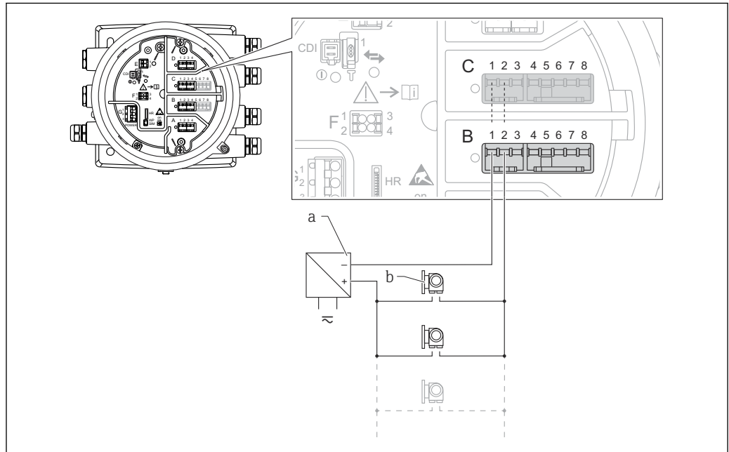
图 24 HART 主站模式下的无源模拟量输入/输出模块
