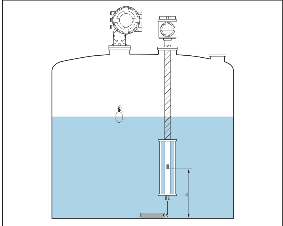
图 59 Prothermo NMT53x: 罐底测温元件位置
