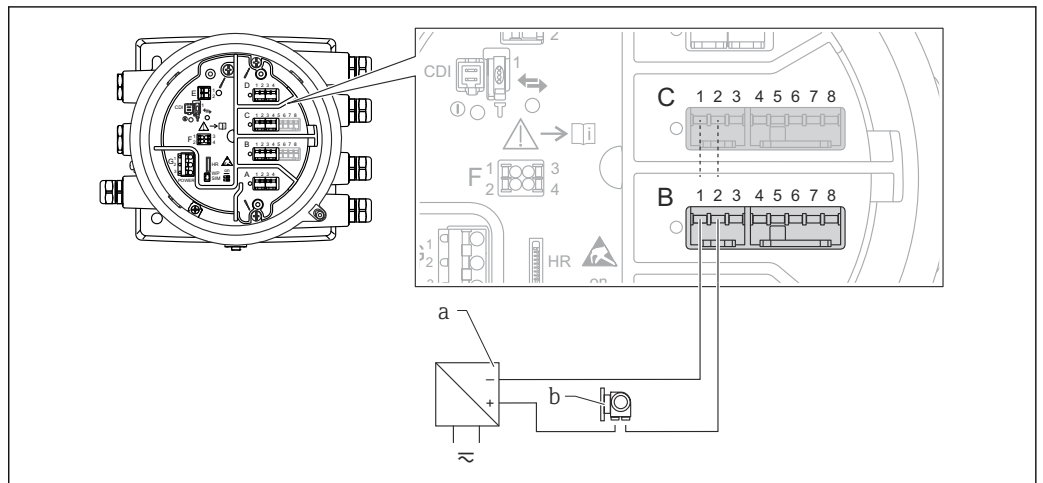
图 23 输入模式下的无源模拟量输入/输出模块
