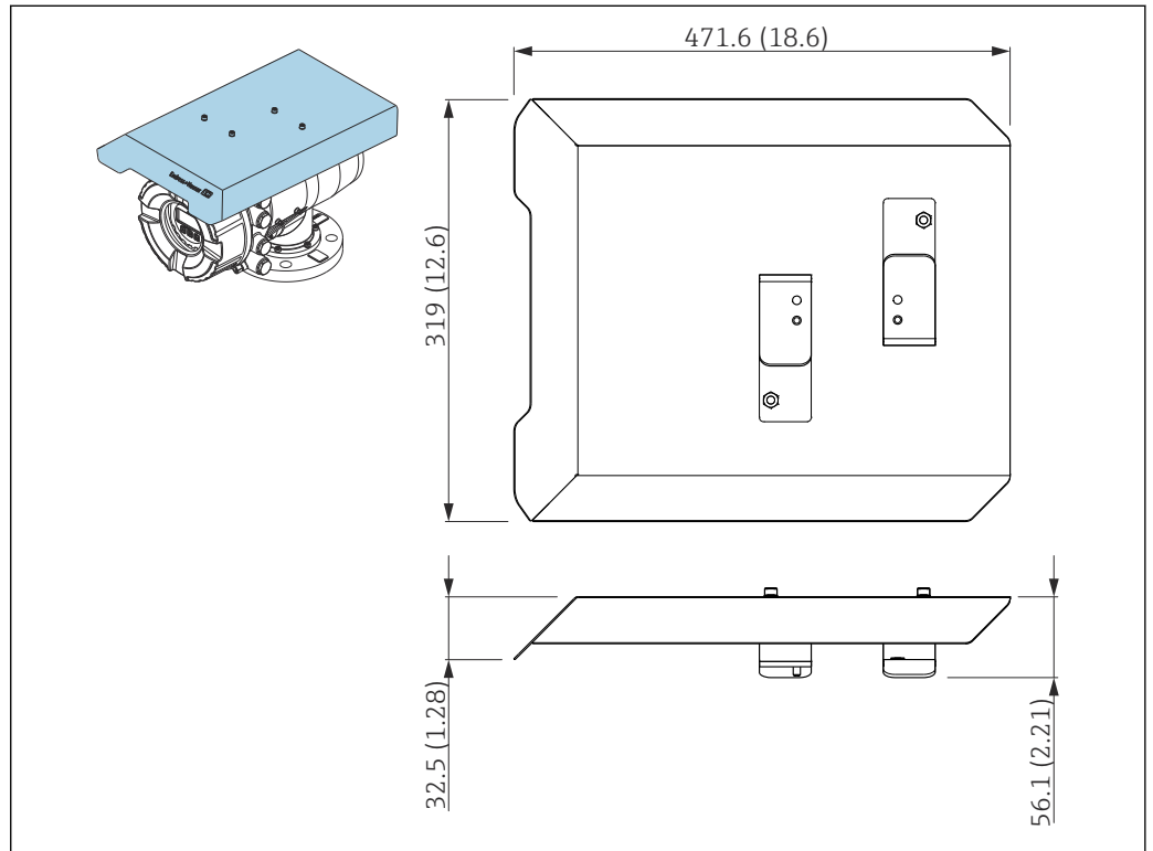
图 78 防护罩的外形尺寸示意图；单位：mm (in)
