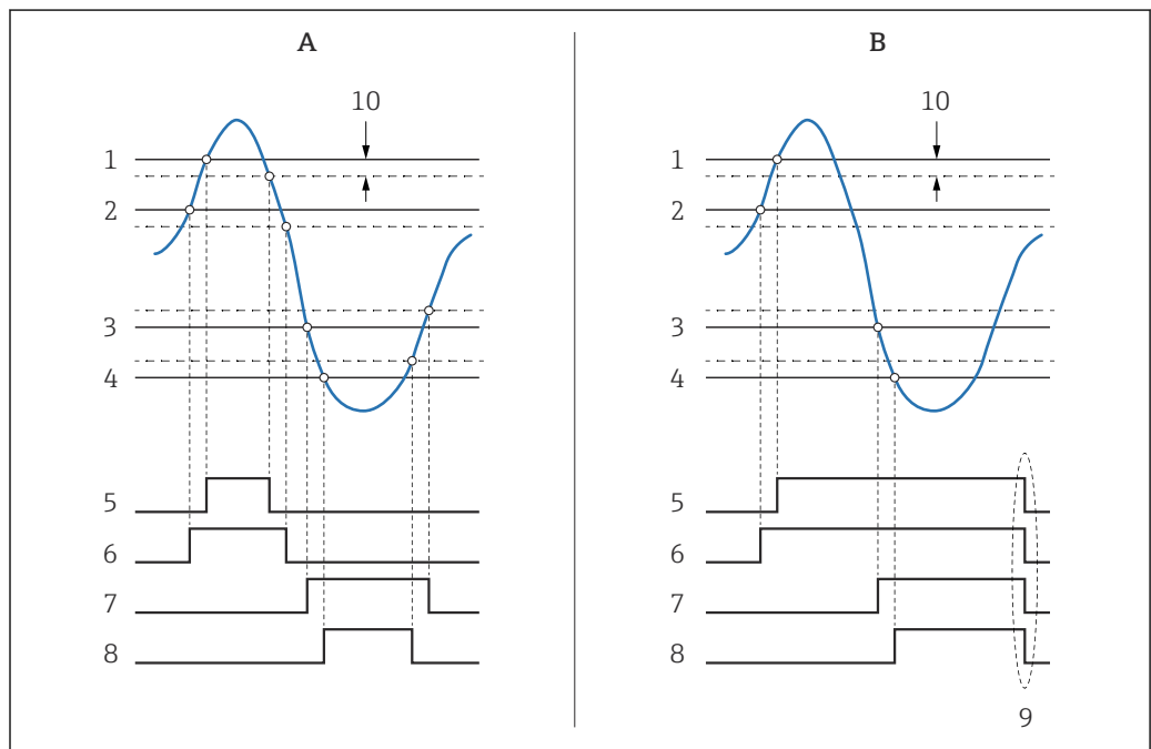
图 98 限定值计算原理
