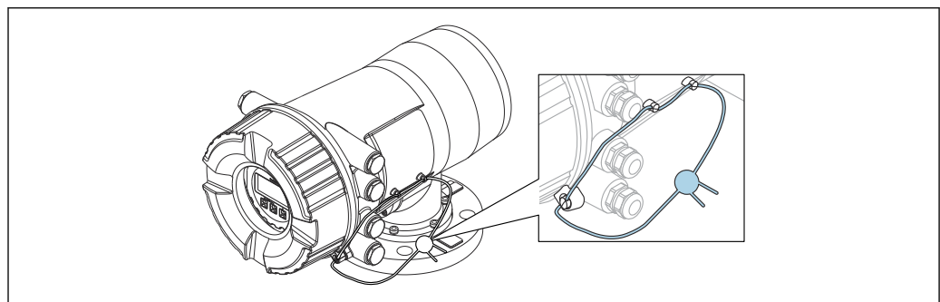
35 密封接线腔盖板
