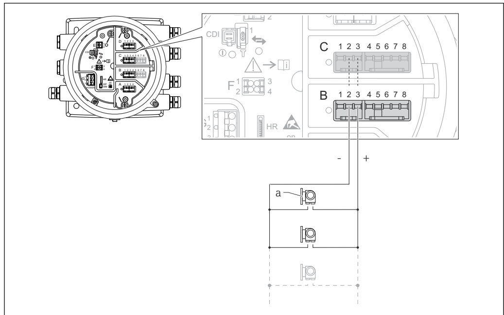
图 27 HART 主站模式下的有源模拟量输入/输出模块
