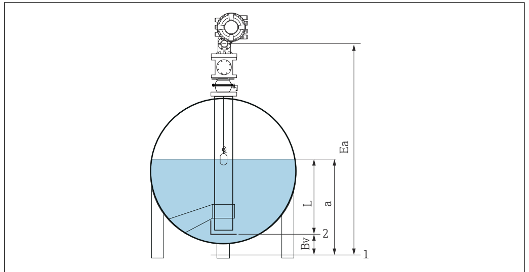
图 51 适用 NMS80 和 NMS81 的封闭式罐体
