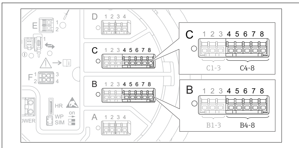
图 63 已连接 RTD 的模拟量输入/输出模块的可能安装位置。设备的订货号确定当前使用的模块 → 图 45。
