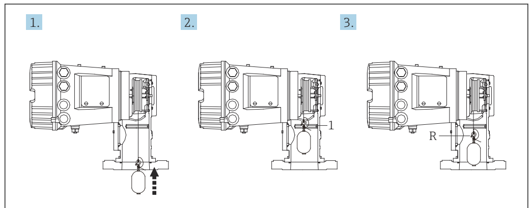
图 45 参考标定步骤
