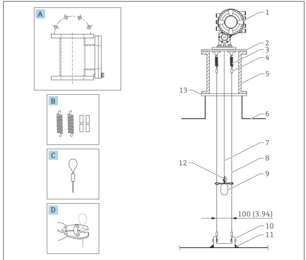
图 10 导向钢丝; 单位: mm (in)
