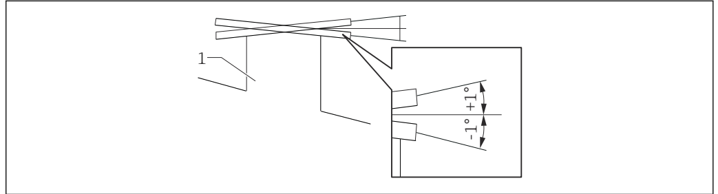
图 12 安装法兰的允许偏差角度范围
