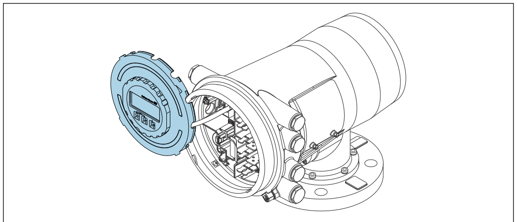
图 37 NMS80: 显示单元安装在接线腔边缘处
