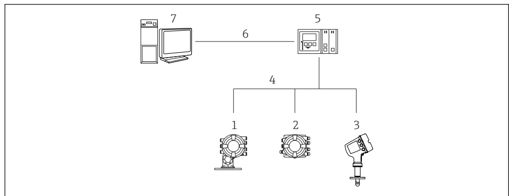
图 40 通过 Tankvision 储罐扫描仪 NXA820 连接雷达液位仪至 FieldCare
