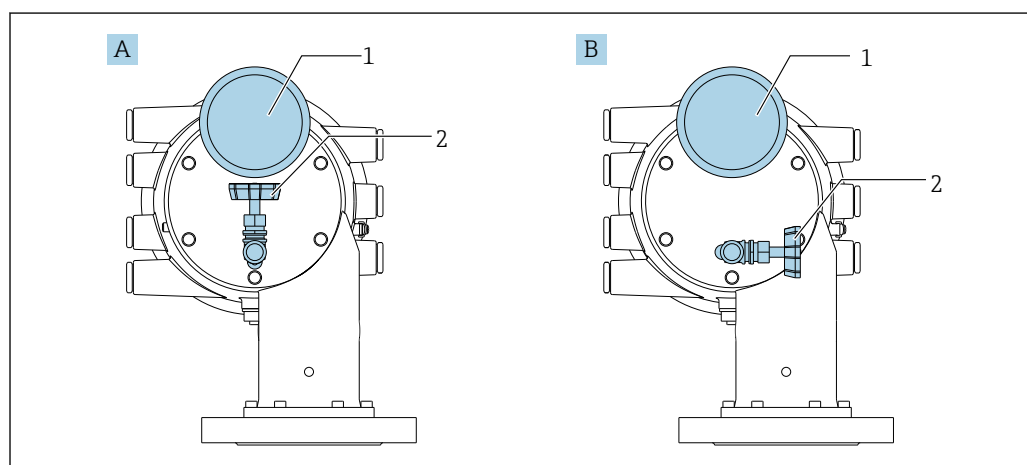
图 79 减压阀和压力表的安装位置
