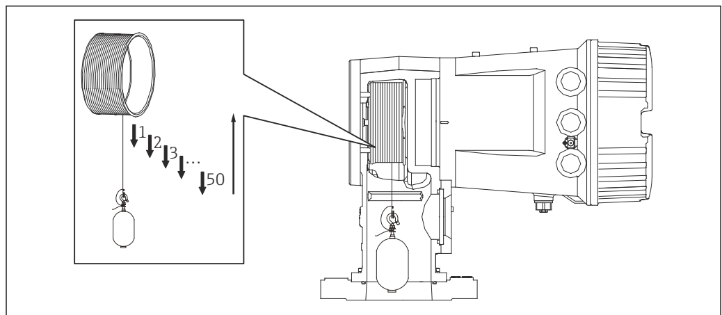
图 46 创建轮鼓表格
