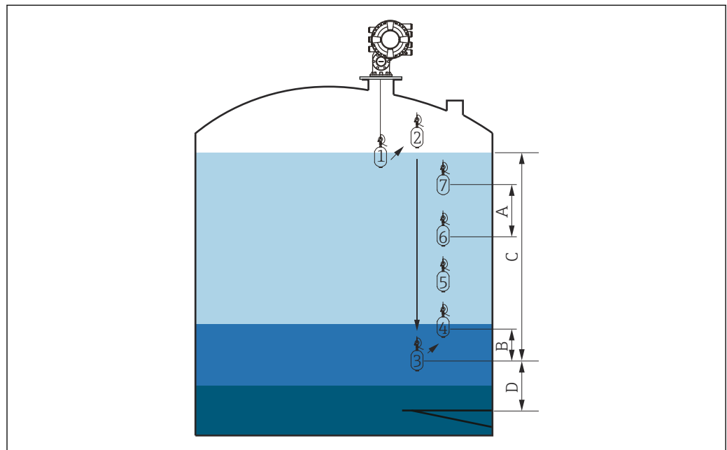
图 57 手动梯度位移（数字显示浮子的移动顺序）示意图
