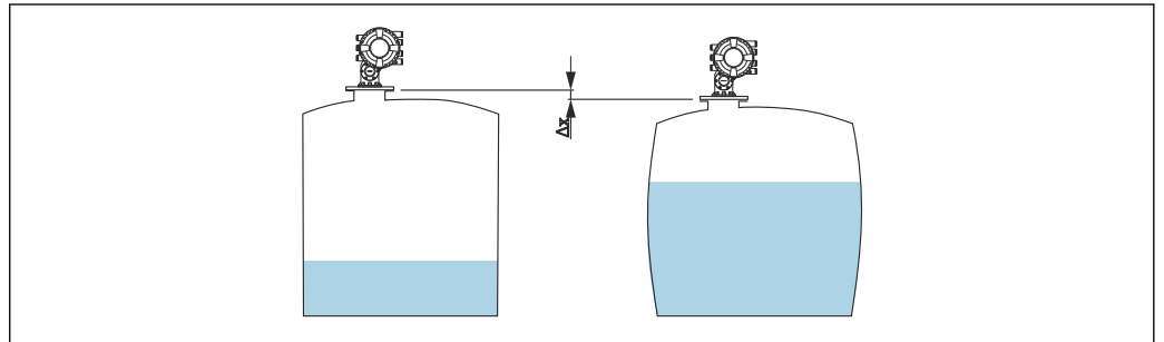
图 24 静压力导致罐体外壳膨胀，从而引起罐体参考高度位移 \Delta x
