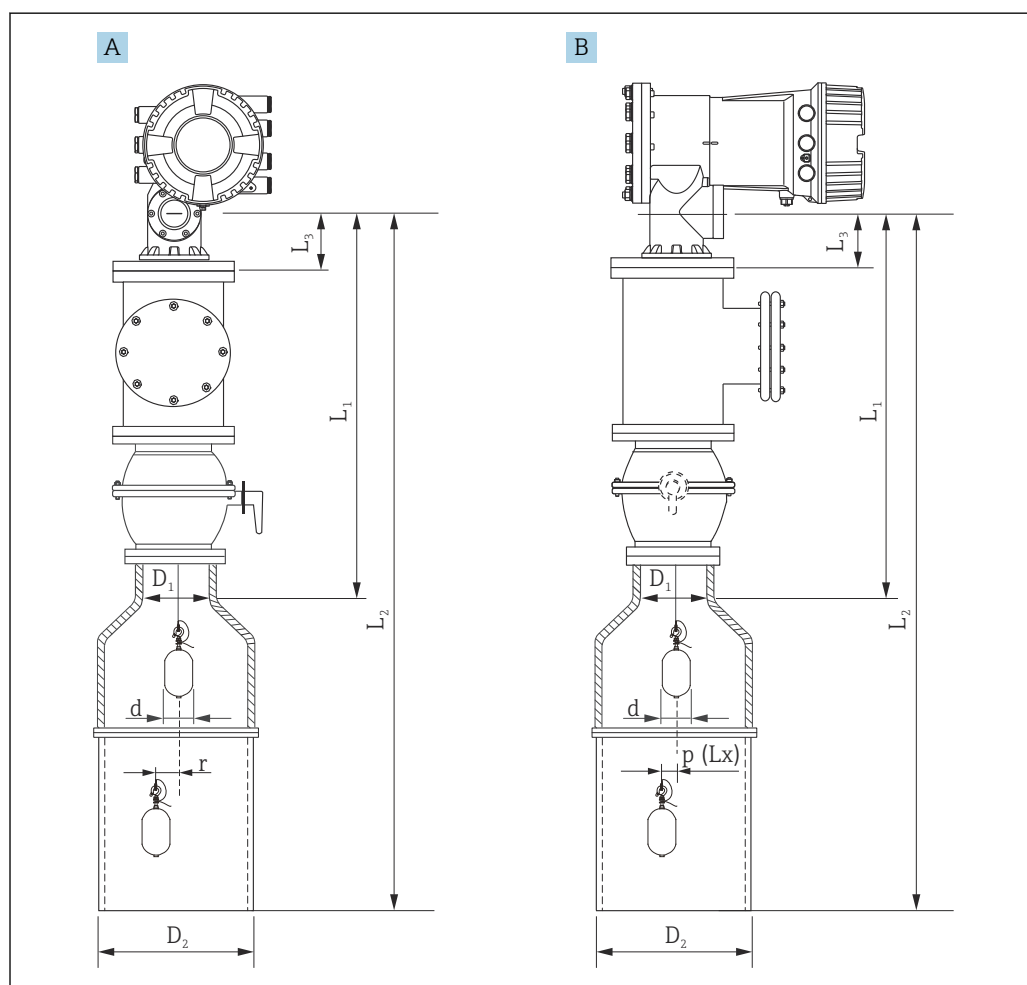
图 14 对中导波管的安装示意图
