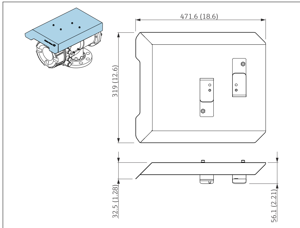
图 25 防护罩的外形尺寸示意图；单位：mm (in)
