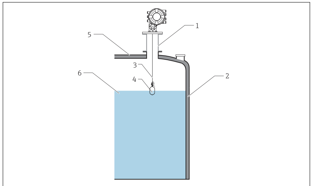
18 过程密封
