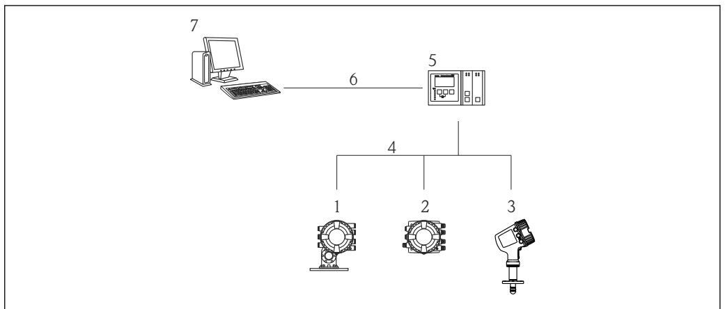
图 22 储罐计量仪表的远程操作
