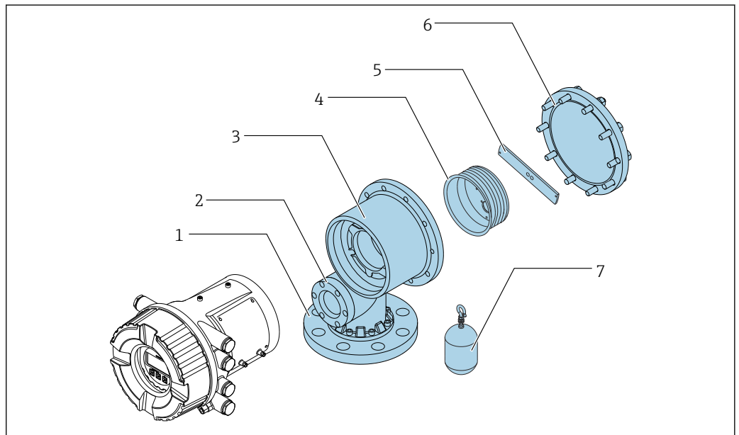
图 19 可以选配 NACE 标准材质的部件
