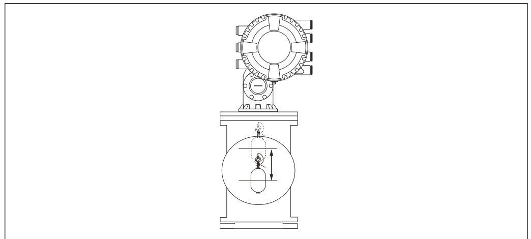
图 43 移动浮子
