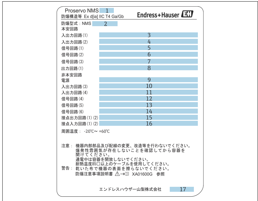
图 4 TIIS 认证型 Proservo NMS8x 的铭牌
