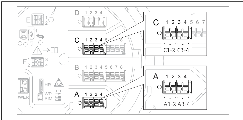
图 74 数字量输入/输出模块的可能安装位置 (实例)；订货号定义数字量输入/输出模块的数量和位置 → 图 44。
