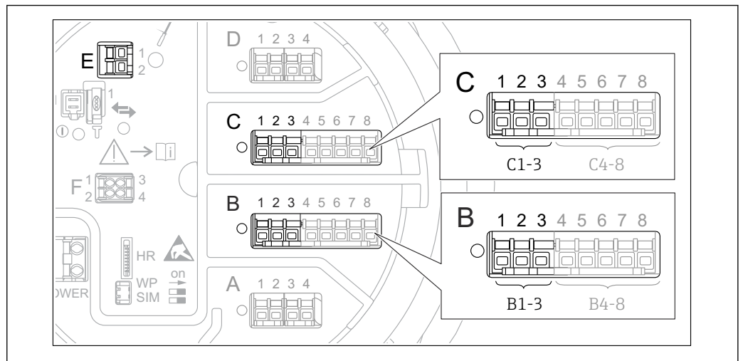
图 58 HART 回路的可能接线端子
