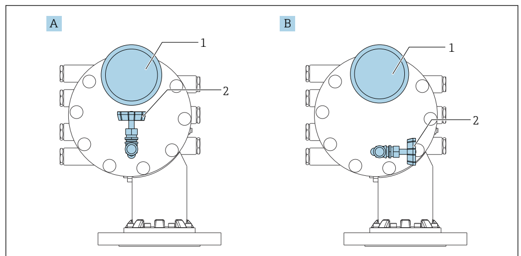
图 79 减压阀和压力表的安装位置
