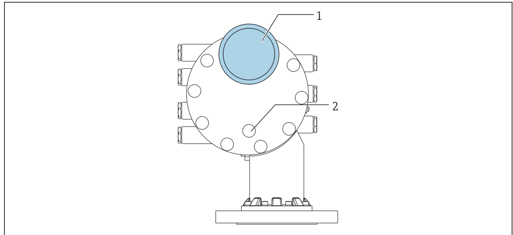
图 84 压力计和气体吹扫短管
