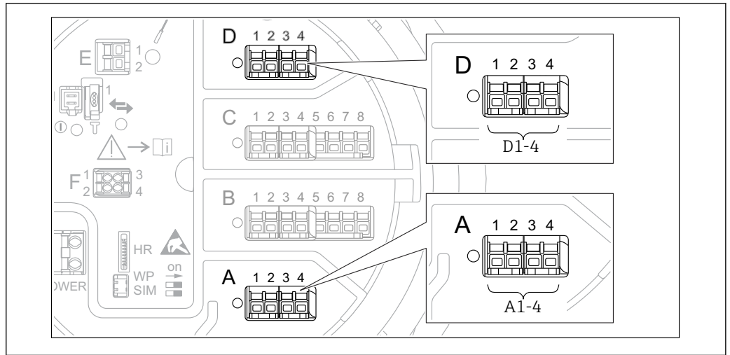
图 71 Modbus 模块的可能安装位置示例；取决于仪表型号，上述模块可以安装在插槽 B 或 C 中 → 图 44。
