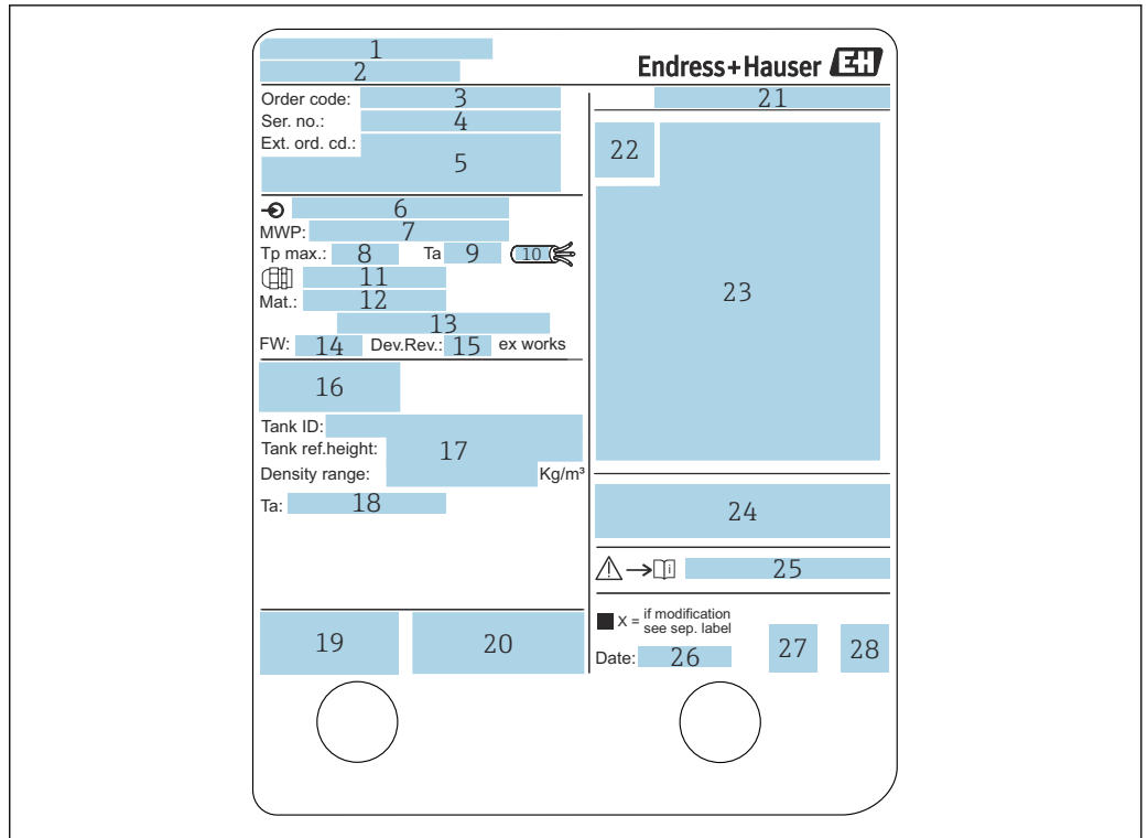
图 3 铭牌
