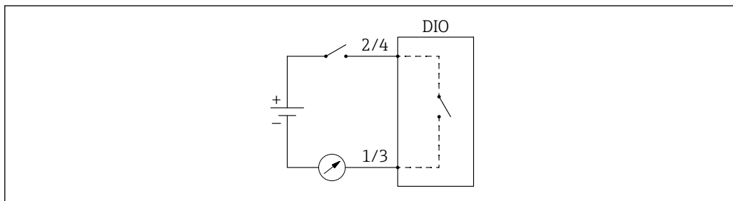
图 75 数字量输入输出模块用作数字量输出
