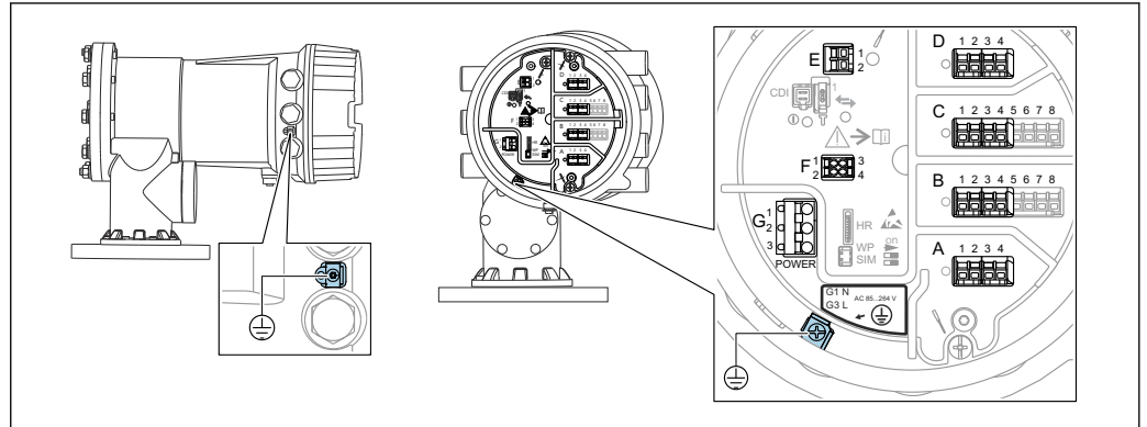
图 18 端子接线腔（典型实例）和接地端子示意图
