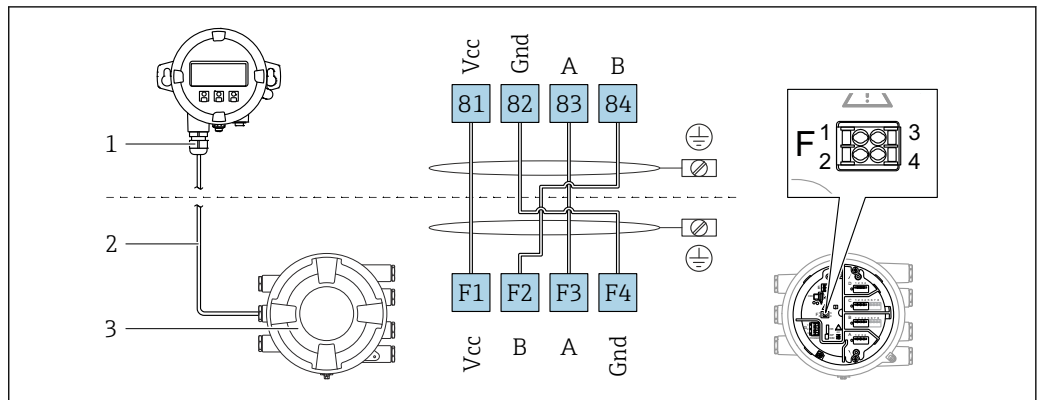
图 20 分离型显示与操作单元 DKX001 连接至罐旁指示仪 (NMR8x、NMS8x 或 NRF8x)
