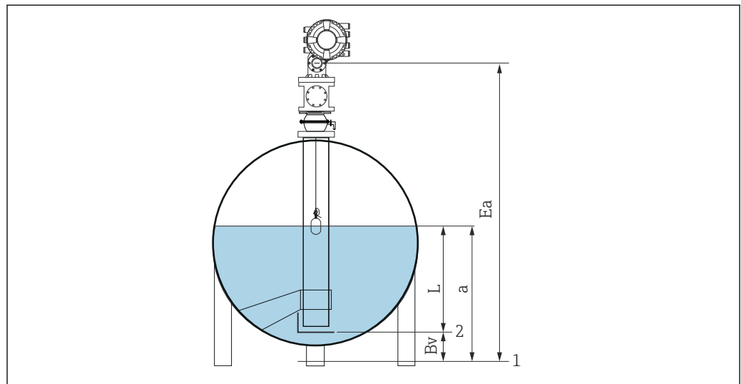
图 51 适用 NMS80 和 NMS81 的封闭式罐体
