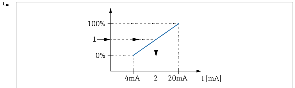
图 69 按输出电流调整罐体参数
