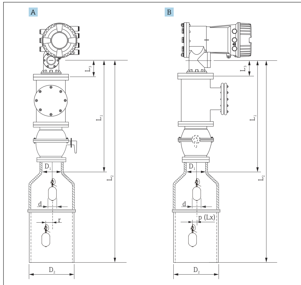
图 7 对中导波管的安装示意图
