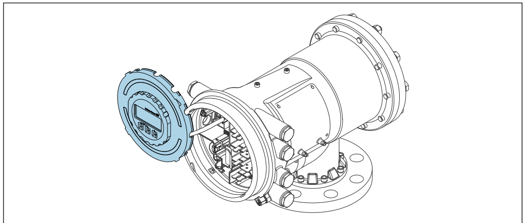
图 37 NMS81: 显示单元安装在接线腔边缘处
