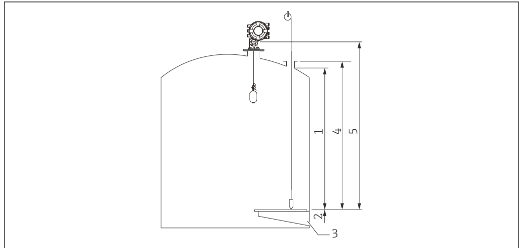
图 48 罐体高度
