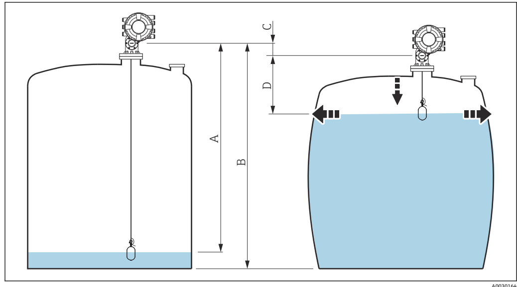
图 66 静压式储罐变形校正值 (HyTD)
