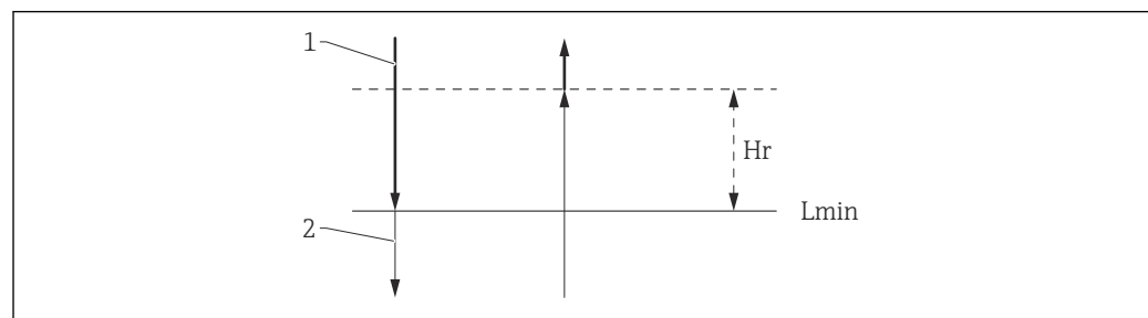
图 97 HTMS 单点回差控制范围
