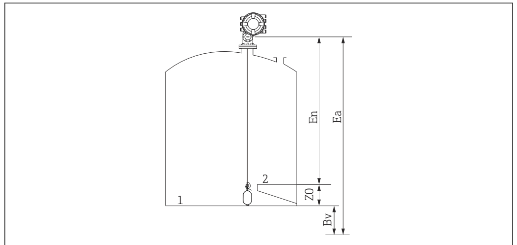
图 50 敞开式无液体储罐
