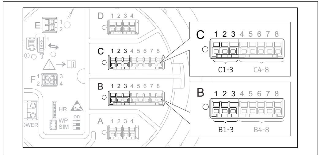
图 68 用作 4...20 mA 输出的模拟量输入/输出模块的可能安装位置。仪表订货号确定当前使用模块 → 图 44。
