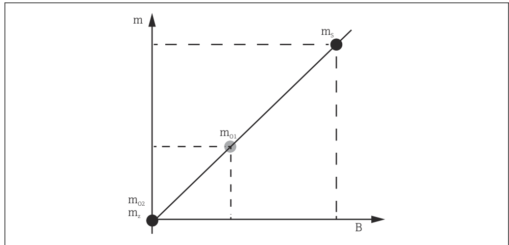
图 44 传感器标定原理
