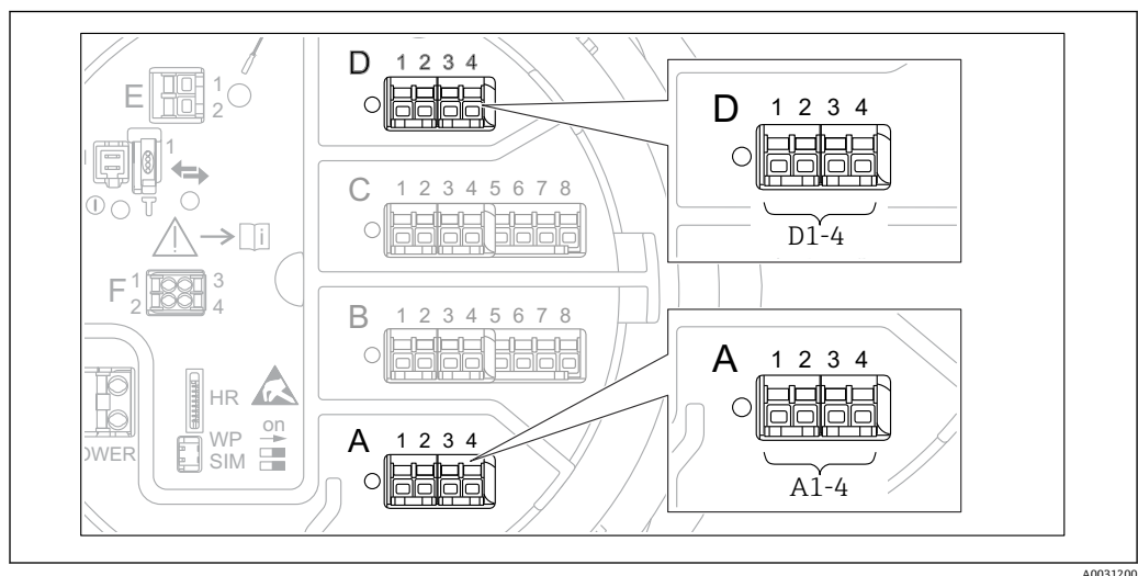
图 73 WM550 模块的可能安装位置（实例）；取决于设备型号，上述模块还可以安装在插槽 B 或 C 中 → 图 44。
