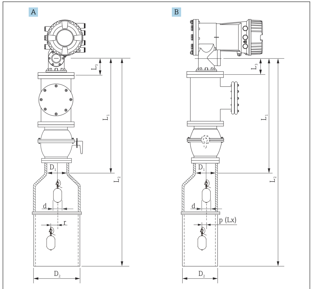
图 8 非对中导波管的安装示意图
