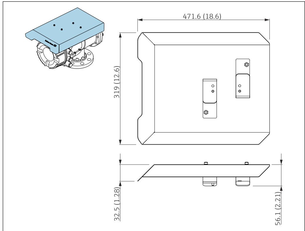
图 78 防护罩的外形尺寸示意图；单位：mm (in)
