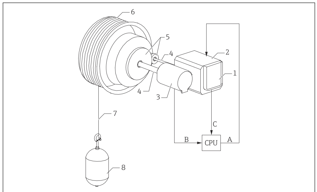
图 1 工作原理
