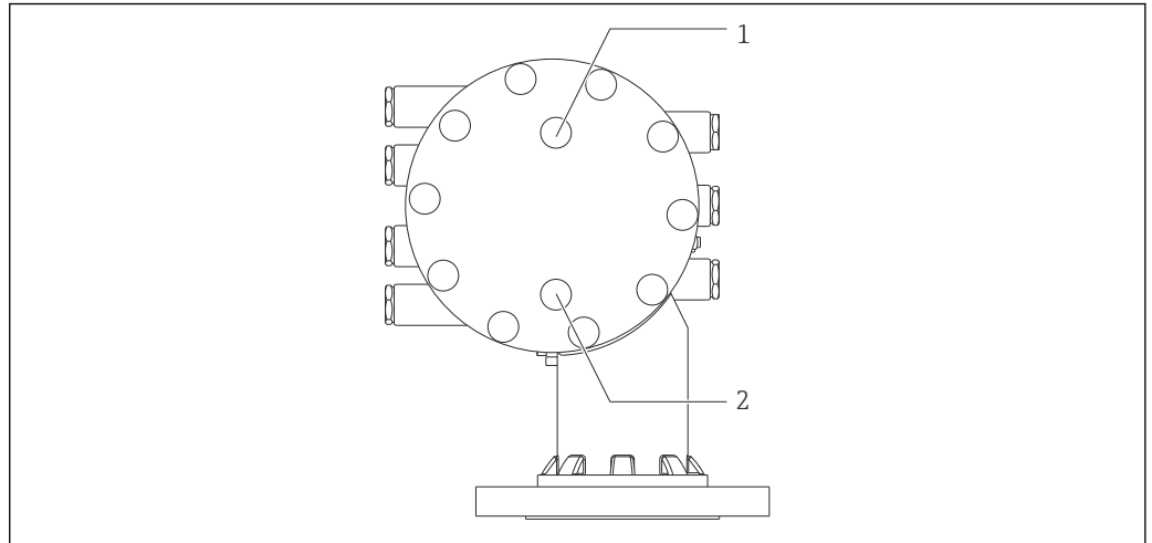
图 27 清洗短管和气体吹扫短管的连接孔口
