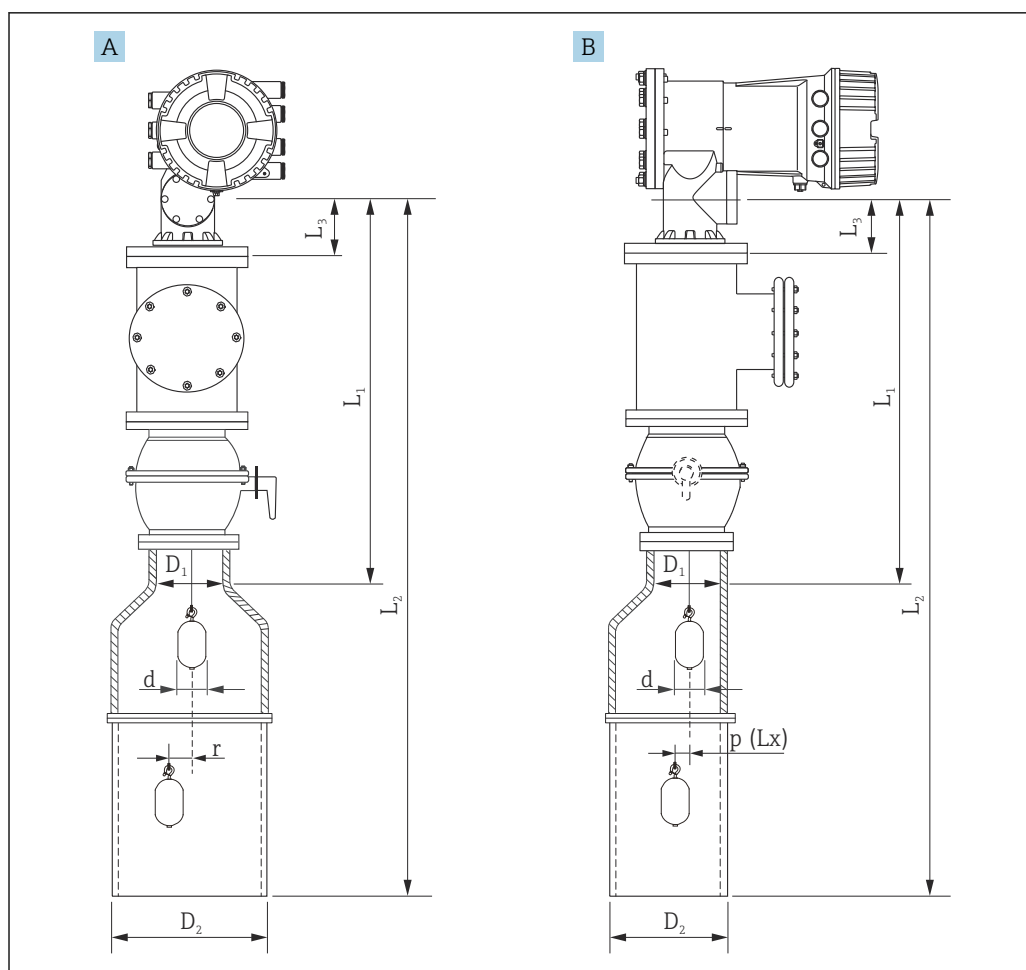
图 15 非对中导波管的安装示意图
