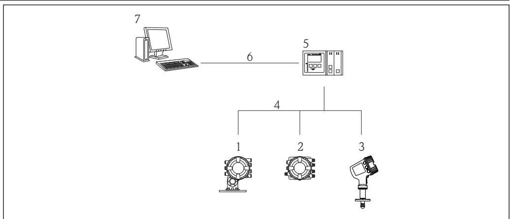
图 20 储罐计量仪表的远程操作
