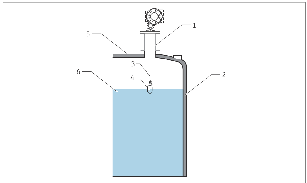
17 过程密封
