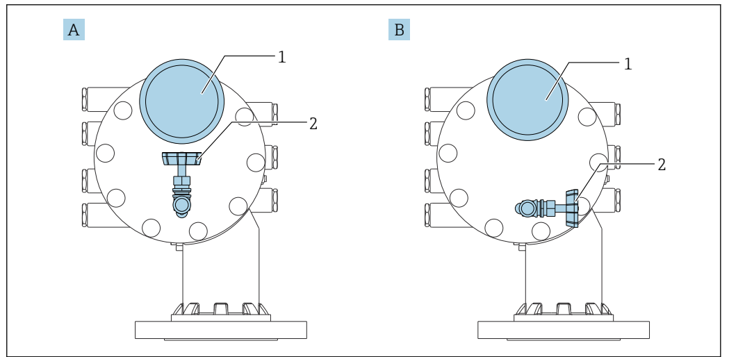
图 24 减压阀和压力表的安装位置
