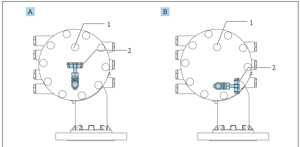
图 28 清洗短管和减压阀
