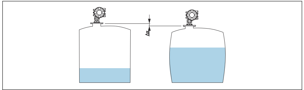
图 22 静压力导致罐体外壳膨胀，从而引起罐体参考高度位移 \Delta x
