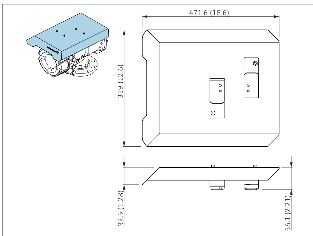
图 23 防护罩的外形尺寸示意图；单位：mm (in)
