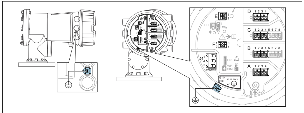
图 11 端子接线腔（典型实例）和接地端子示意图
