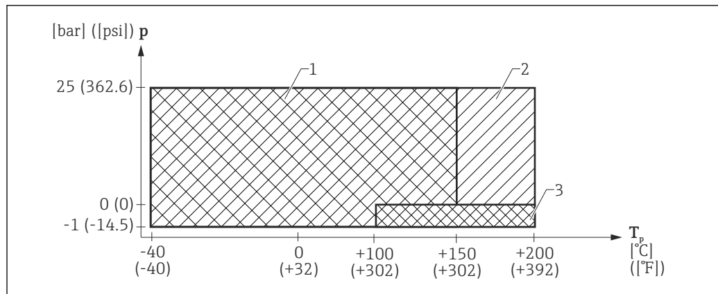
图 23 FMR62: 允许过程温度和过程压力范围, 带法兰或 DIN11851 过程连接
