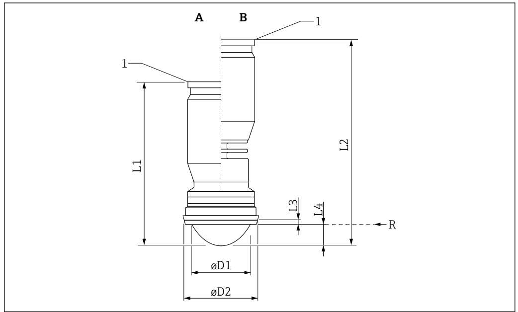
图 29 外形尺寸示意图: PTFE 涂层天线, 带 DIN 11851 卫生型转接头。测量单位 mm (in)
