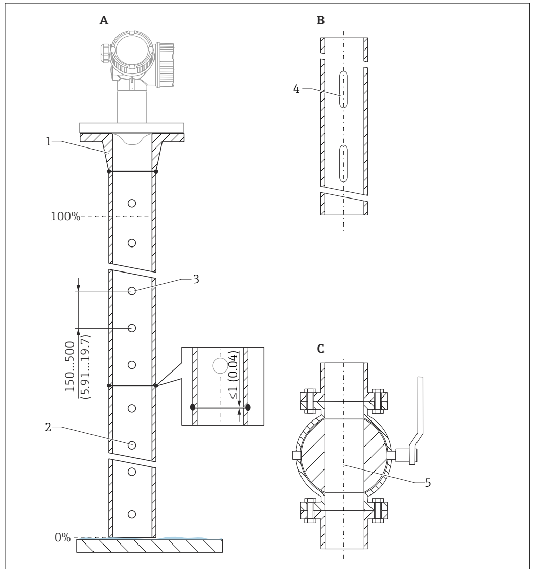
图 16 导波管设计实例。测量单位 mm (in)
