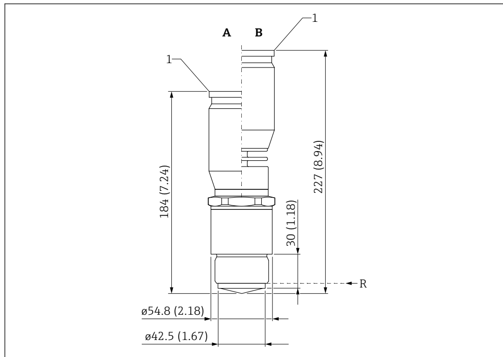
图 28 外形尺寸示意图: PEEK 一体型天线, 40 mm (1-1/2"); 1-1/2"螺纹过程连接。测量单位 mm (in)
