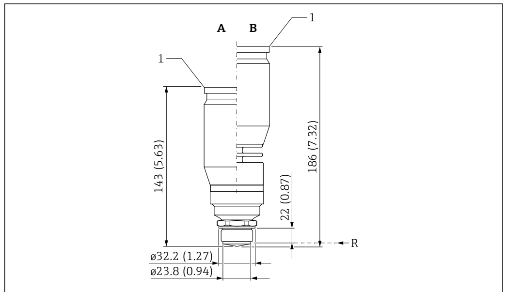
图 27 外形尺寸示意图: PEEK 一体型天线, 20 mm (3/4"); 3/4"螺纹过程连接。测量单位 mm (in)
