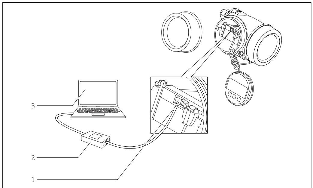
36 DeviceCare/FieldCare, 使用服务接口 (CDI)
