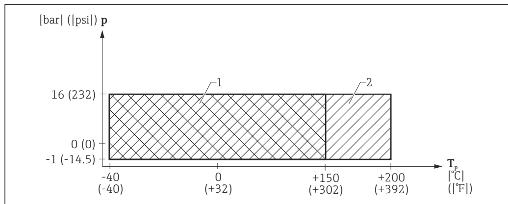
图 21 FMR62: 允许过程温度和过程压力范围, 带 Tri-Clamp 2"卡箍过程连接
