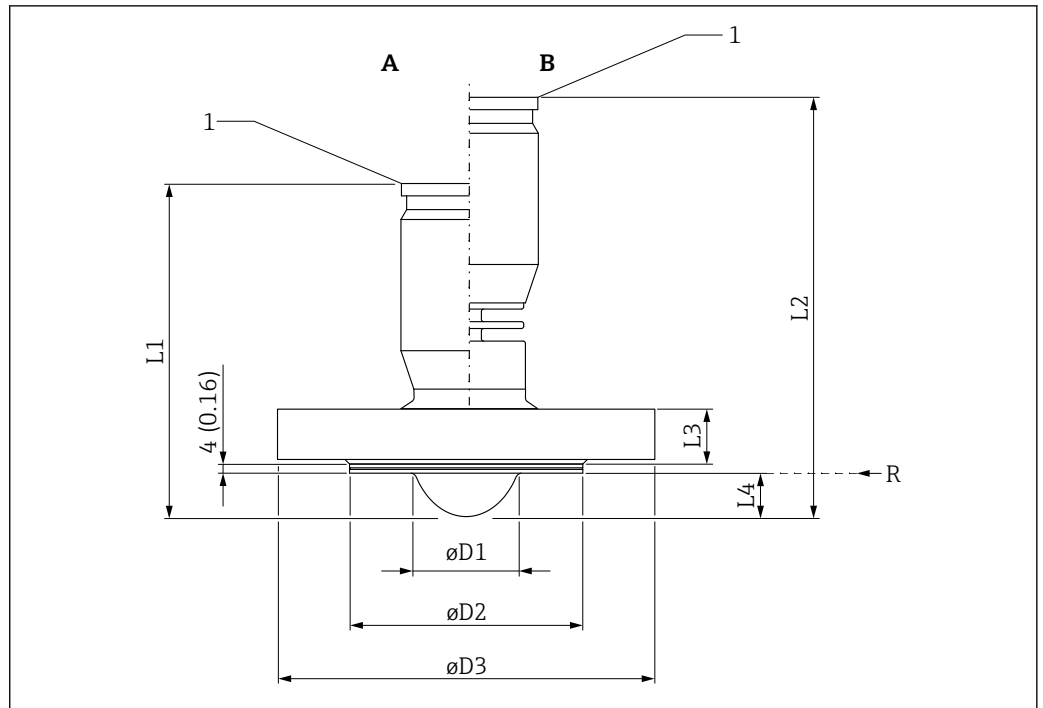
图 31 外形尺寸示意图: PTFE 涂层天线, 带 EN1092-1、ASME B16.5 或 JIS B2220 法兰。测量单位 mm (in)
