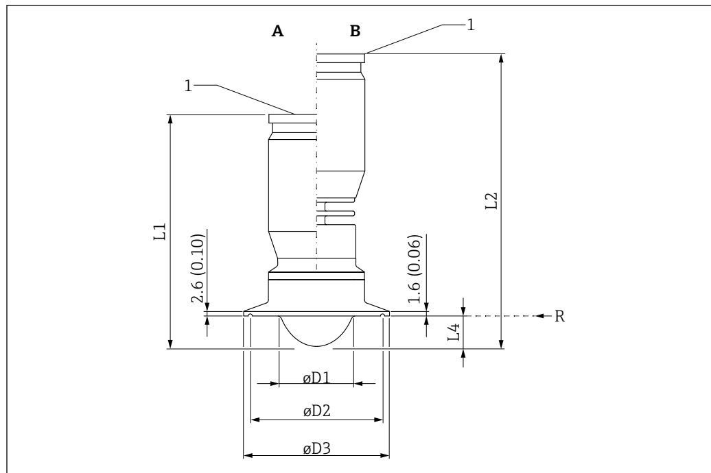
图 30 外形尺寸示意图: PTFE 涂层天线, 带 Tri-Clamp 卡箍。测量单位 mm (in)
