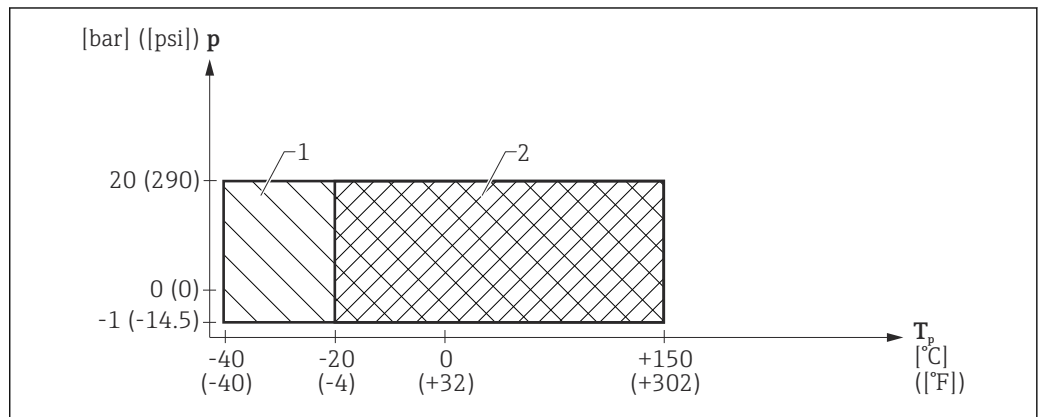
图 19 FMR62: 允许过程温度和过程压力范围, 带 PEEK 一体型天线 (订购选项 070, 选型代号: GE、GF), 150 °C (302 °F)
