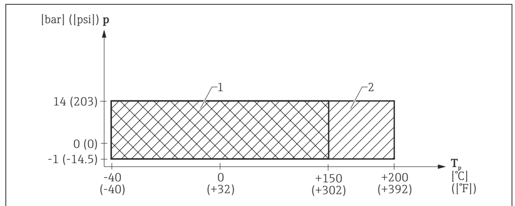
图 22 FMR62: 允许过程温度和过程压力范围, 带 Tri-Clamp 3"或 Tri-Clamp 4"卡箍过程连接
