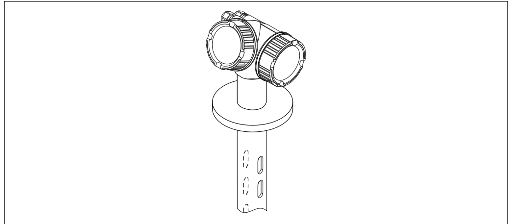
图 15 安装在导波管中
