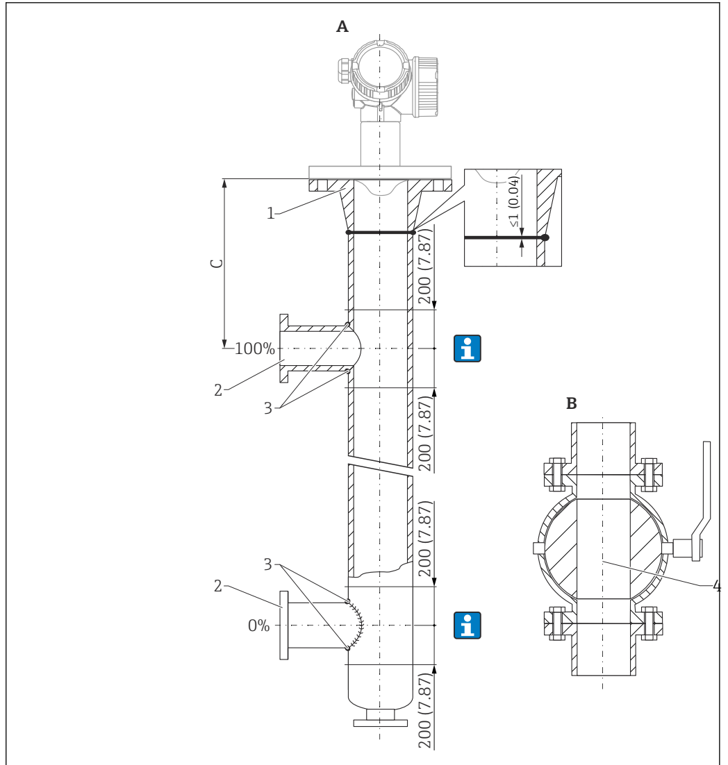
18 旁通管设计实例。测量单位 mm (in)
