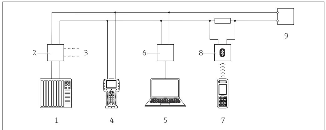
35 通过 HART 通信进行远程操作
