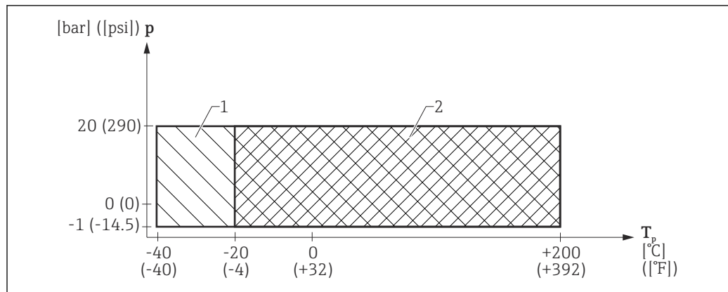
图 20 FMR62: 允许过程温度和过程压力范围, 带 PEEK 一体型天线 (订购选项 070, 选型代号: GE、GF), 200 °C (392 °F)
