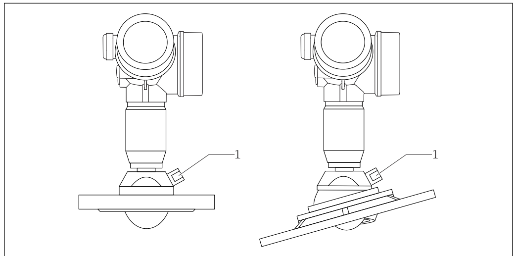
图 17 齐平安装天线的内置空气吹扫接口
