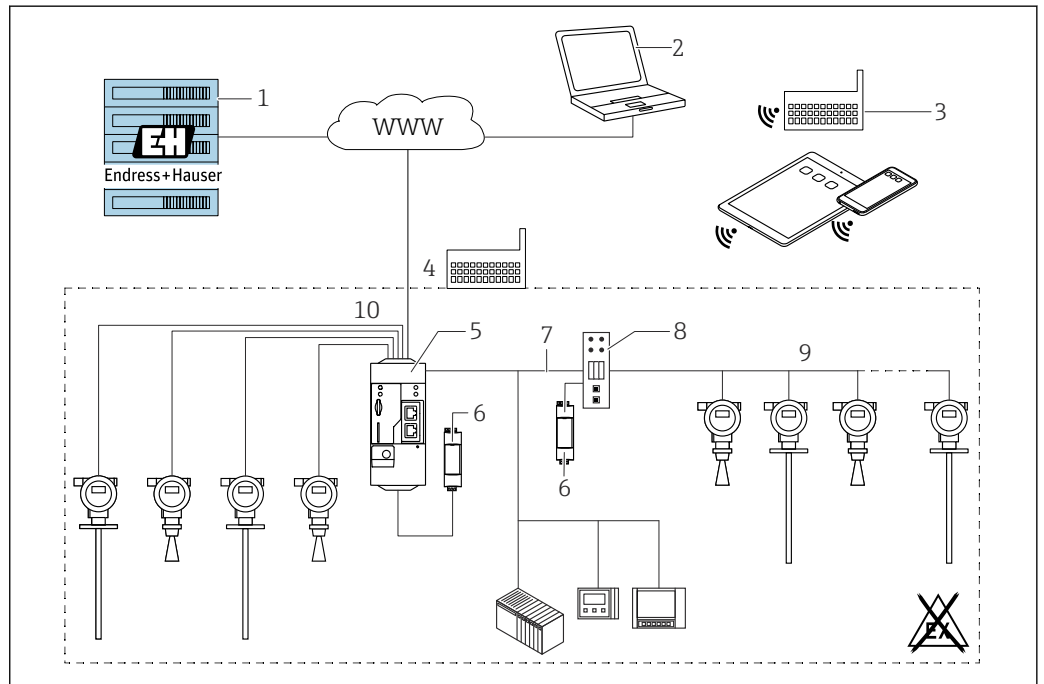
图 40 SupplyCare Hosting SCH30 的库存管理平台示例
