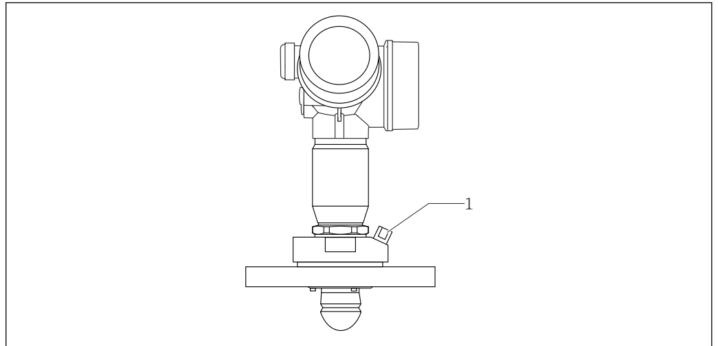
图 16 水滴型天线的空气吹扫接口
