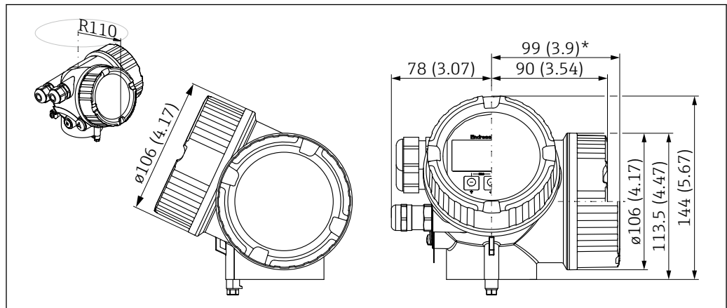
图 23 GT19 外壳 (塑料 PBT)。测量单位 mm (in)
