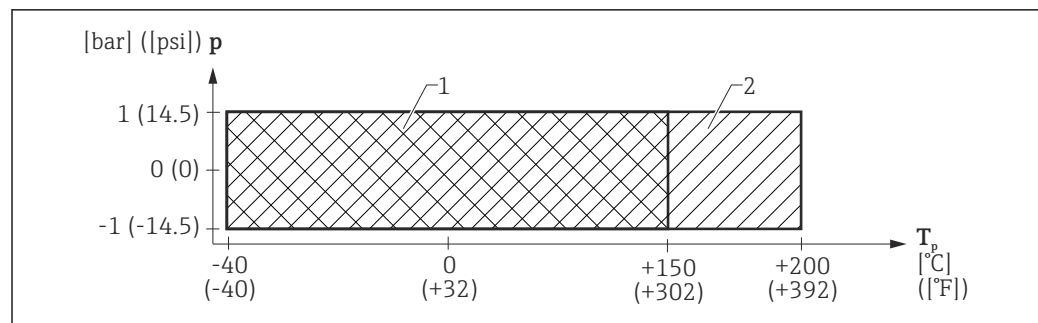
图 20 FMR67: 允许过程温度和过程压力范围, 带 PTFE 齐平安装天线, DN80; UNI 法兰, 316L
