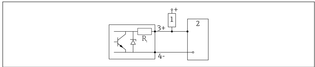
图 10 连接数字量输入
