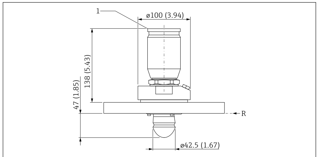
图 27 外形尺寸示意图: 水滴型天线, 带空气吹扫接口。测量单位 mm (in)
