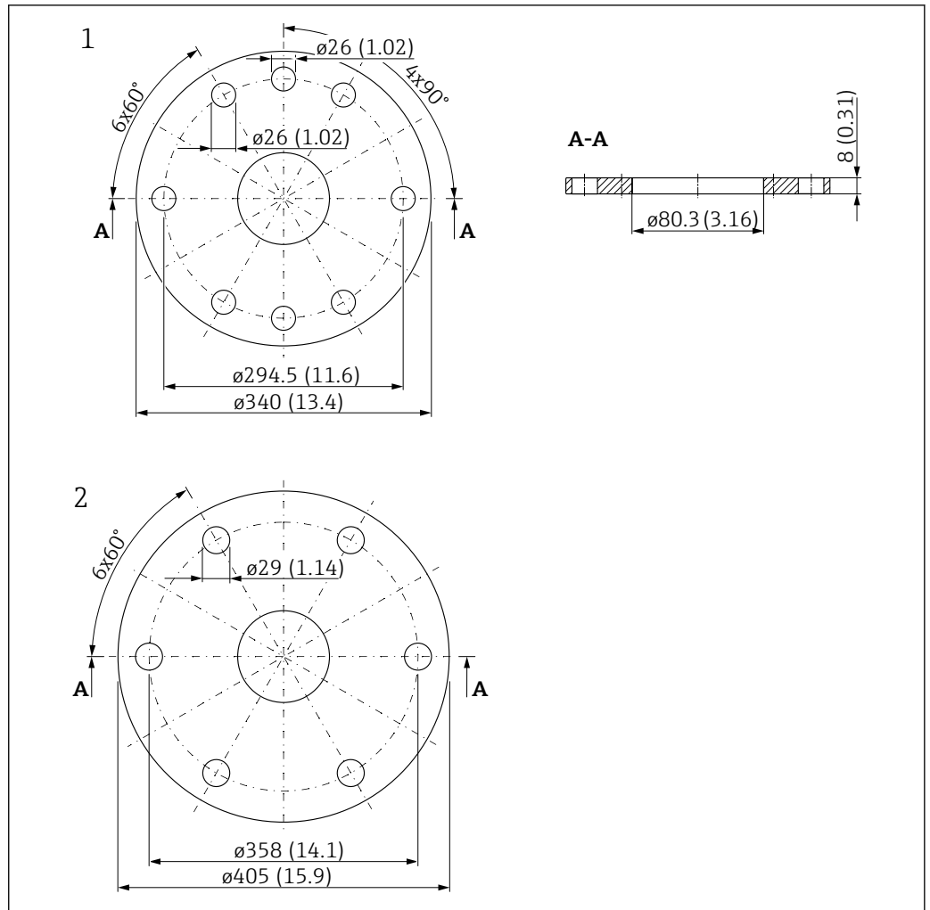
图 31 外形尺寸示意图: FMR67 的配套 UNI 法兰，带空气吹扫接口。测量单位 mm (in)
