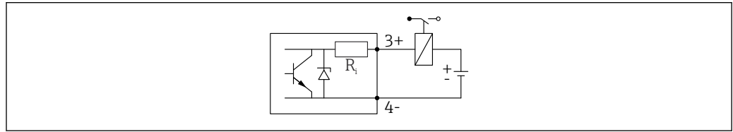
图 9 连接继电器
