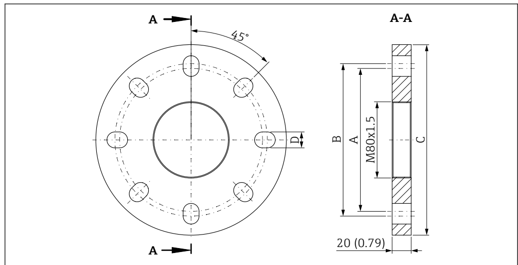
图 28 外形尺寸示意图：FMR67 的配套 UNI 法兰，带空气吹扫接口。测量单位 mm (in)
