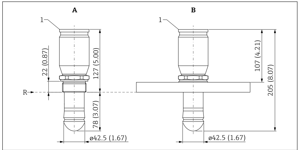
图 25 外形尺寸示意图: 水滴型天线, 不带空气吹扫接口。测量单位 mm (in)
