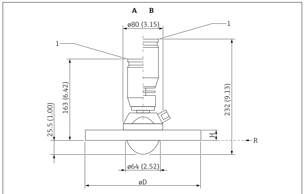
图 29 外形尺寸示意图: 齐平安装天线, 带标准法兰和空气吹扫接口。测量单位 mm (in)
