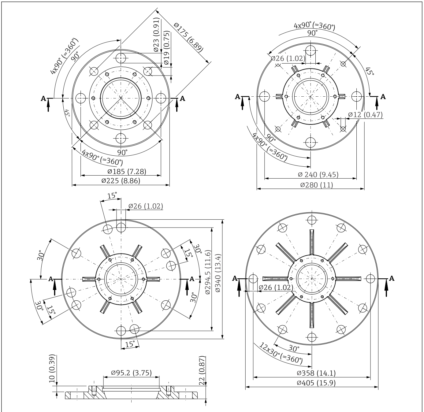
33 外形尺寸示意图: FMR67 的配套 UNI 法兰, 带天线角度调节装置和空气吹扫接口。测量单位 mm (in)
