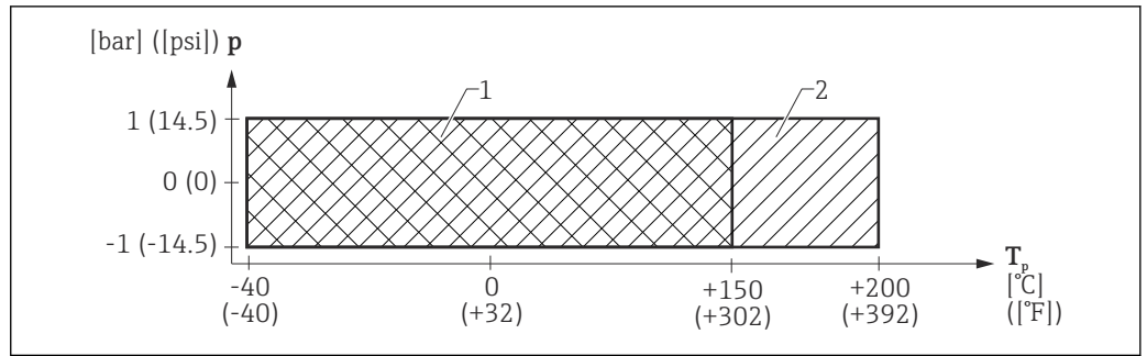
图 21 FMR67: 允许过程温度和过程压力范围, 带 PTFE 齐平安装天线, DN80; 可调节 UNI 法兰, 铝
