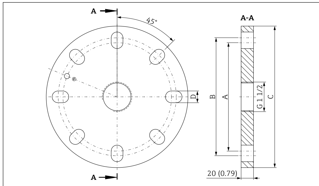
图 26 外形尺寸示意图：FMR67 的配套 UNI 法兰，不带空气吹扫接口。测量单位 mm (in)
