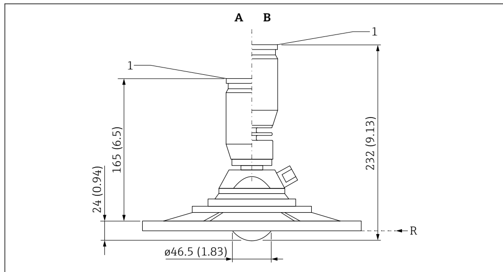
图 32 外形尺寸示意图: 天线, 带 UNI 法兰、天线角度调节装置和空气吹扫接口。测量单位 mm (in)
