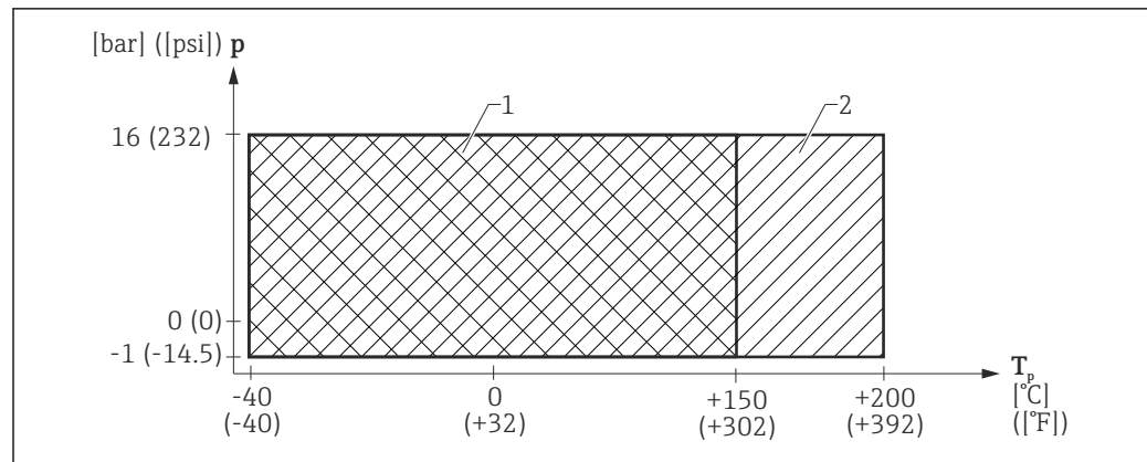
图 19 FMR67: 允许过程温度和过程压力范围, 带 PTFE 齐平安装天线, DN80; 标准法兰, 316L
