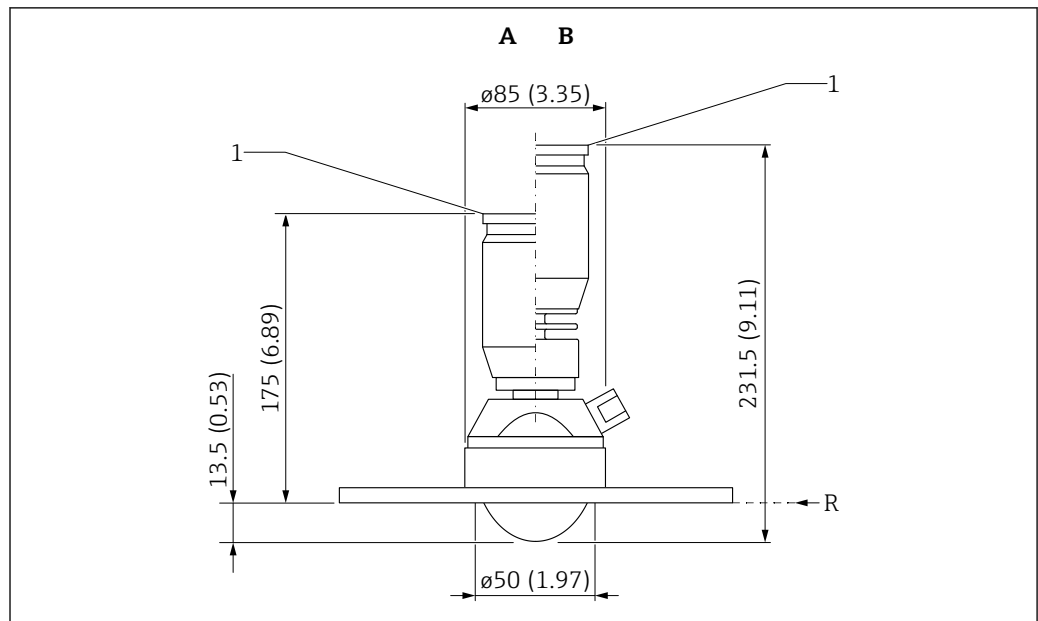
图 30 外形尺寸示意图: 天线, 带 UNI 法兰和空气吹扫接口。测量单位 mm (in)
