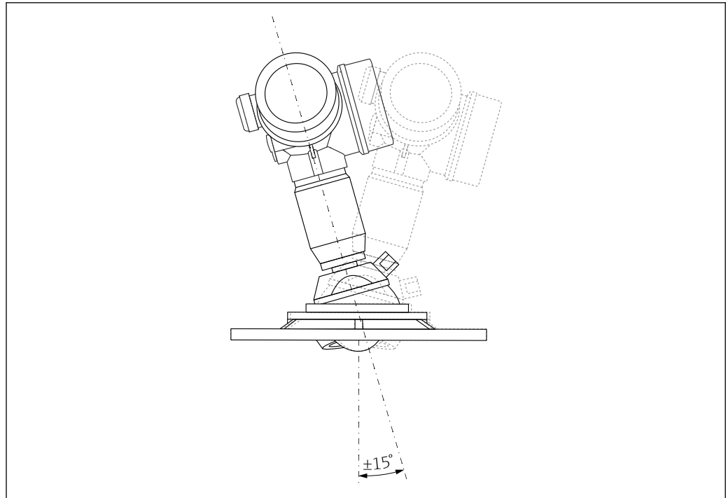
图 15 带天线角度调节装置的 Micropilot FMR67
