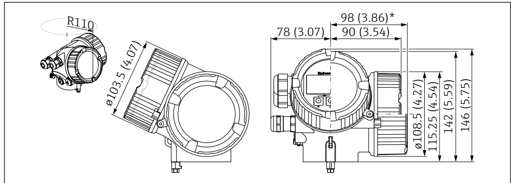
图 22 GT18 外壳 (316 L)。测量单位 mm (in)
