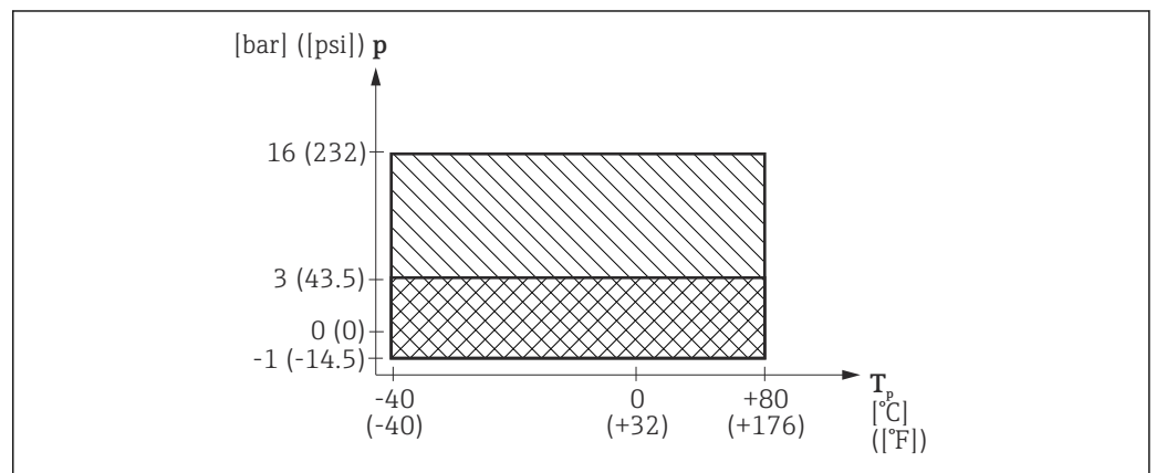
18 FMR67: 允许过程温度和过程压力范围，带 PTFE 水滴型天线，DN50
