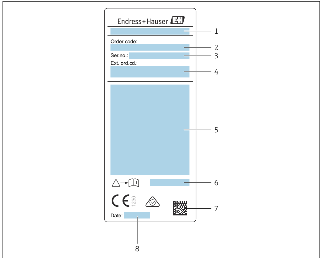
图 3 传感器的铭牌示意图
