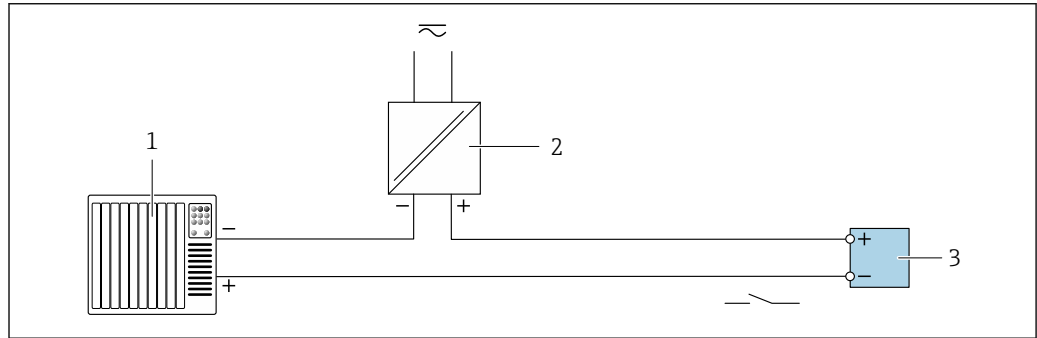
图 25 开关量输出(无源信号)的连接实例
