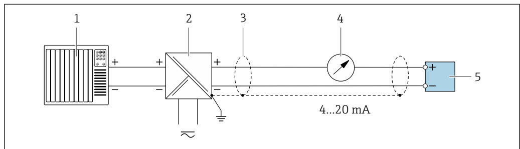
图 20 接线示例：4...20 mA HART 电流输出（无源信号）
