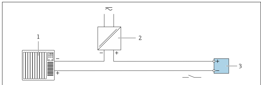
图 26 继电器输出的连接实例(无源)
