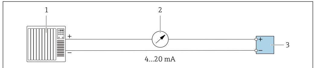
图 21 4...20 mA 有源电流输出的连接示例
