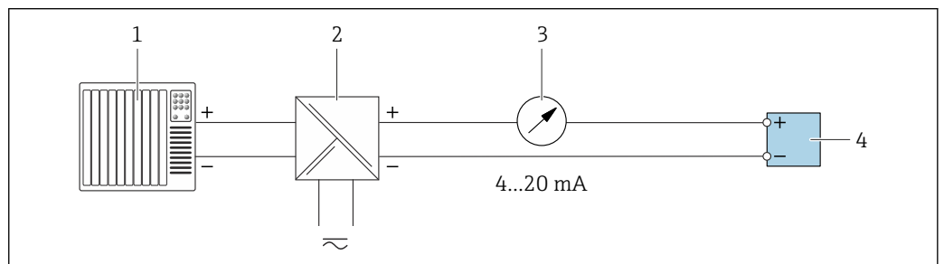
图 22 4...20 mA 电流输出（无源）的连接示例
