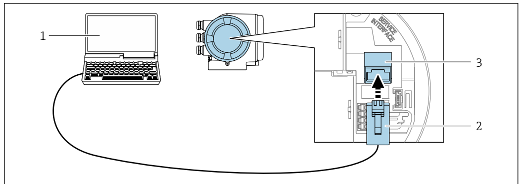
54 通过服务接口（CDI-RJ45）连接
