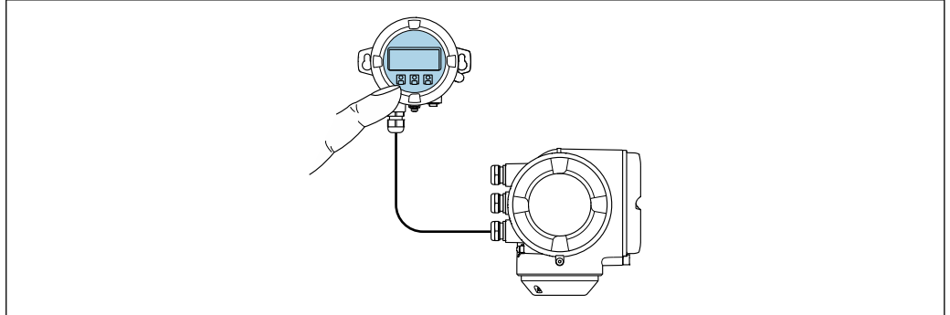
图 43 通过分离型显示与操作单元 DKX001 操作
