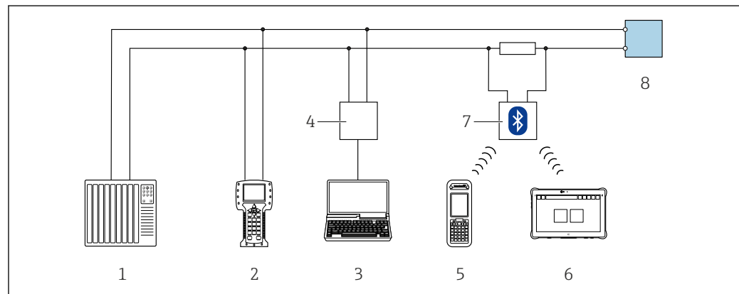
图 44 通过 HART 通信进行远程操作（有源信号）
