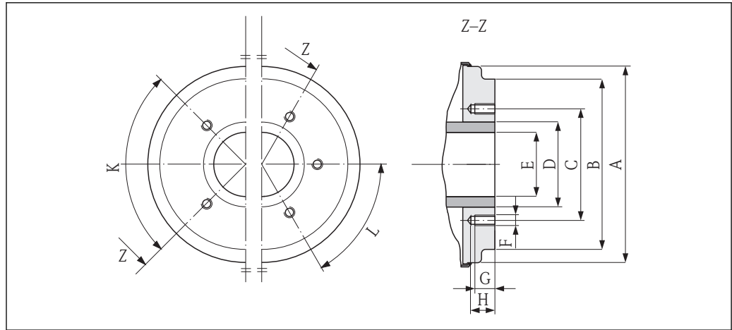
图 35 正视图，无过程连接
