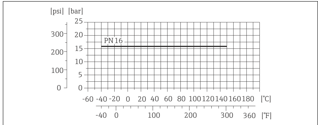
图 27 过程连接材料: 不锈钢 1.4404 (F316L)
