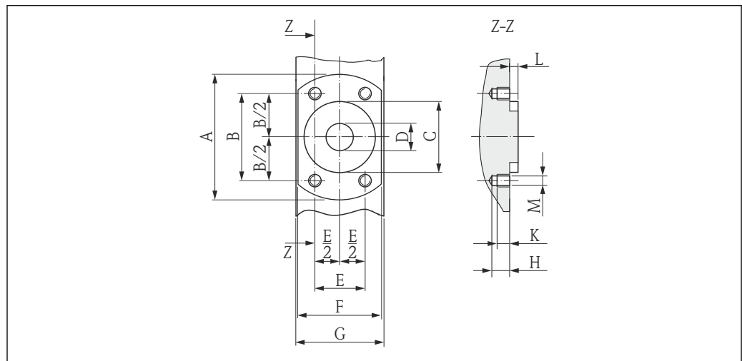
48 正视图, 无过程连接
