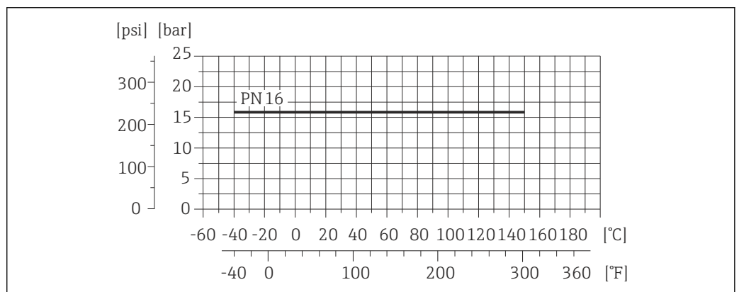
26 过程连接材料: 不锈钢 1.4404 (F316L)
