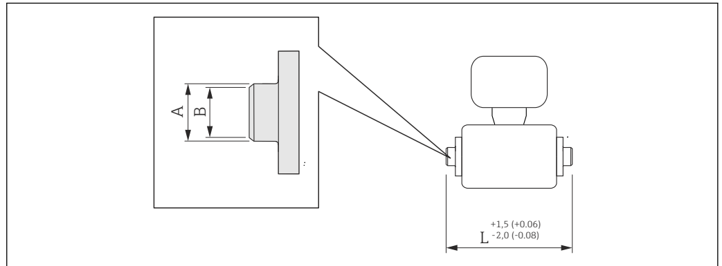
图 52 单位: mm (in)
