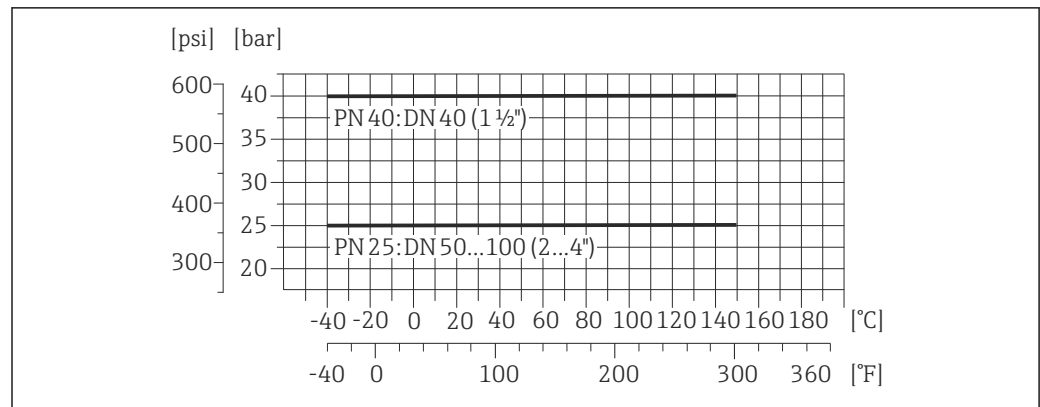
图 31 过程连接材料: 不锈钢 1.4404 (F316L)
