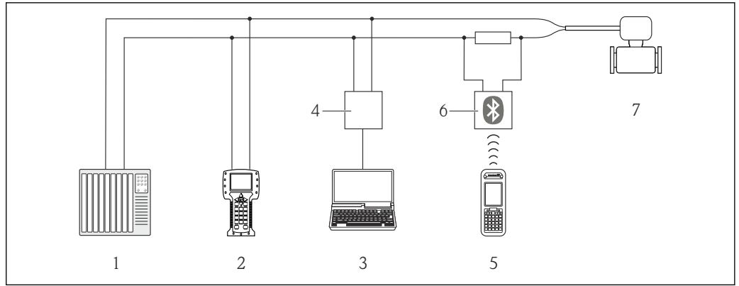
图 61 通过 HART 通信进行远程操作
