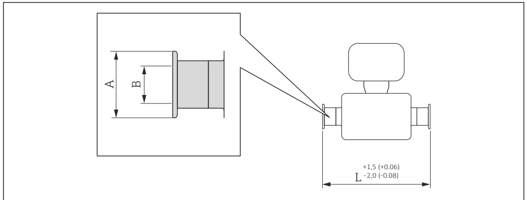
58 卫生型卡箍连接，适用于 ASME BPE 管道连接(缩径型)；单位：mm (in)
