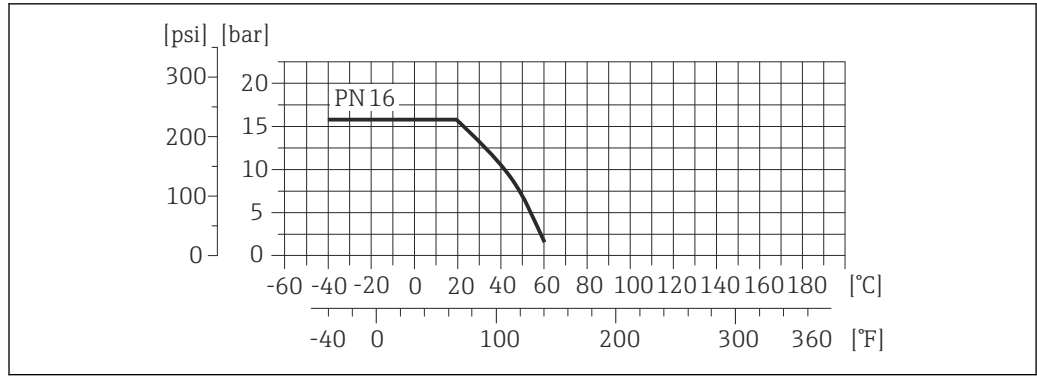
图 21 过程连接材料: PVC-U
