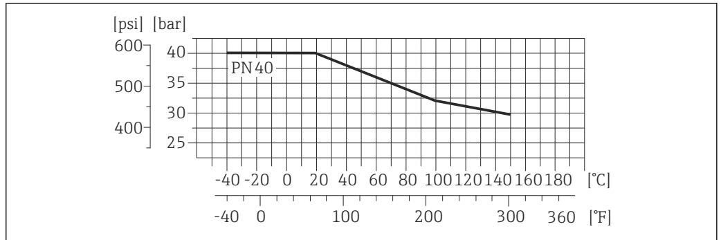
18 过程连接材料: 不锈钢 1.4404 (F316L)
