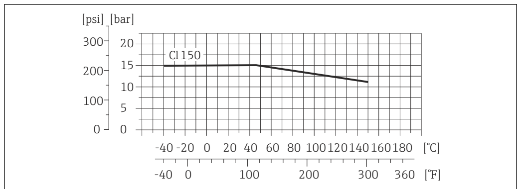
图 22 过程连接材料: 不锈钢 1.4404 (F316L)
