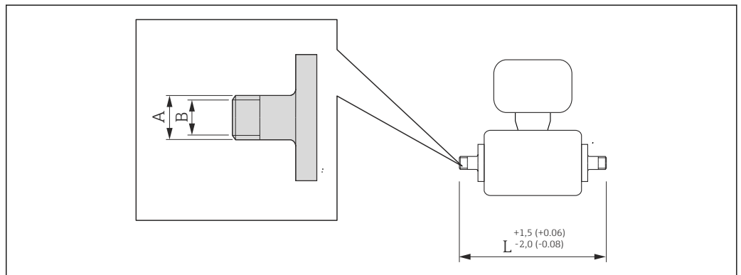
图 55 单位: mm (in)
