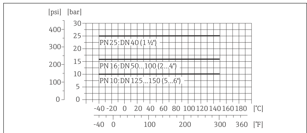
图 32 过程连接材料: 不锈钢 1.4404 (F316L)
