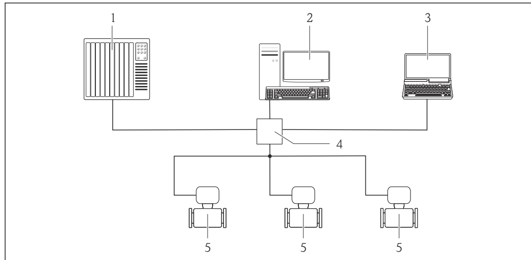
图 63 通过以太网现场总线进行远程操作
