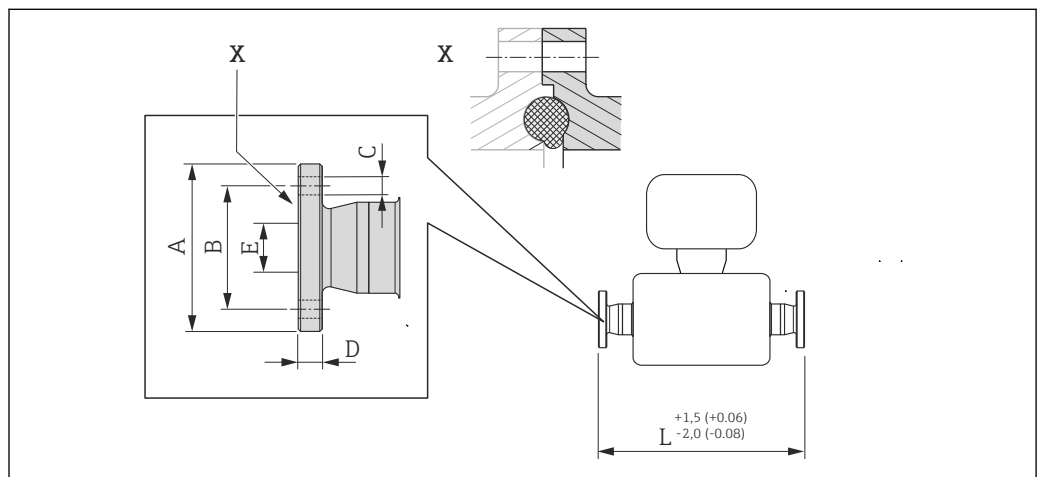
图 36 视图 X: 非对称型过程连接；灰色部分由供应商提供 单位: mm (in)
