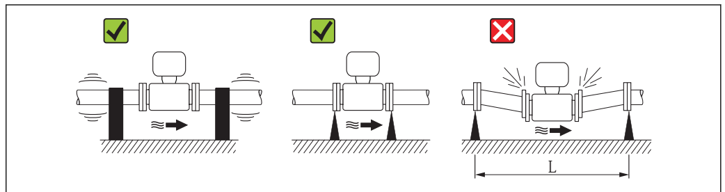
图 33 避免设备振动的措施(L > 10 m (33 ft))
