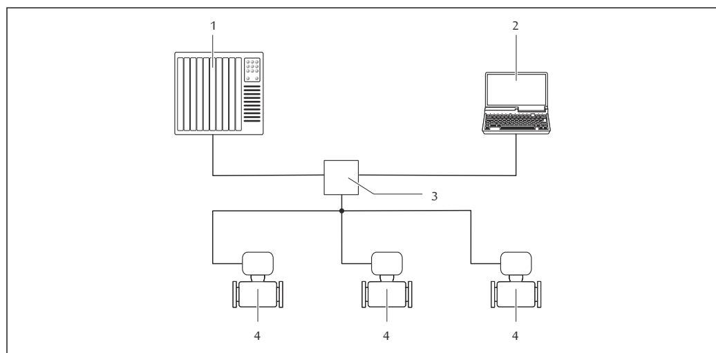
图 64 通过 PROFINET 网络进行远程操作
