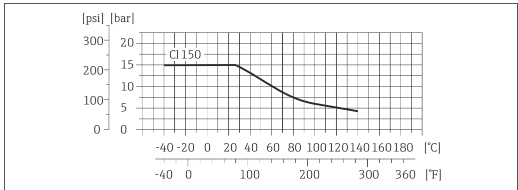
图 23 过程连接材料: PVDF
