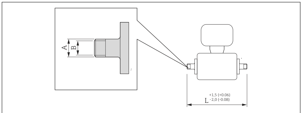
59 单位：mm (in)
