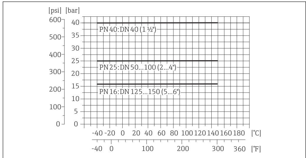
图 28 过程连接材料: 不锈钢 1.4404 (F316L)
