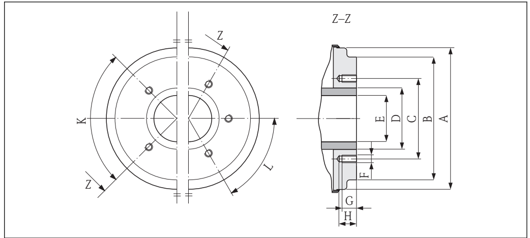
图 49 正视图，无过程连接
