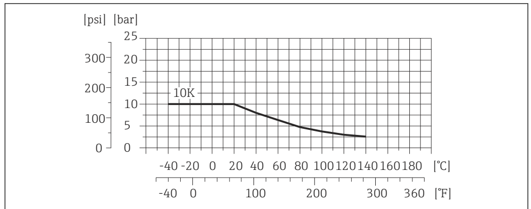
25 过程连接材料: PVDF
