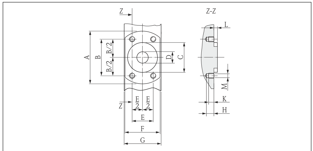
图 34 正视图，无过程连接
