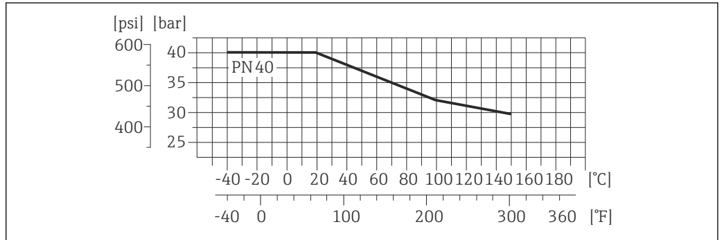
19 过程连接材料: 不锈钢 1.4404 (F316L)
