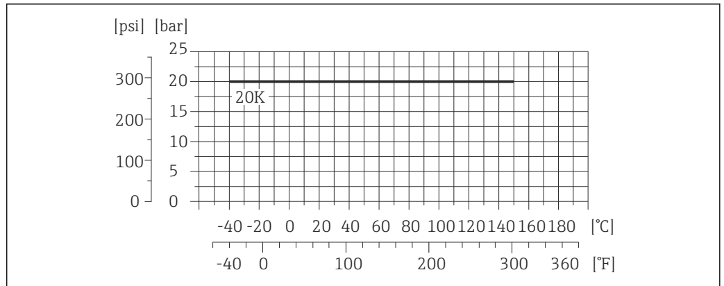
24 过程连接材料: 不锈钢 1.4404 (F316L)
