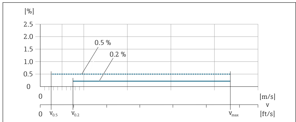
图 25 指定测量精度 (% o.r.)
