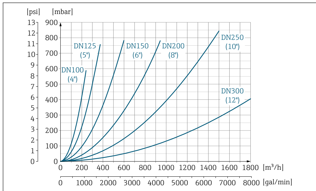
图 37 压损: 适用口径 DN 100...300 (4...12"); 订购选项“设计”, 选型代号 C “固定法兰, 无前后直管段”
