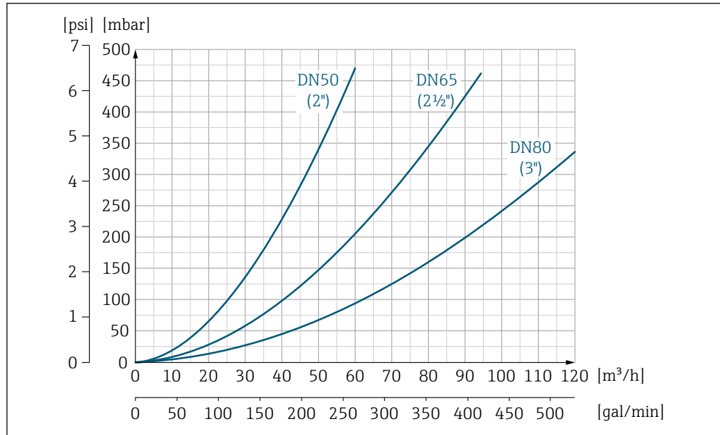
图 36 压损: 适用口径 DN 50...80 (2...3"); 订购选项“设计”, 选型代号 C “固定法兰, 无前后直管段”
