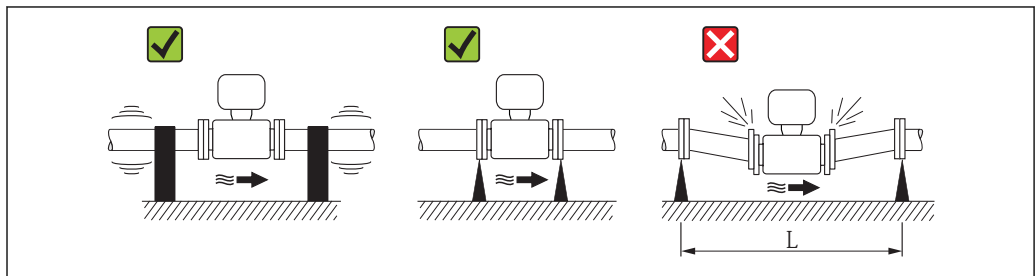
图 18 避免设备振动的措施( L > 10\text{ m} (33 ft))
