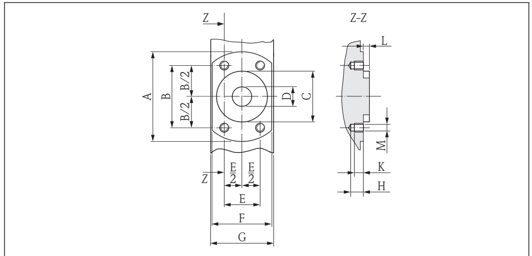
20 正视图, 无过程连接
