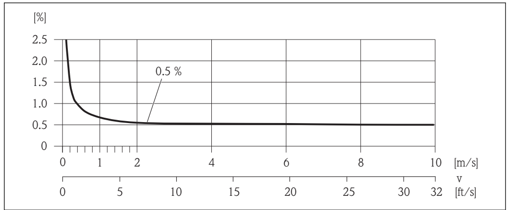
图 7 最大测量误差(% o.r.)
