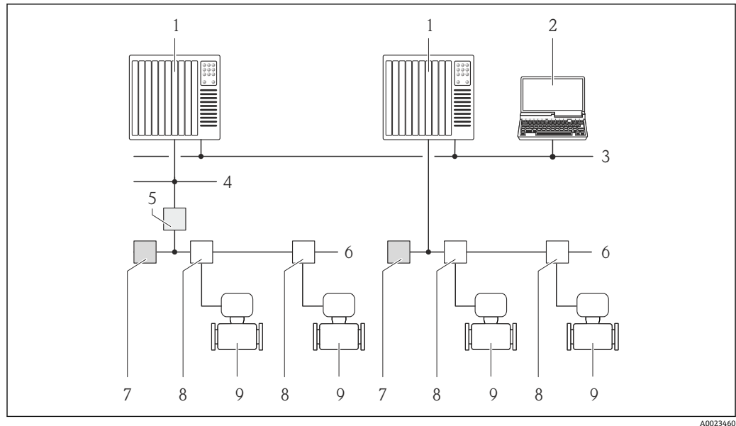
图 25 通过基金会现场总线(FF)网络进行远程操作
