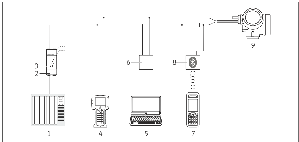
图 23 通过 HART 通信进行远程操作
