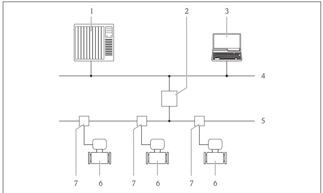
图 24 通过 PROFIBUS PA 网络进行远程操作
