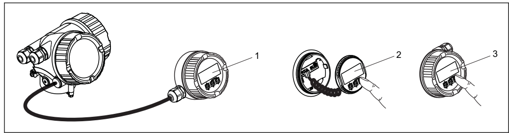
图 22 通过 FHX50 操作的操作选项
