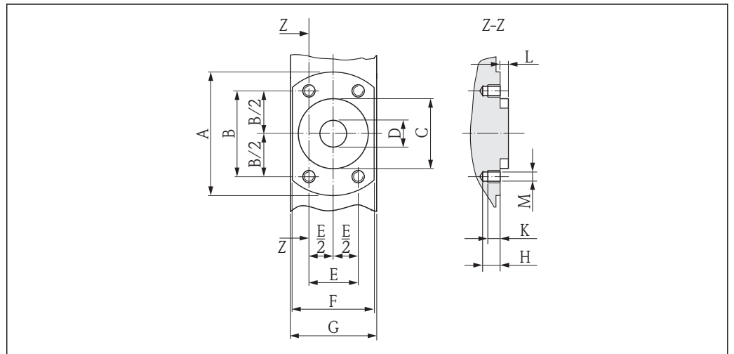
图 19 正视图, 无过程连接
