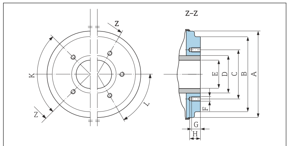
图 11 正视图, 未安装过程连接
