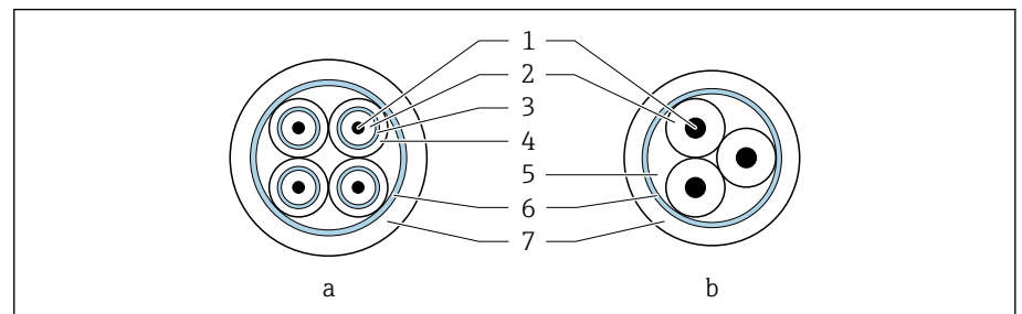
图 8 电缆截面图
