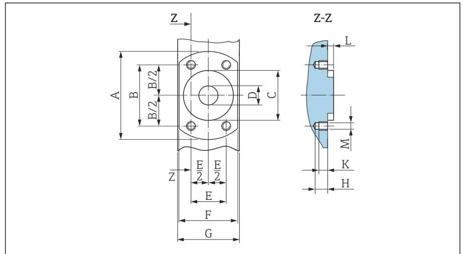
图 10 正视图, 未安装过程连接
