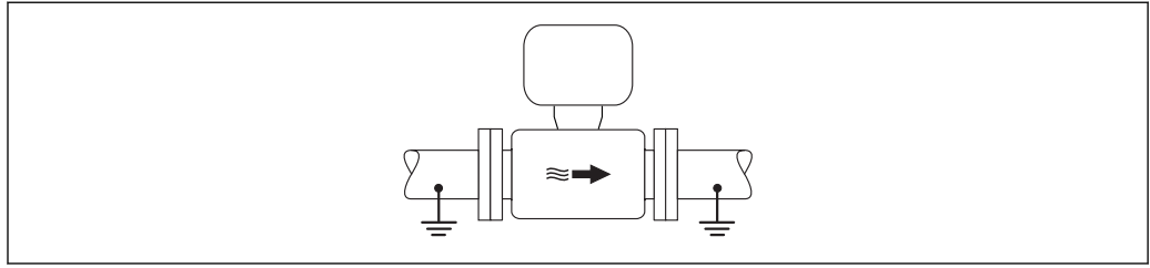
图 9 通过测量管实现电势平衡
