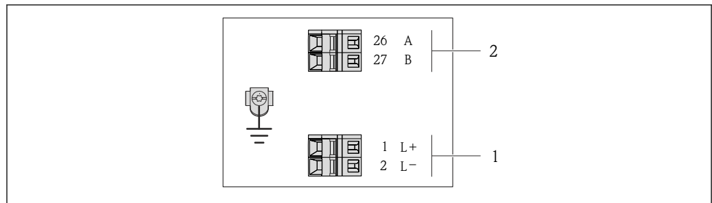
图 6 Modbus RS485 型仪表的接线端子分配示意图
