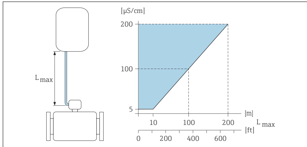
图 29 允许连接电缆长度
