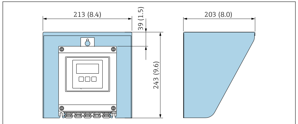
图 34 Proline 500 (数字) 的防护罩
