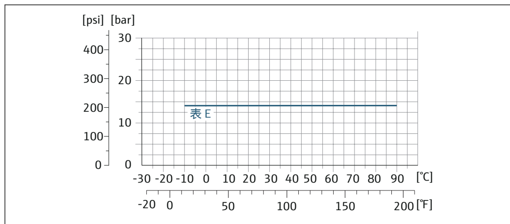
图 42 过程连接材质: 碳钢
