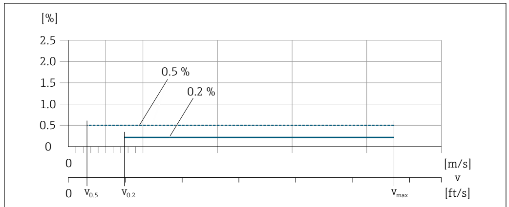
图 26 指定测量精度 (% o.r.)
