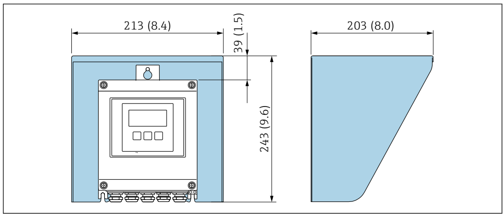
48 Proline 500 (数字) 的防护罩
