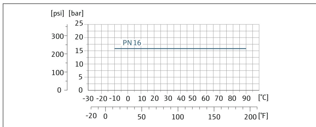
图 43 过程连接材质: 碳钢
