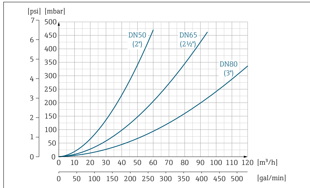
图 45 压损: 适用口径 DN 50...80 (2...3"); 订购选项“设计”, 选型代号 C “固定法兰, 无前后直管段”
