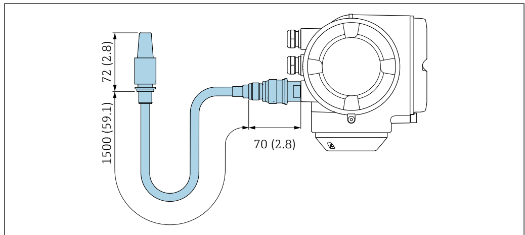
图 59 单位: mm (in)
