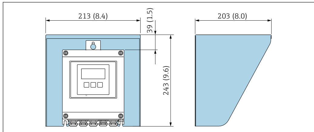
图 54 Proline 500 (数字) 的防护罩
