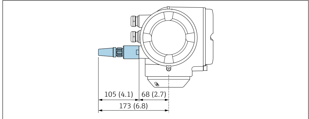
图 58 单位: mm (in)
