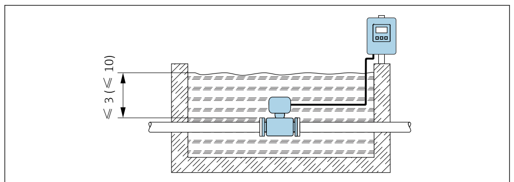
图 36 单位: m (ft)
