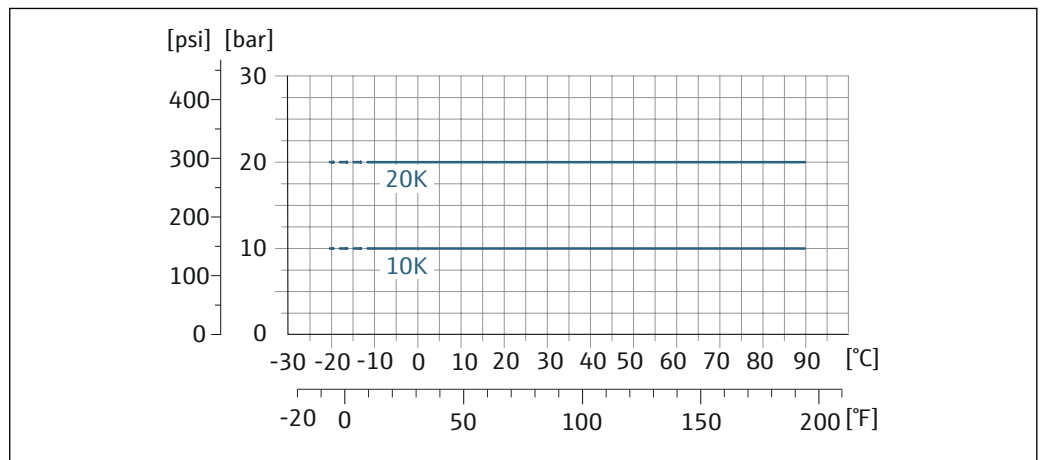
40 过程连接材质: 不锈钢 (-20 °C (-4 °F)) ; 碳钢 (-10 °C (14 °F))
