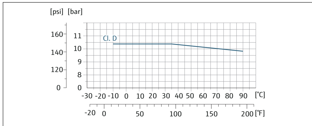
图 41 过程连接材质: 碳钢
