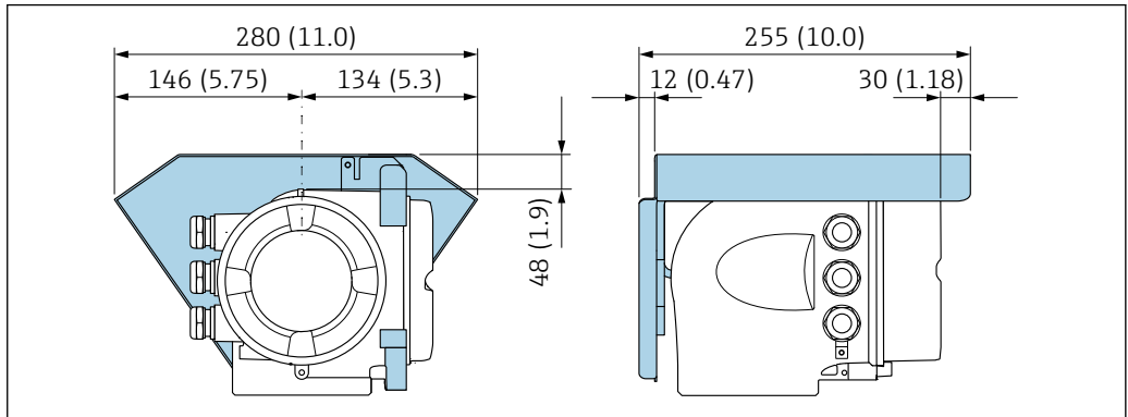
49 Proline 500 (模拟) 的防护罩
