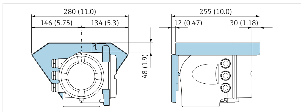
图 55 Proline 500 (模拟) 的防护罩
