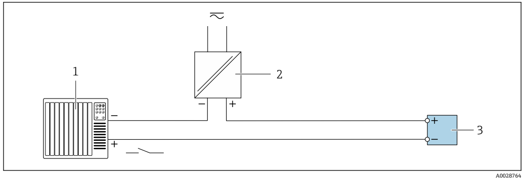
图 30 状态输入的连接示例
