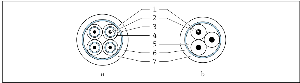
图 16 电缆截面
