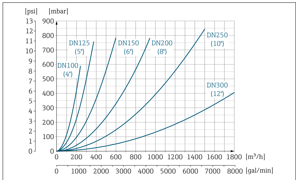
图 48 压损: 适用口径 DN 100...300 (4...12"); 订购选项“设计”, 选型代号 C “固定法兰, 无前后直管段”
