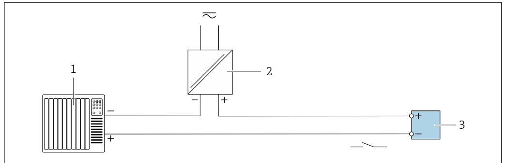
图 28 继电器输出的连接实例(无源)
