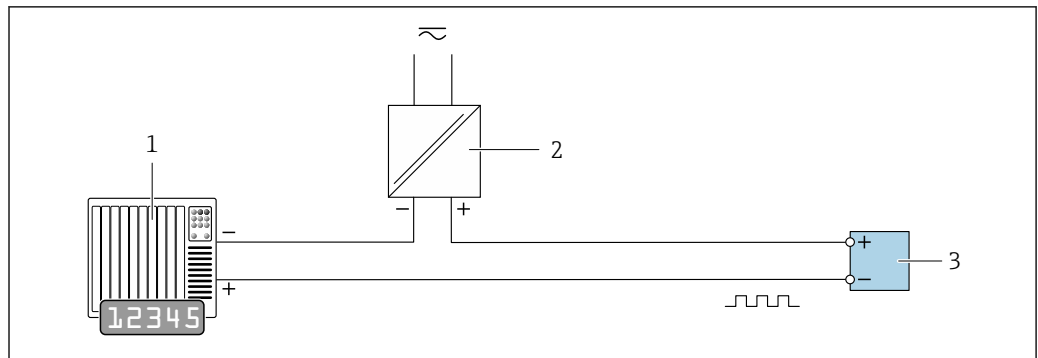
图 26 脉冲/频率输出（无源）的连接实例
