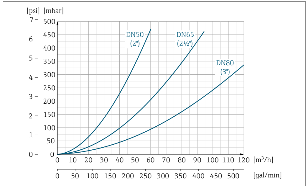
图 47 压损: 适用口径 DN 50...80 (2...3"); 订购选项“设计”, 选型代号 C “固定法兰, 无前后直管段”
