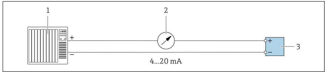
图 24 4...20 mA 有源电流输出的连接示例
