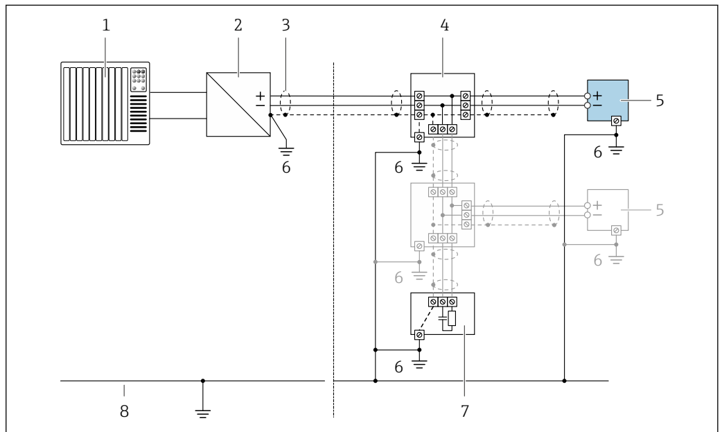
图 23 基金会现场总线(FF)的连接实例
