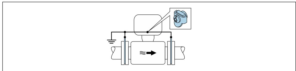
图 22 通过接地端子和接地环实现系统电势平衡
