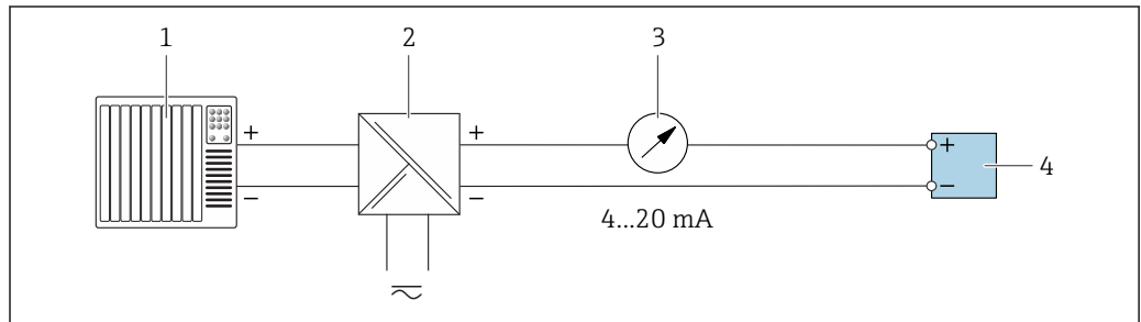
图 25 4...20 mA 电流输出（无源）的连接示例
