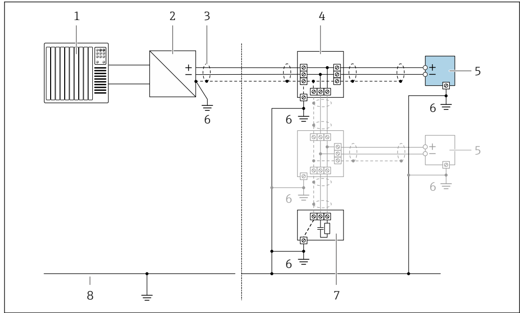
图 17 FOUNDATION Fieldbus 的接线实例
