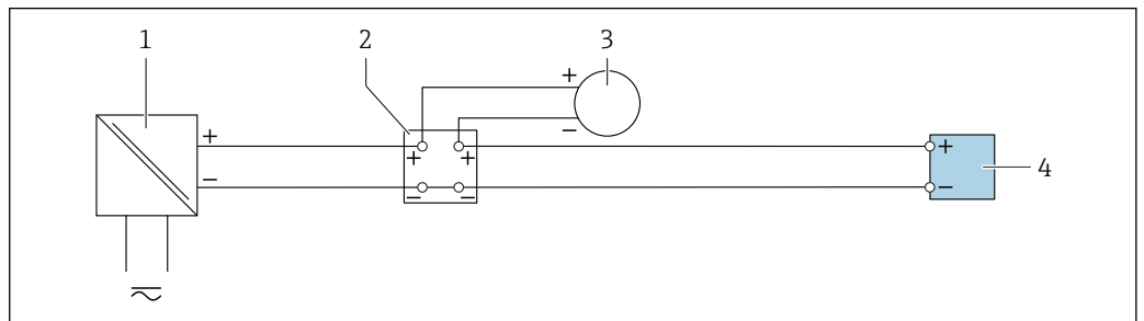
图 29 4...20 mA 电流输入的连接示例
