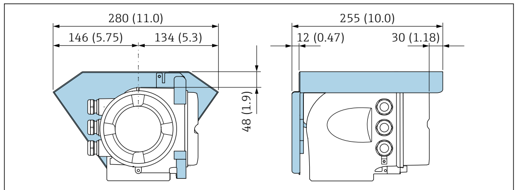
图 10 Proline 500 (模拟) 的防护罩
