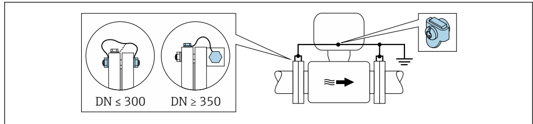
图 21 通过接地端子和管道法兰实现电势平衡
