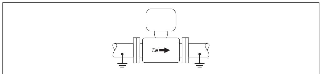
图 20 通过测量管实现电势平衡
