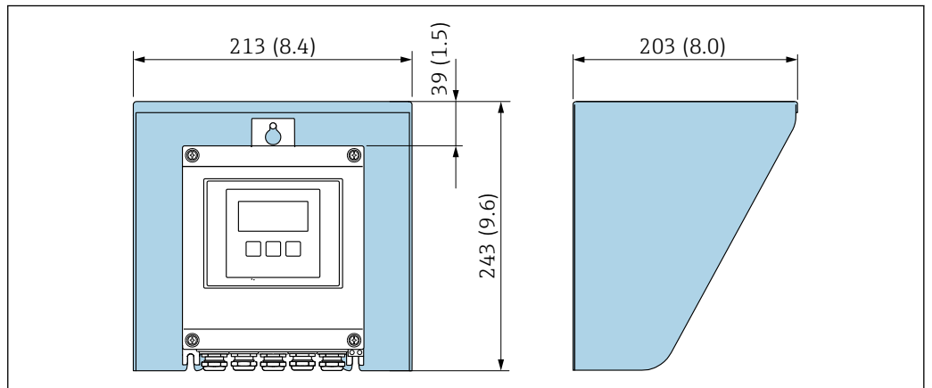
图 9 Proline 500 (数字) 的防护罩
