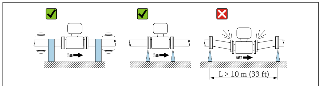
图 8 设备防振措施
