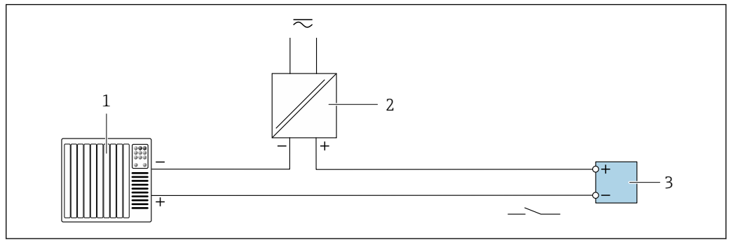
图 27 开关量输出(无源信号)的连接实例
