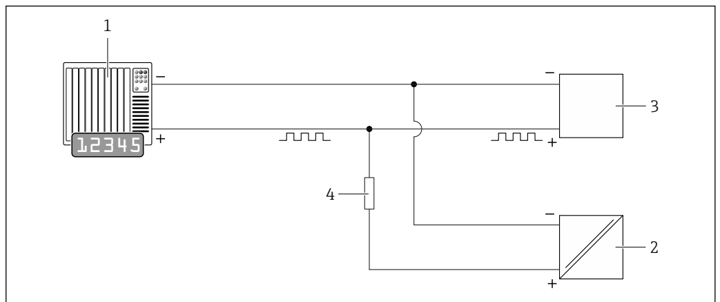
图 7 接线示例: 脉冲输出 (无源信号)
