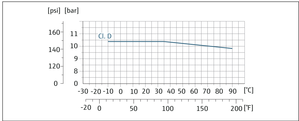
图 19 过程连接材质: 碳钢
