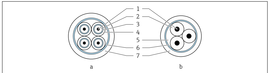
图 9 电缆截面图
