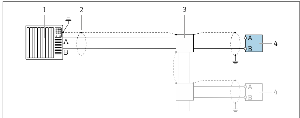
图 8 接线实例：Modbus RS485，非危险区
