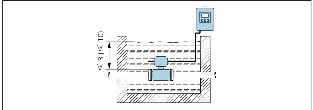
图 14 长期水下测量的仪表安装示意图
