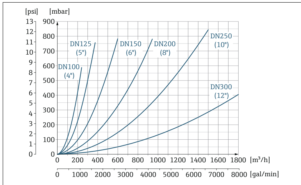
图 24 压损: 适用口径 DN 100...300 (4...12"); 订购选项“设计”, 选型代号 C “固定法兰, 缩径测量管, 无前后直管段长度要求”
