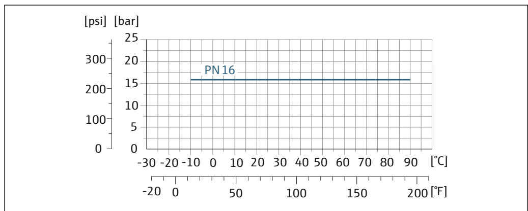
图 21 过程连接材质: 碳钢
