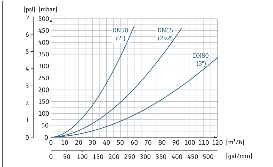
图 23 压损: 适用口径 DN 50...80 (2...3"); 订购选项“设计”, 选型代号 C “固定法兰, 缩径测量管, 无前后直管段长度要求”
