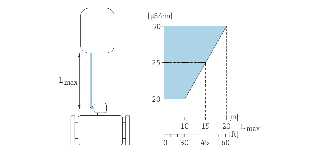
11 允许连接电缆长度
