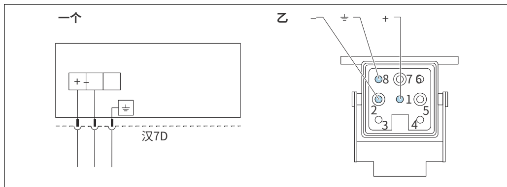
一个 带有 Harting 插头 Han7D 的设备的电气连接 设备上的插入
