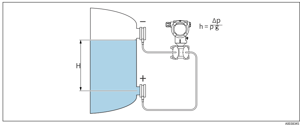
带毛细管的两侧隔膜密封
